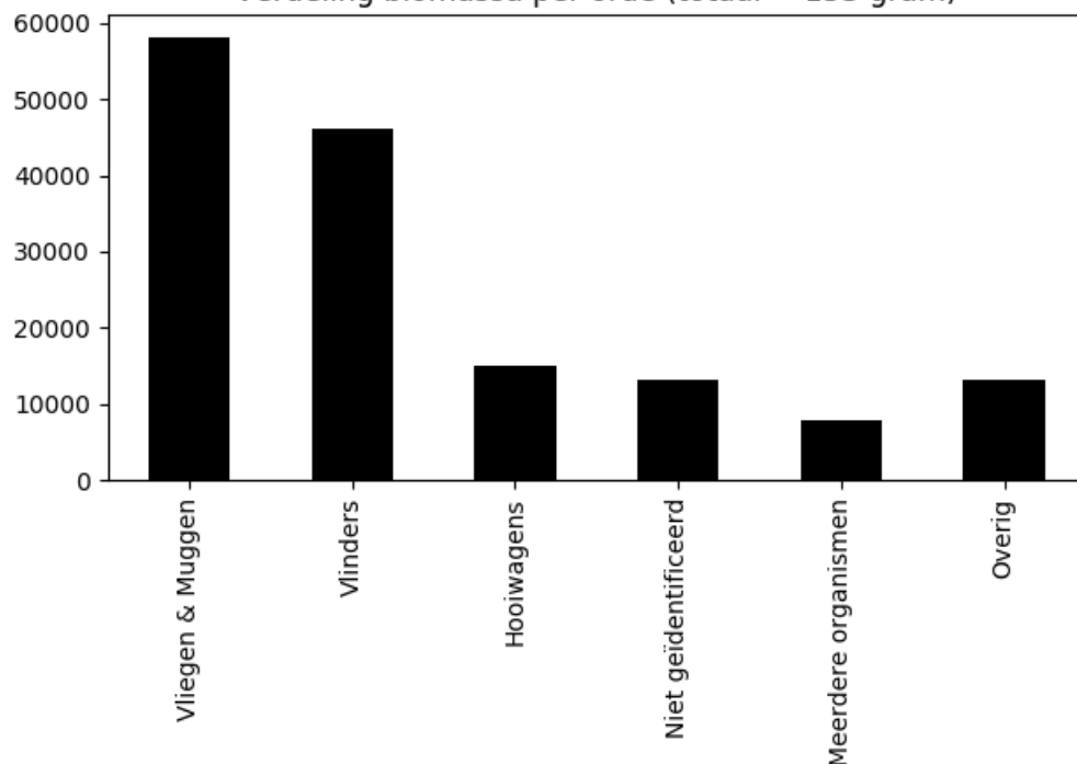
Verdeling biomassa per orde (totaal = 153 gram)
