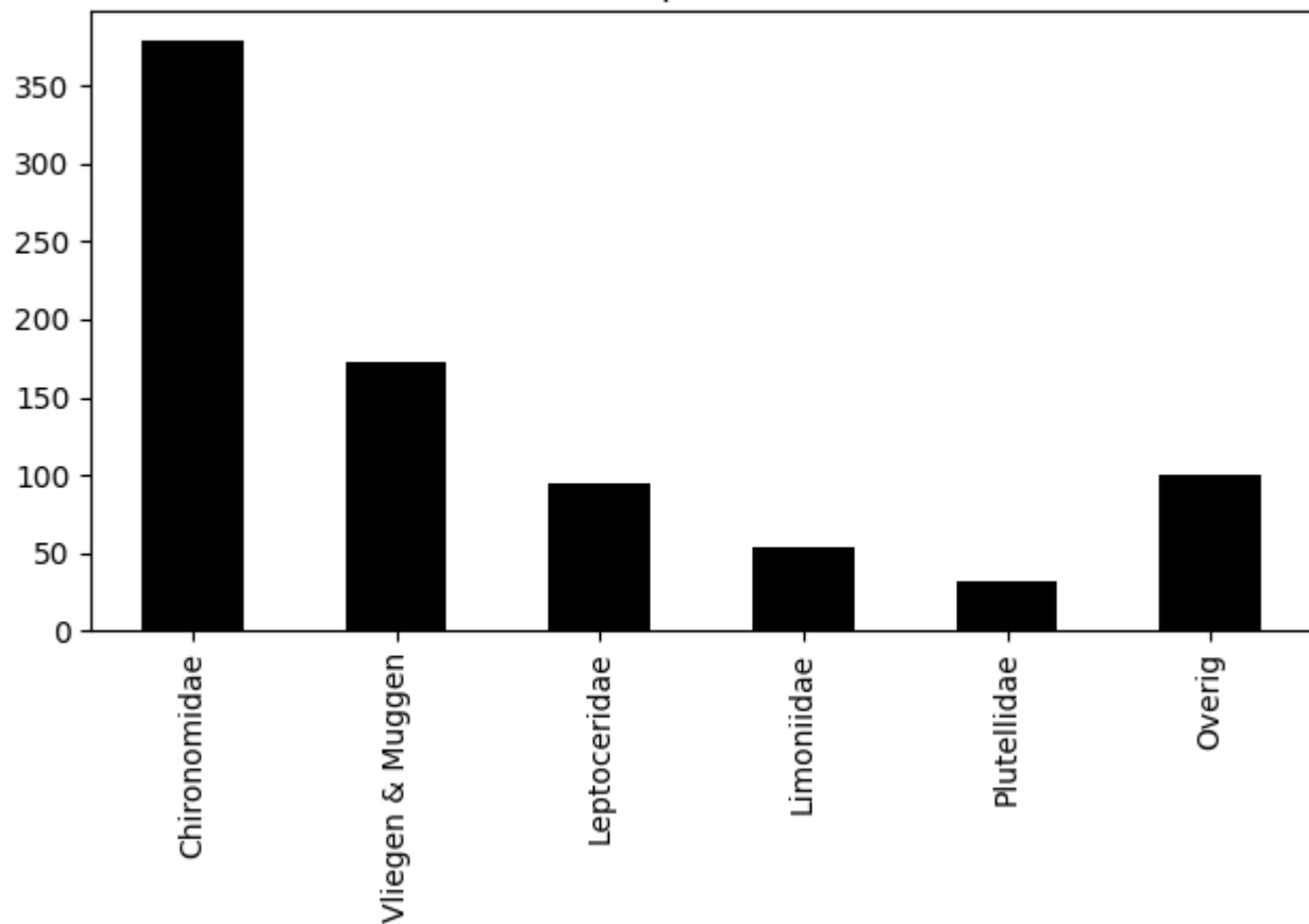
Voorkomen van ordes op 2020-07-29 (totaal = 831)
