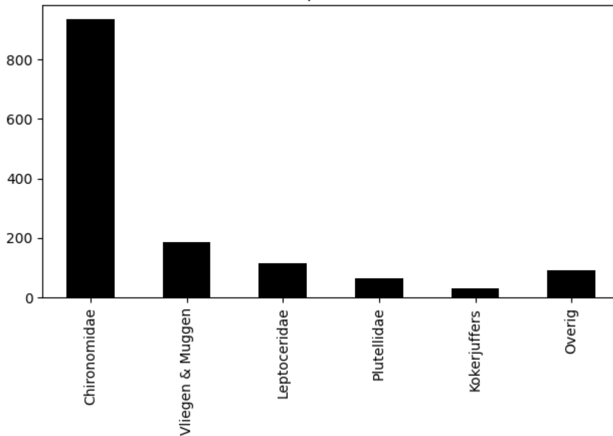
Voorkomen van ordes op 2020-07-28 (totaal = 1425)
