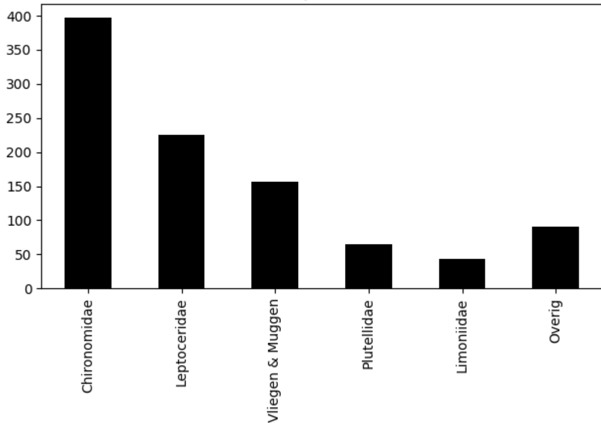
Voorkomen van ordes op 2020-07-23 (totaal = 978)
