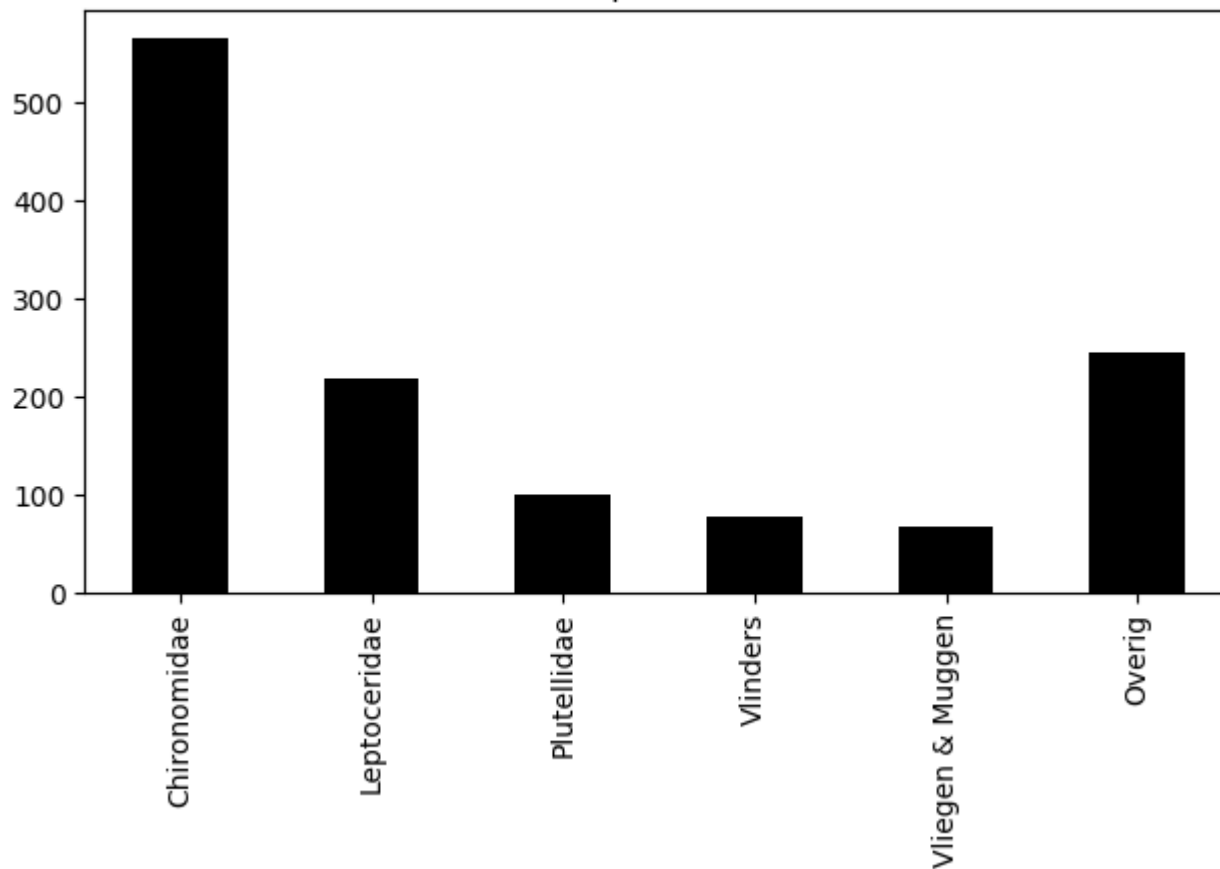
Voorkomen van ordes op 2020-07-31 (totaal = 1273)
