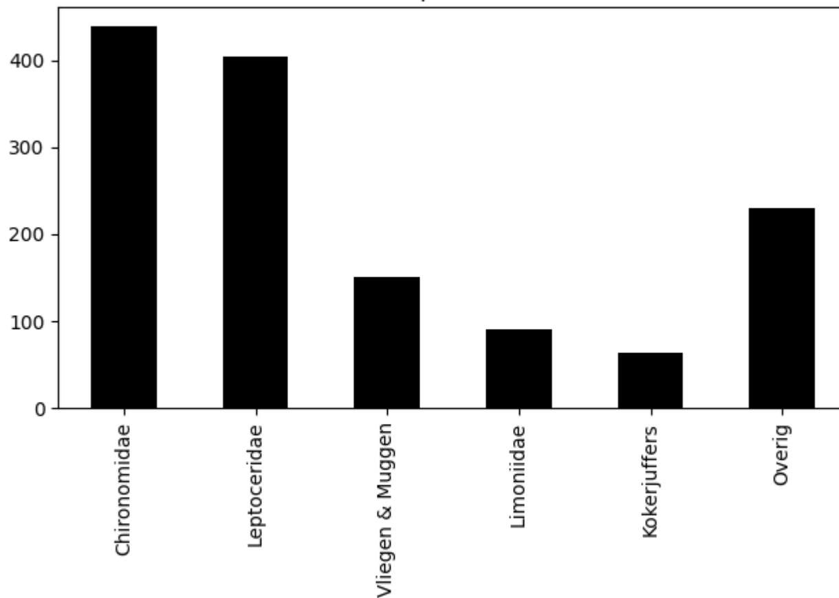
Voorkomen van ordes op 2020-07-25 (totaal = 1380)
