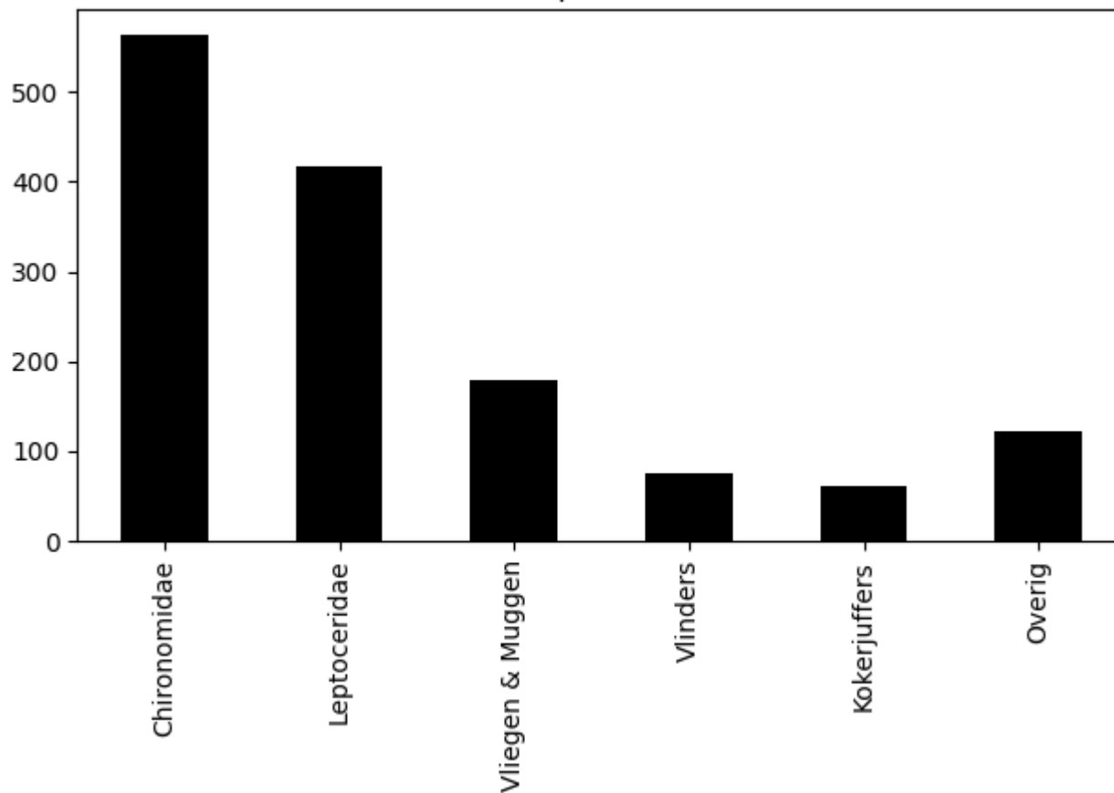
Voorkomen van ordes op 2020-07-26 (totaal = 1420)
