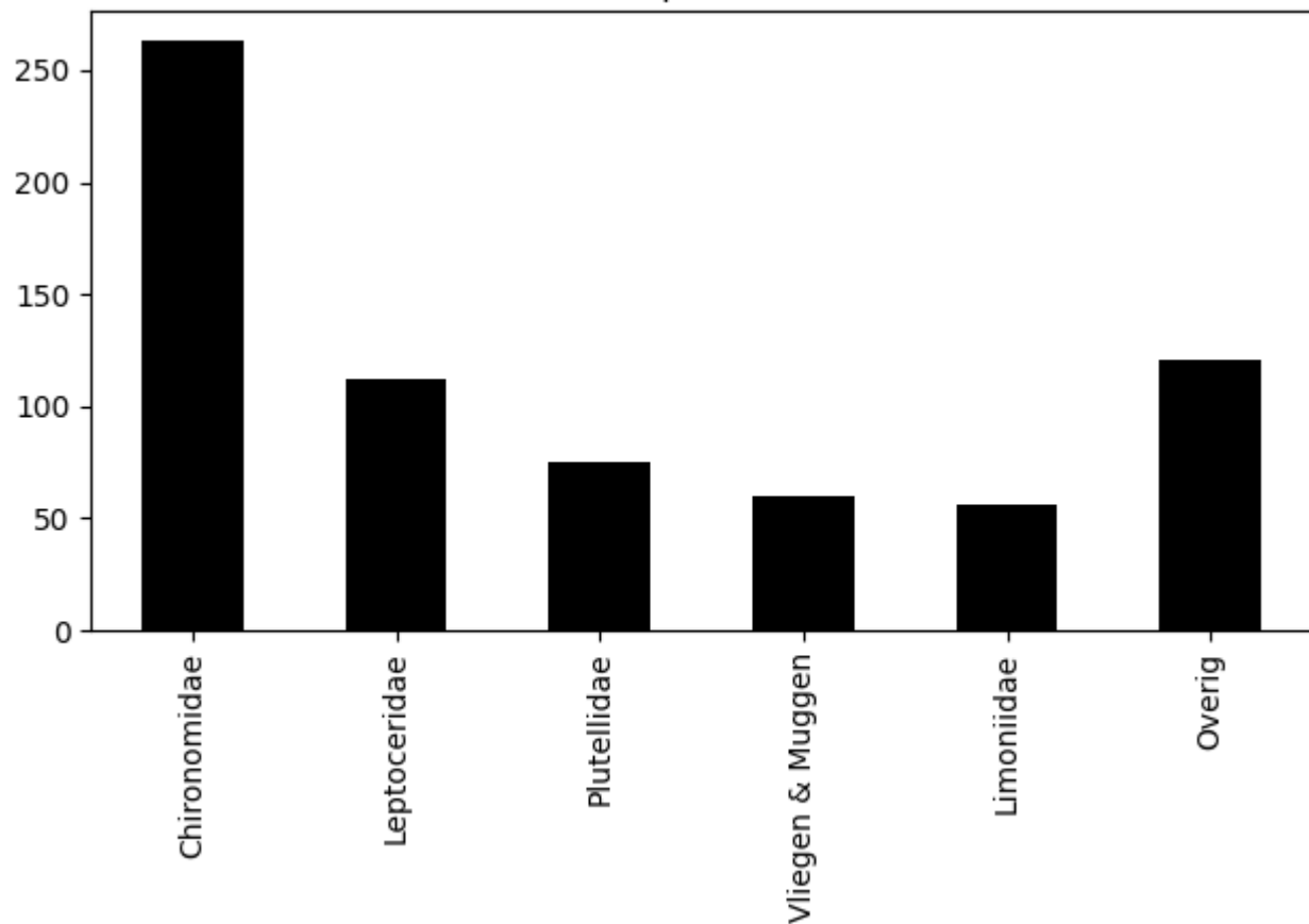
Voorkomen van ordes op 2020-07-30 (totaal = 687)
