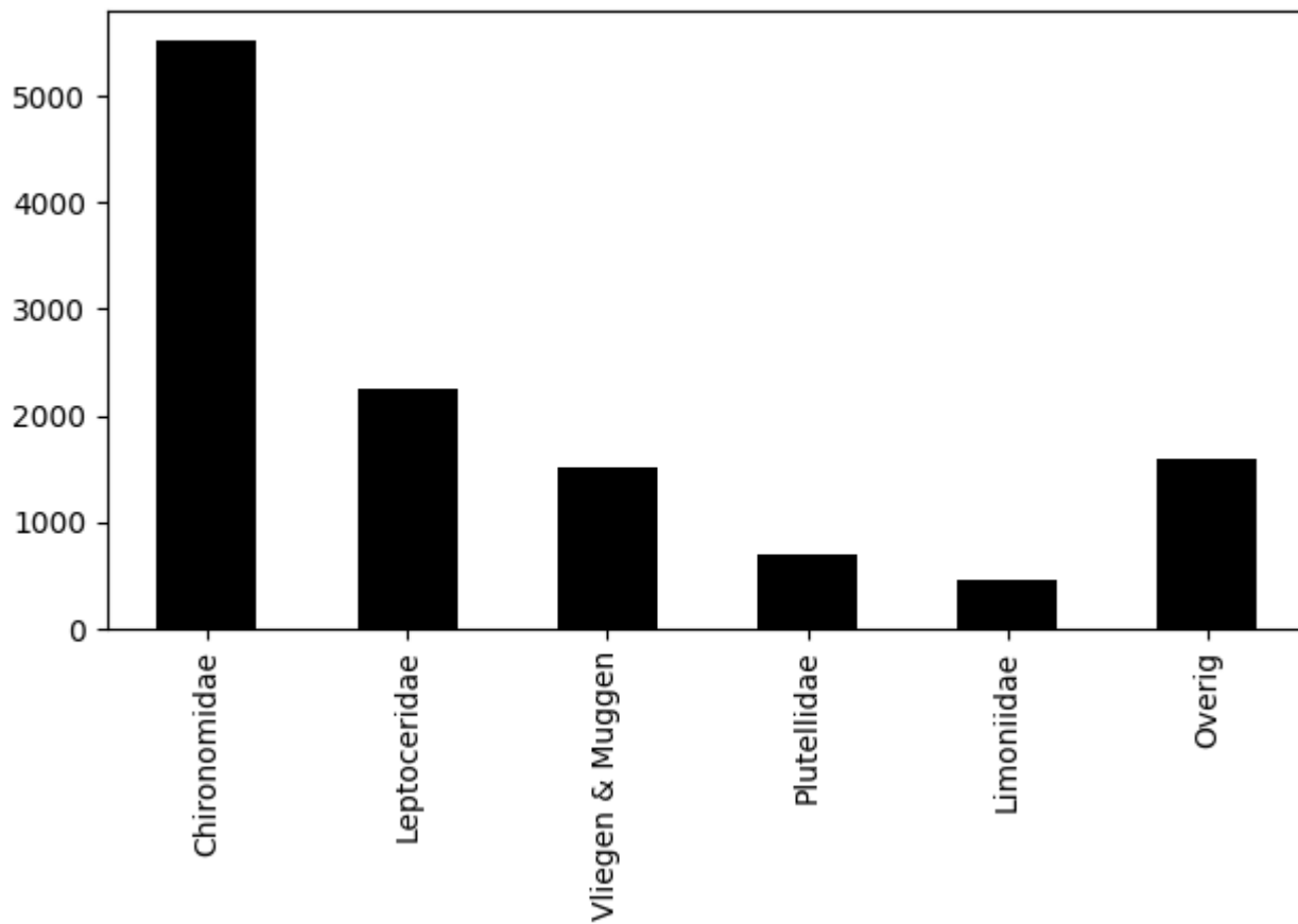
Voorkomen van ordes (totaal = 12047)
