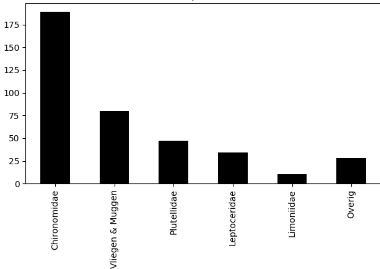
Voorkomen van ordes op 2020-07-21 (totaal = 388)
