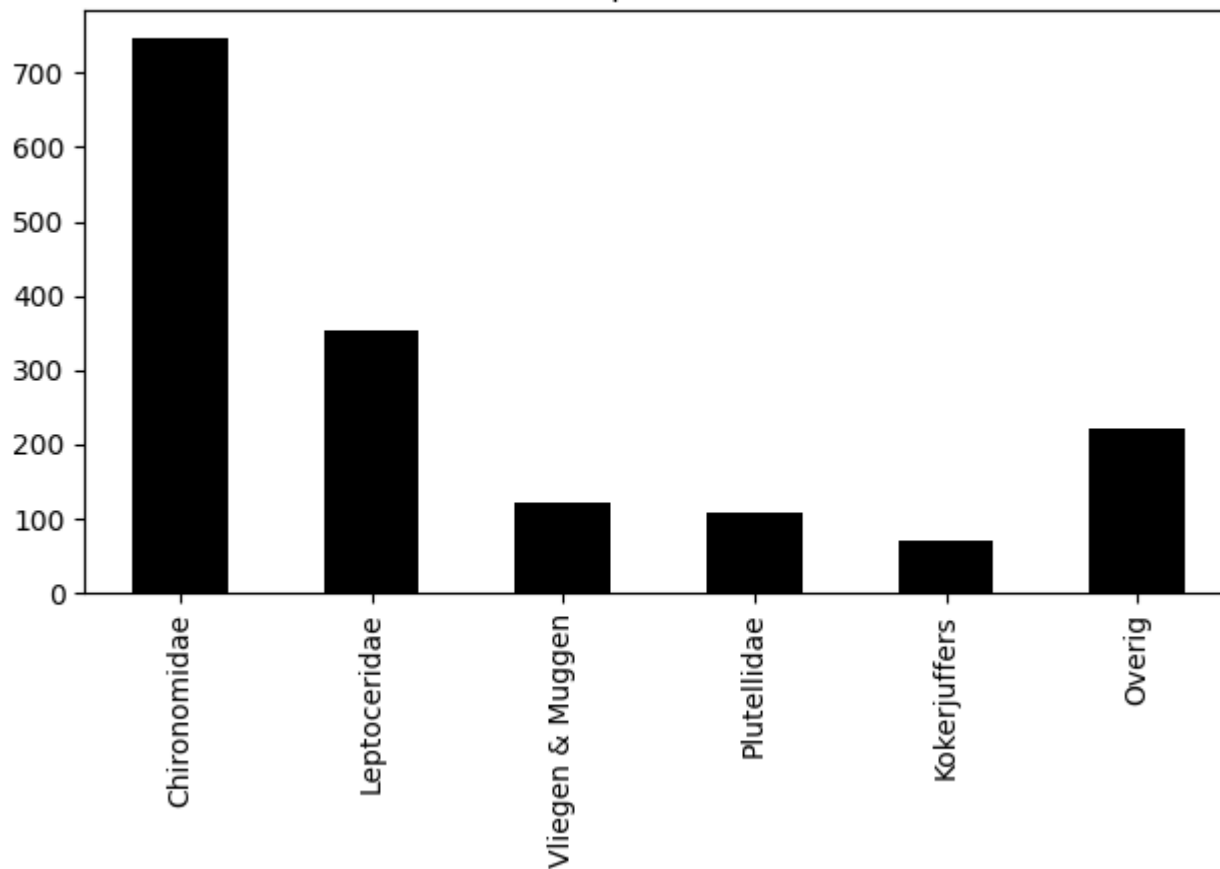
Voorkomen van ordes op 2020-07-24 (totaal = 1621)
