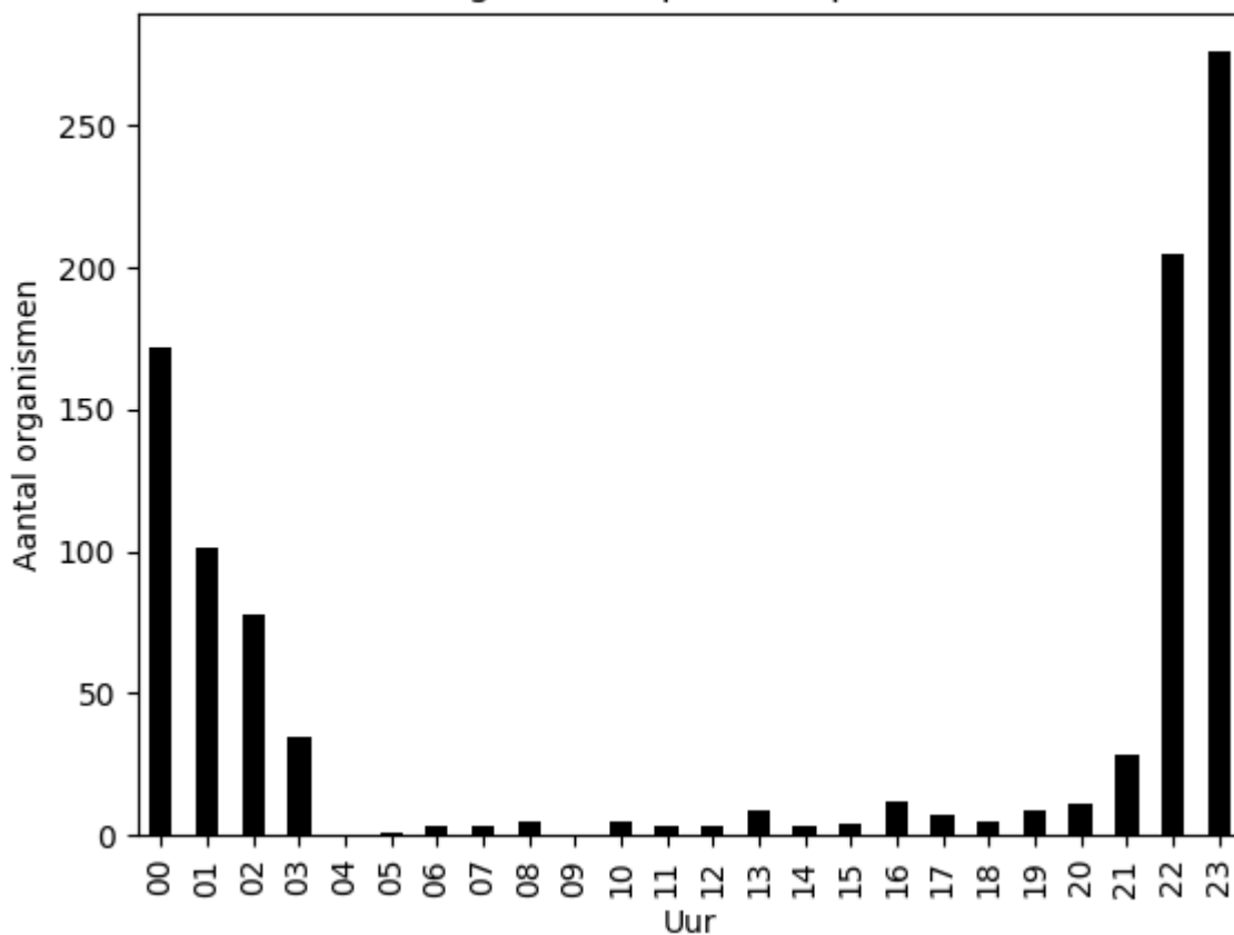
Aantal organismen per uur op 2020-07-23
