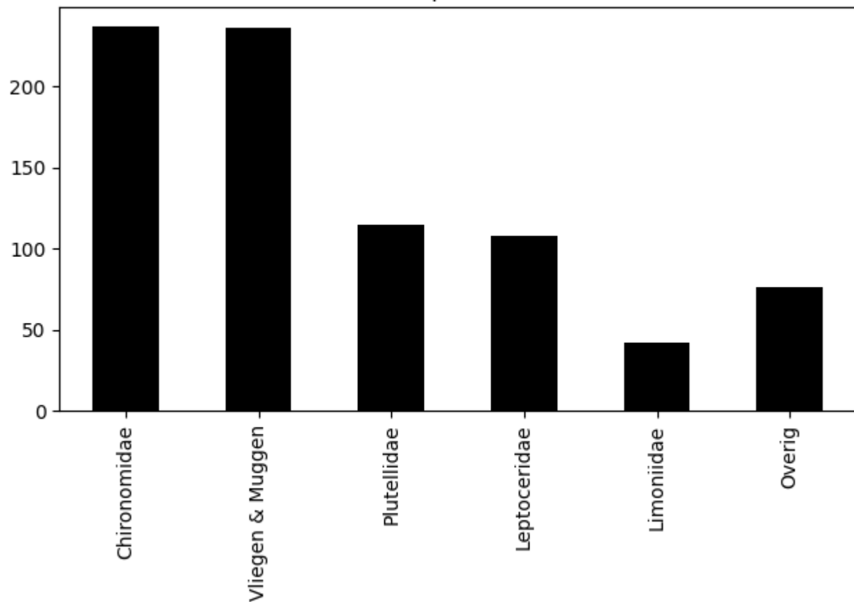
Voorkomen van ordes op 2020-07-22 (totaal = 814)
