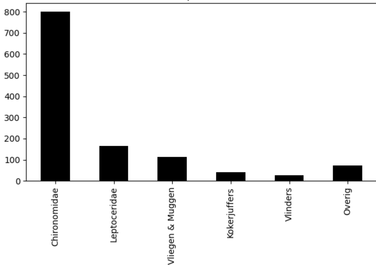
Voorkomen van ordes op 2020-07-27 (totaal = 1218)
