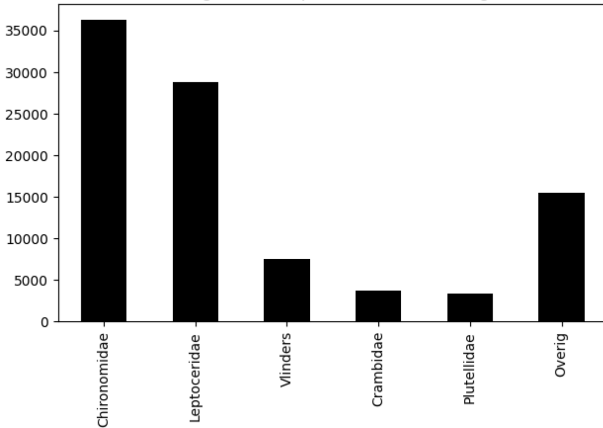
Verdeling biomassa per orde (totaal = 95 gram)
