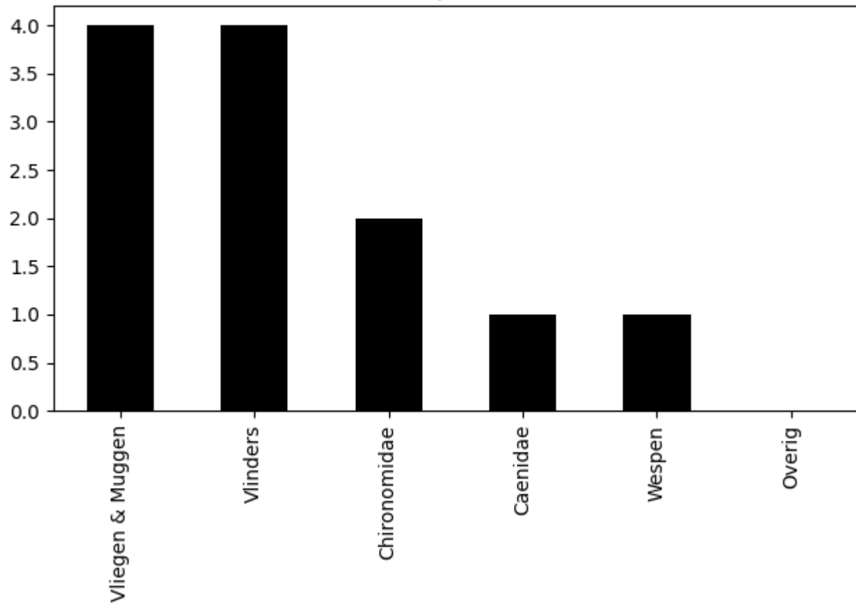
Voorkomen van ordes op 2020-08-01 (totaal = 12)
