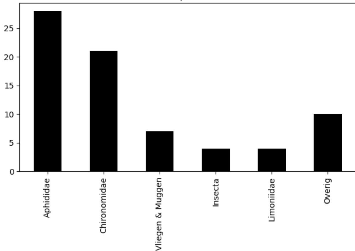
Voorkomen van ordes op 2020-07-25 (totaal = 74)
