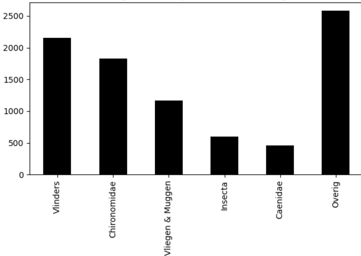
Verdeling biomassa per orde (totaal = 9 gram)
