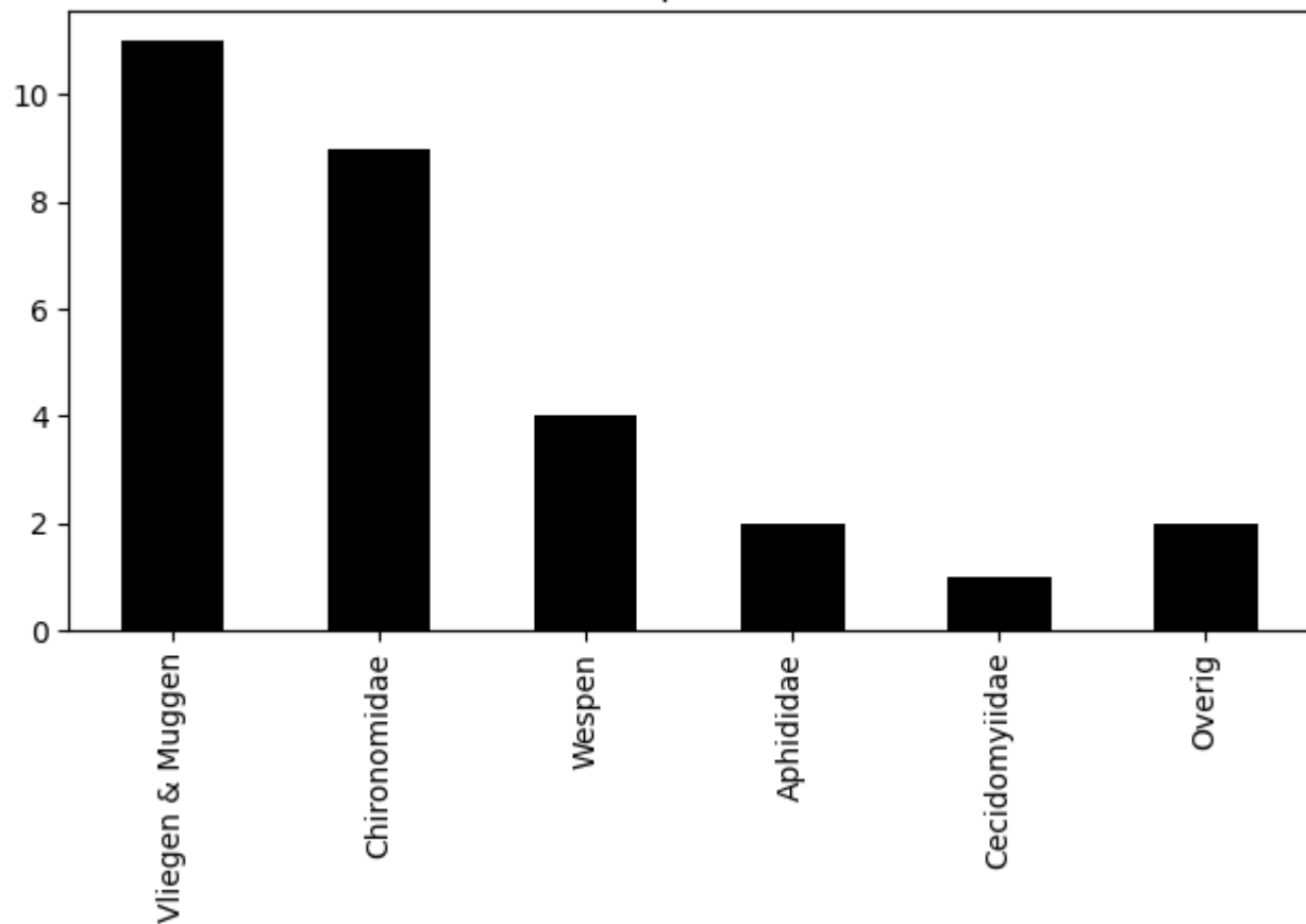
Voorkomen van ordes op 2020-07-27 (totaal = 29)
