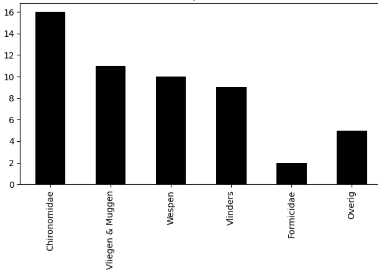
Voorkomen van ordes op 2020-08-07 (totaal = 53)
