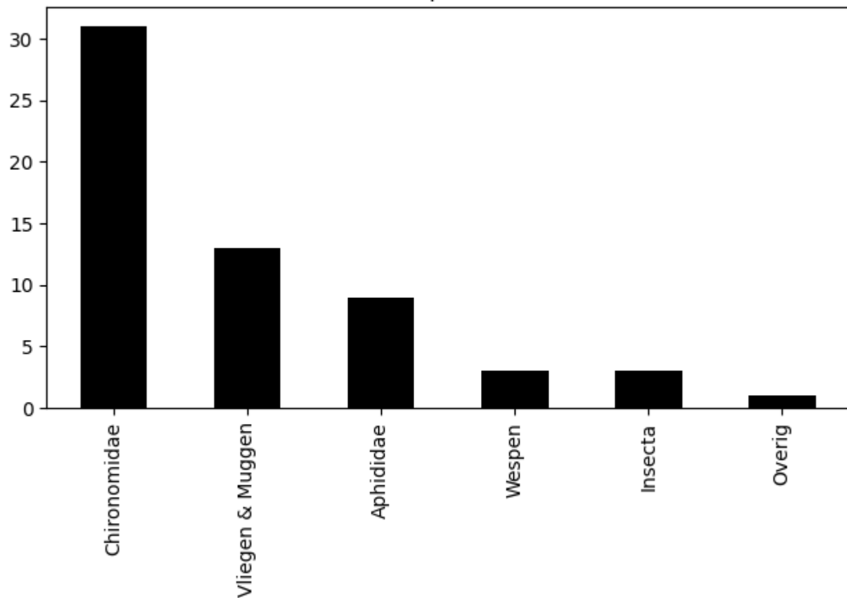
Voorkomen van ordes op 2020-07-24 (totaal = 60)
