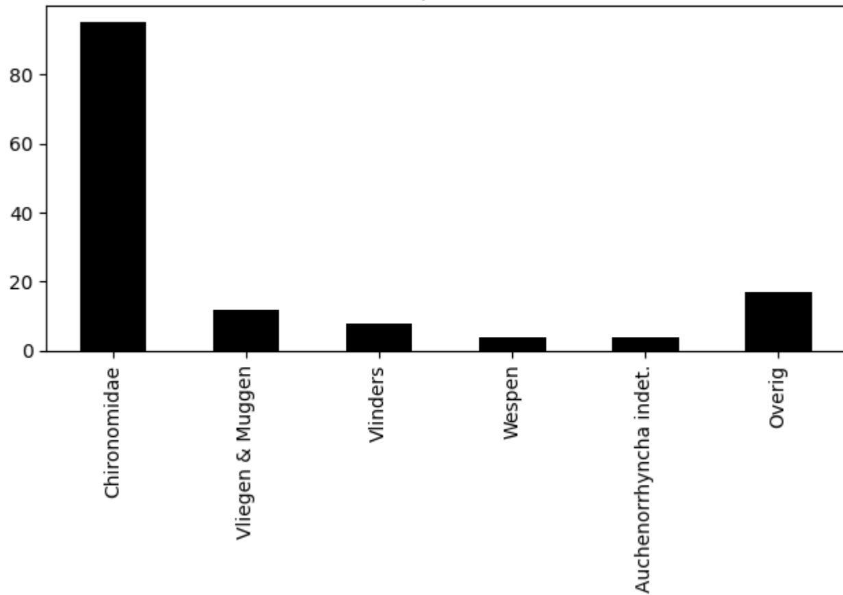
Voorkomen van ordes op 2020-08-12 (totaal = 140)
