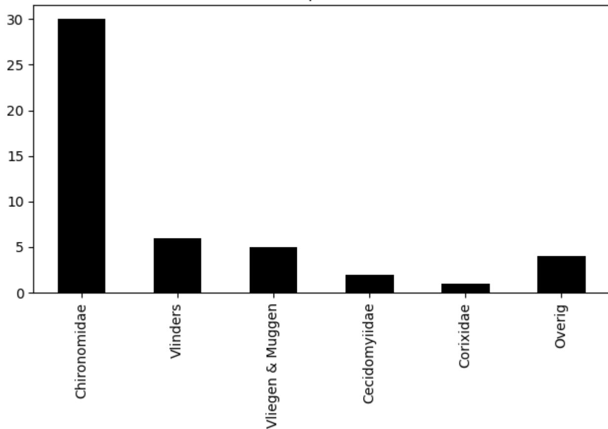
Voorkomen van ordes op 2020-08-16 (totaal = 48)
