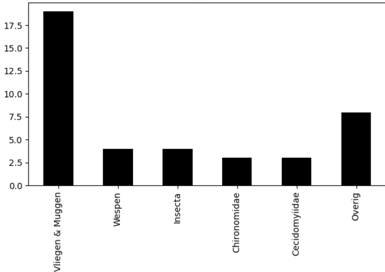
Voorkomen van ordes op 2020-08-04 (totaal = 41)
