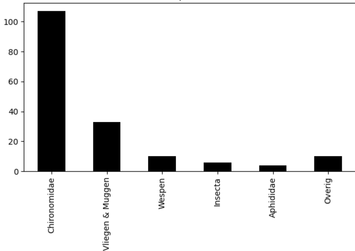
Voorkomen van ordes op 2020-08-01 (totaal = 170)
