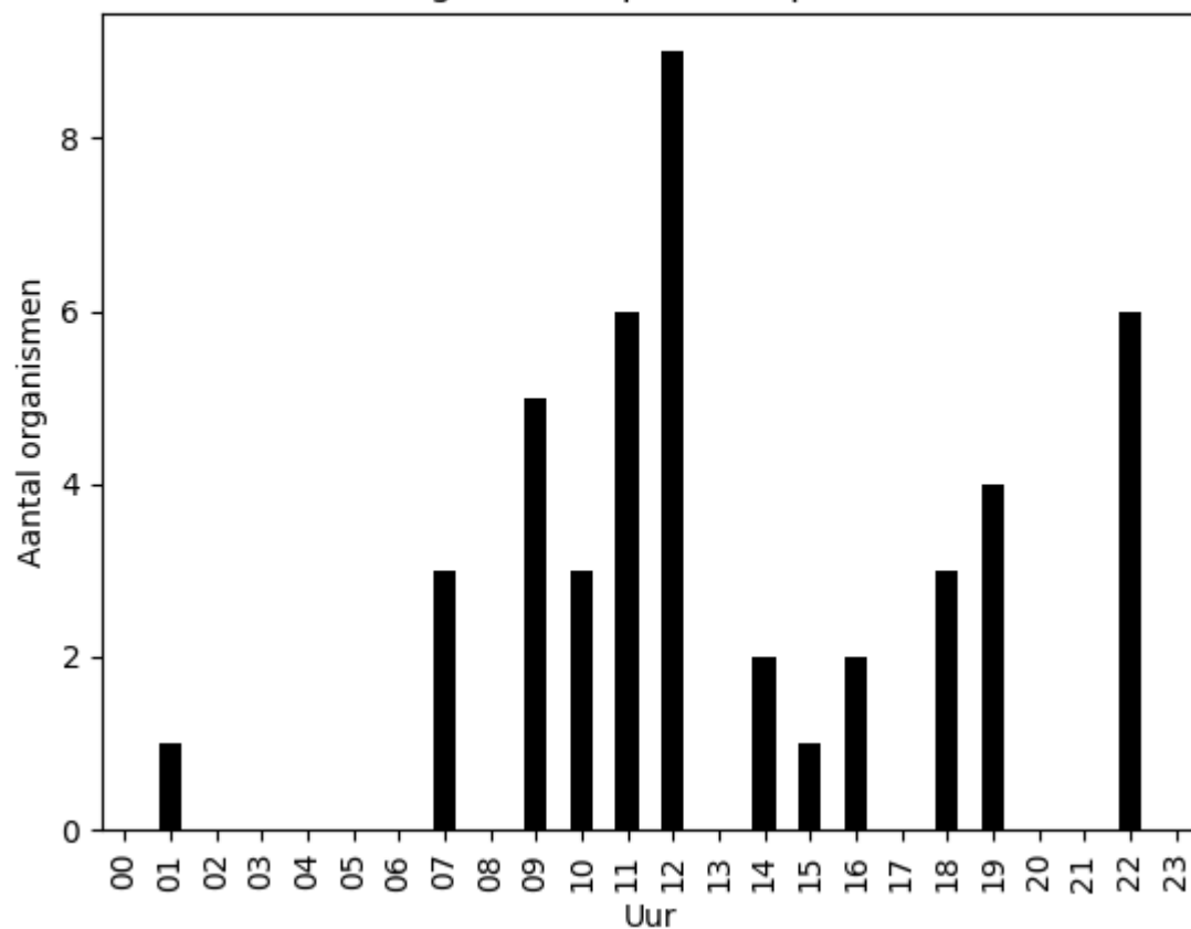
Aantal organismen per uur op 2020-08-02
