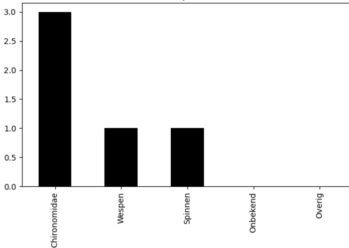
Voorkomen van ordes op 2020-09-10 (totaal = 5)
