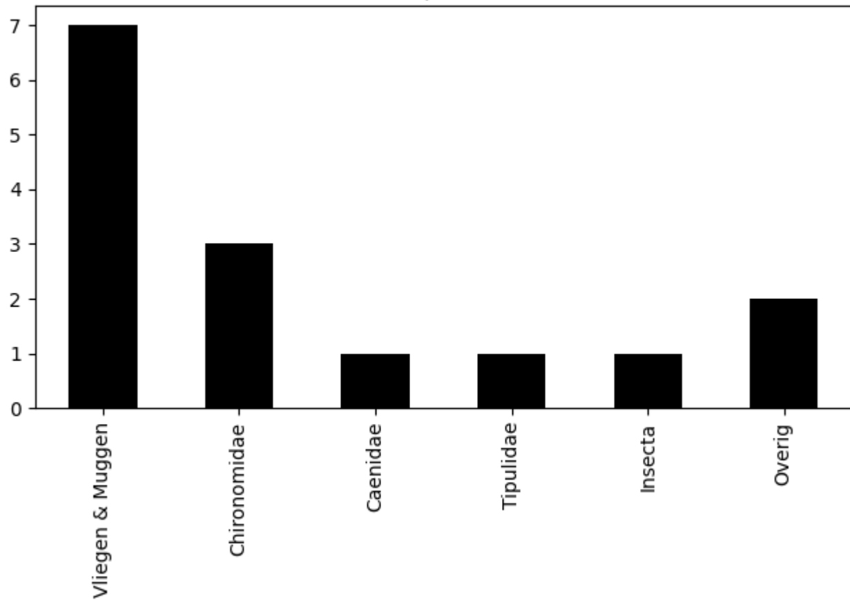
Voorkomen van ordes op 2020-09-12 (totaal = 15)
