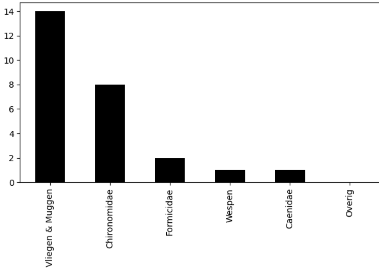
Voorkomen van ordes op 2020-09-11 (totaal = 26)
