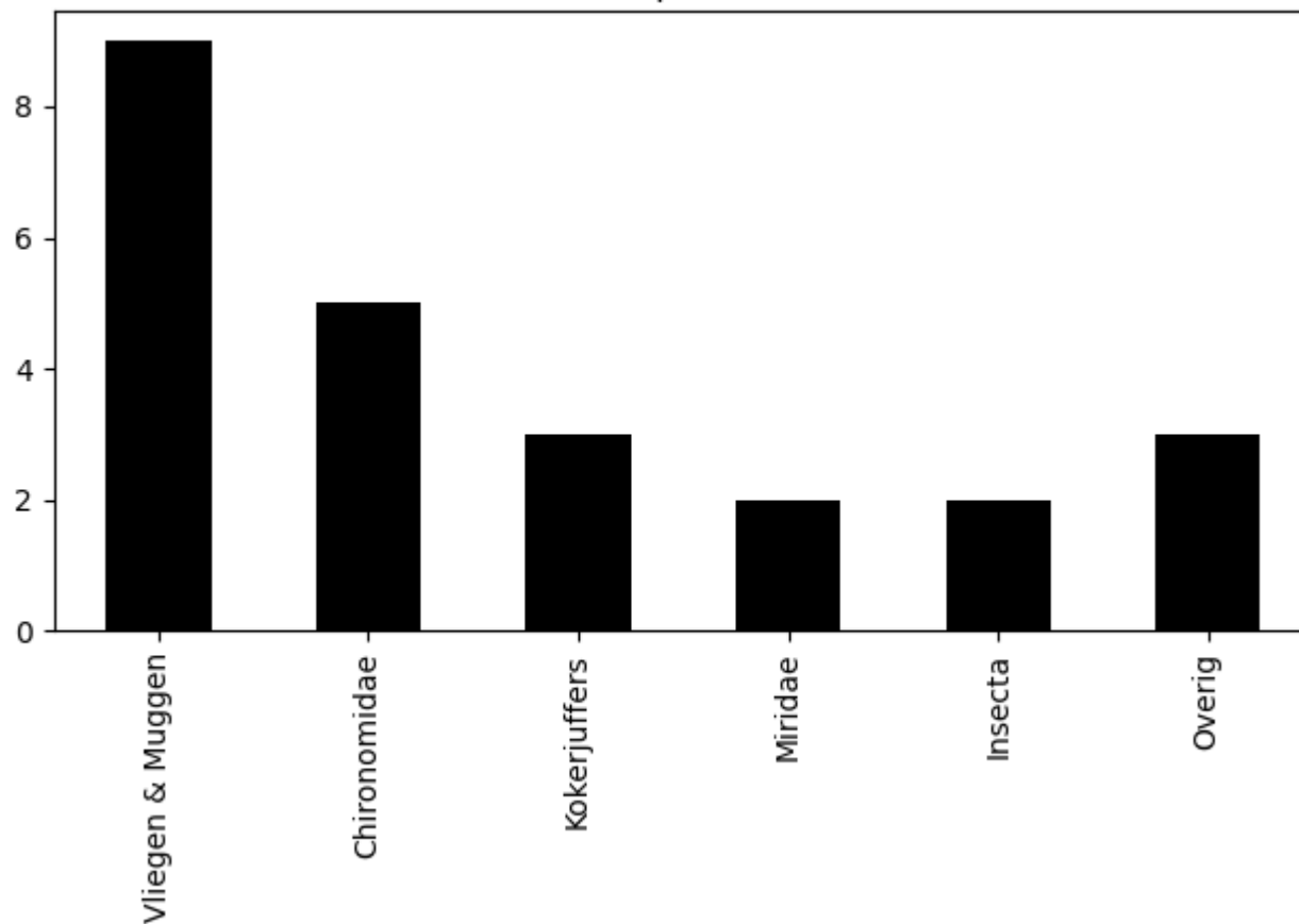
Voorkomen van ordes op 2020-09-09 (totaal = 24)
