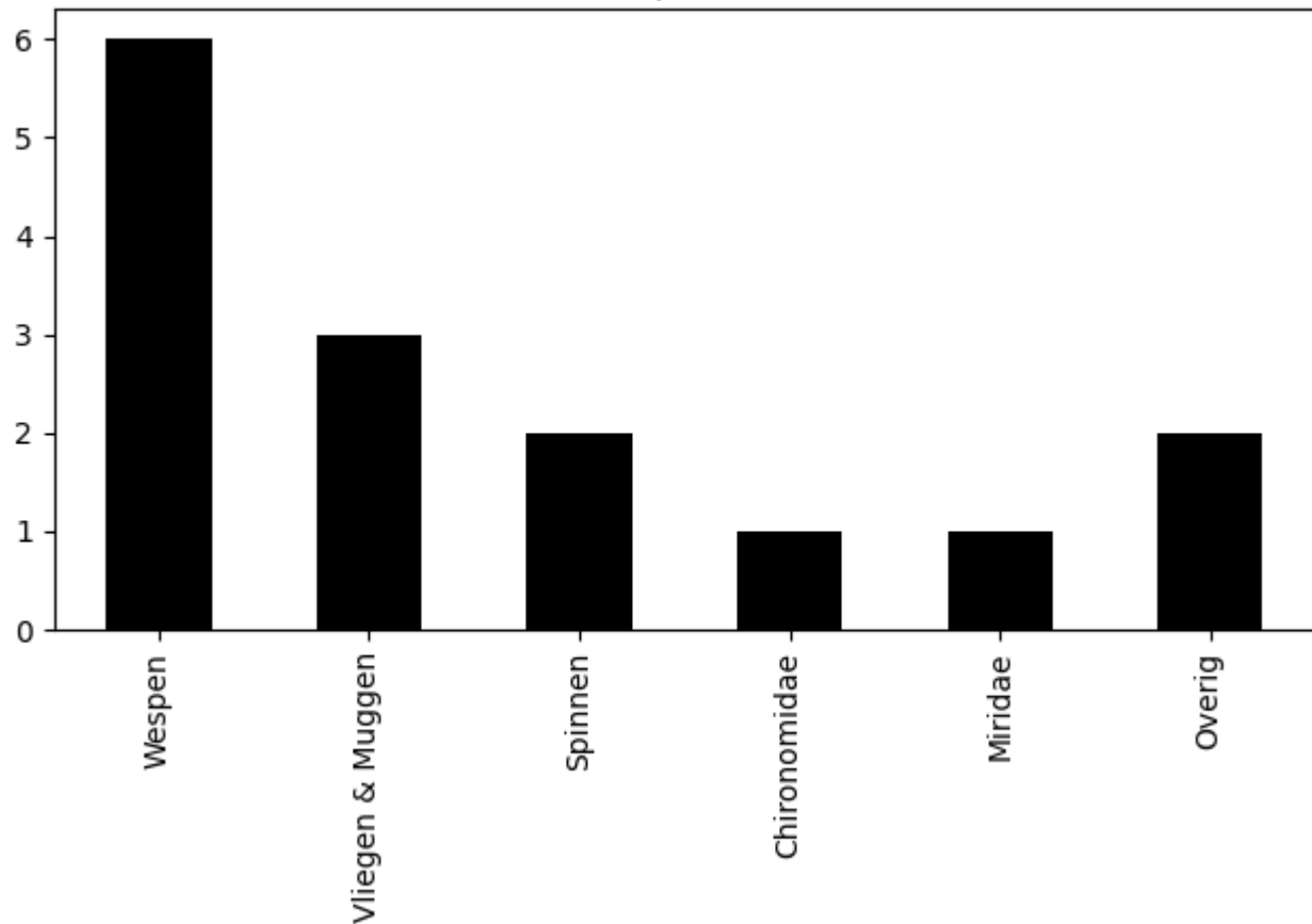
Voorkomen van ordes op 2020-09-14 (totaal = 15)
