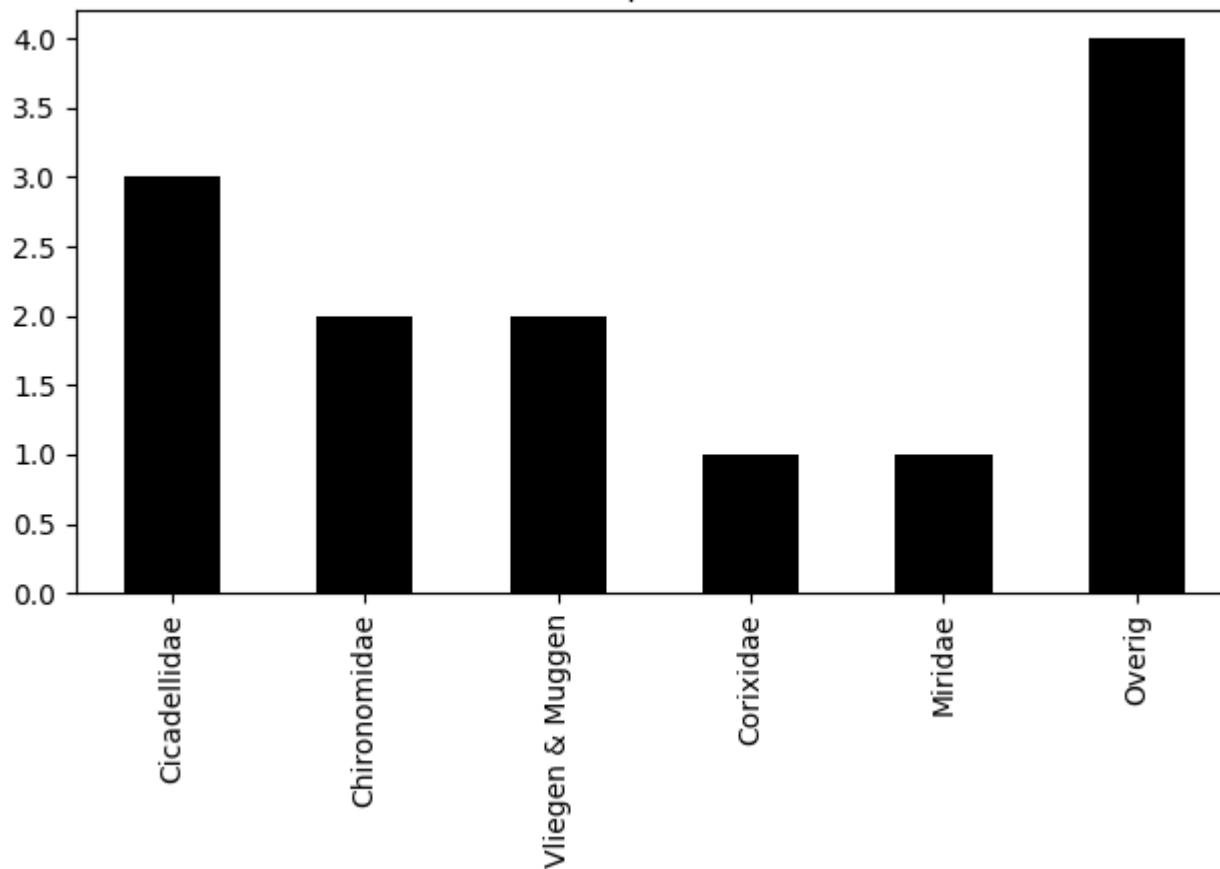
Voorkomen van ordes op 2020-09-16 (totaal = 13)
