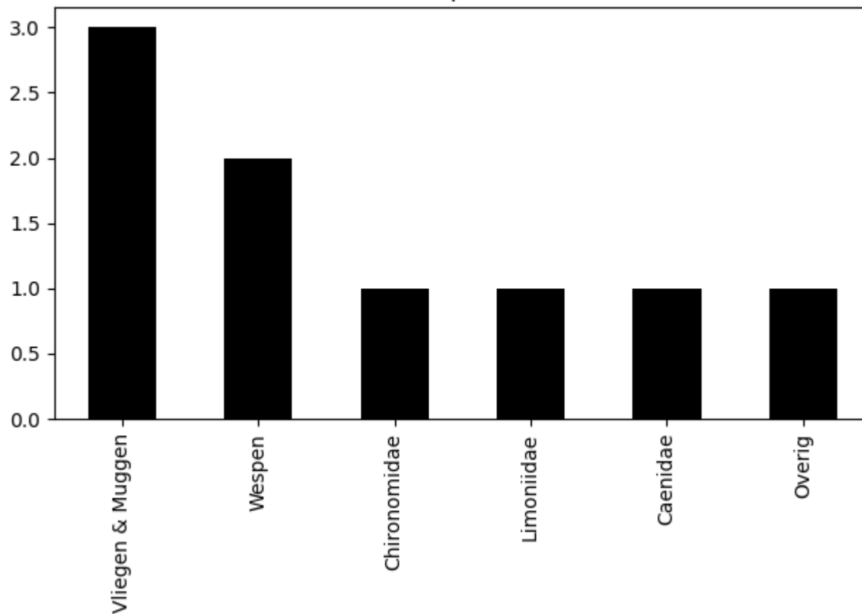
Voorkomen van ordes op 2020-08-17 (totaal = 9)
