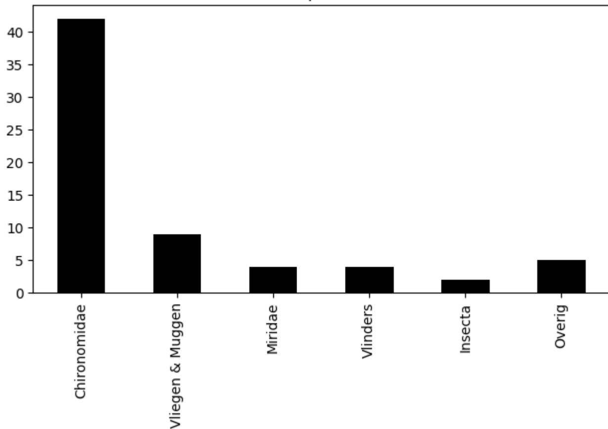
Voorkomen van ordes op 2020-08-14 (totaal = 66)
