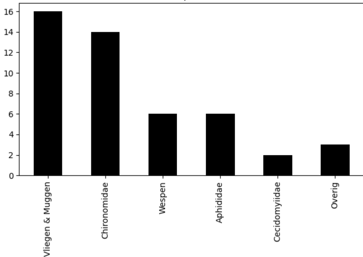
Voorkomen van ordes op 2020-07-26 (totaal = 47)
