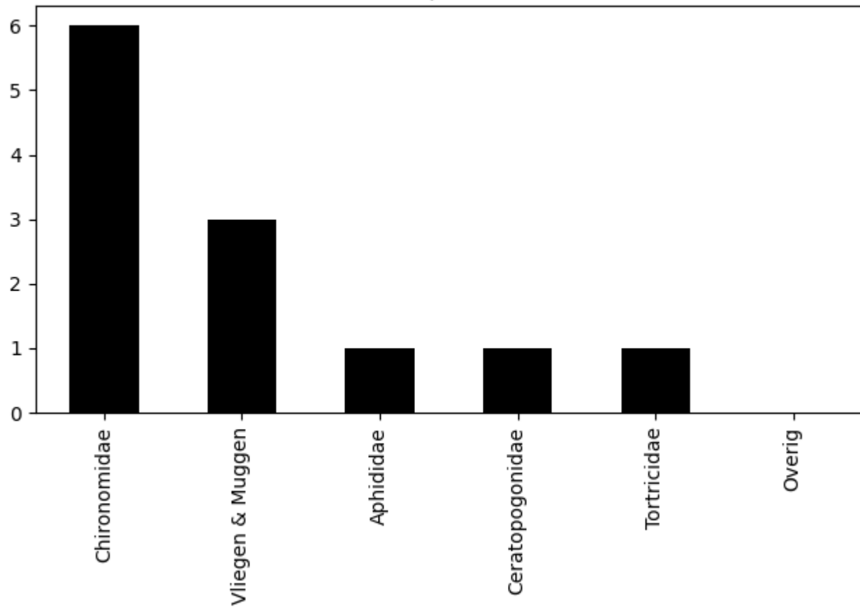
Voorkomen van ordes op 2020-07-30 (totaal = 12)
