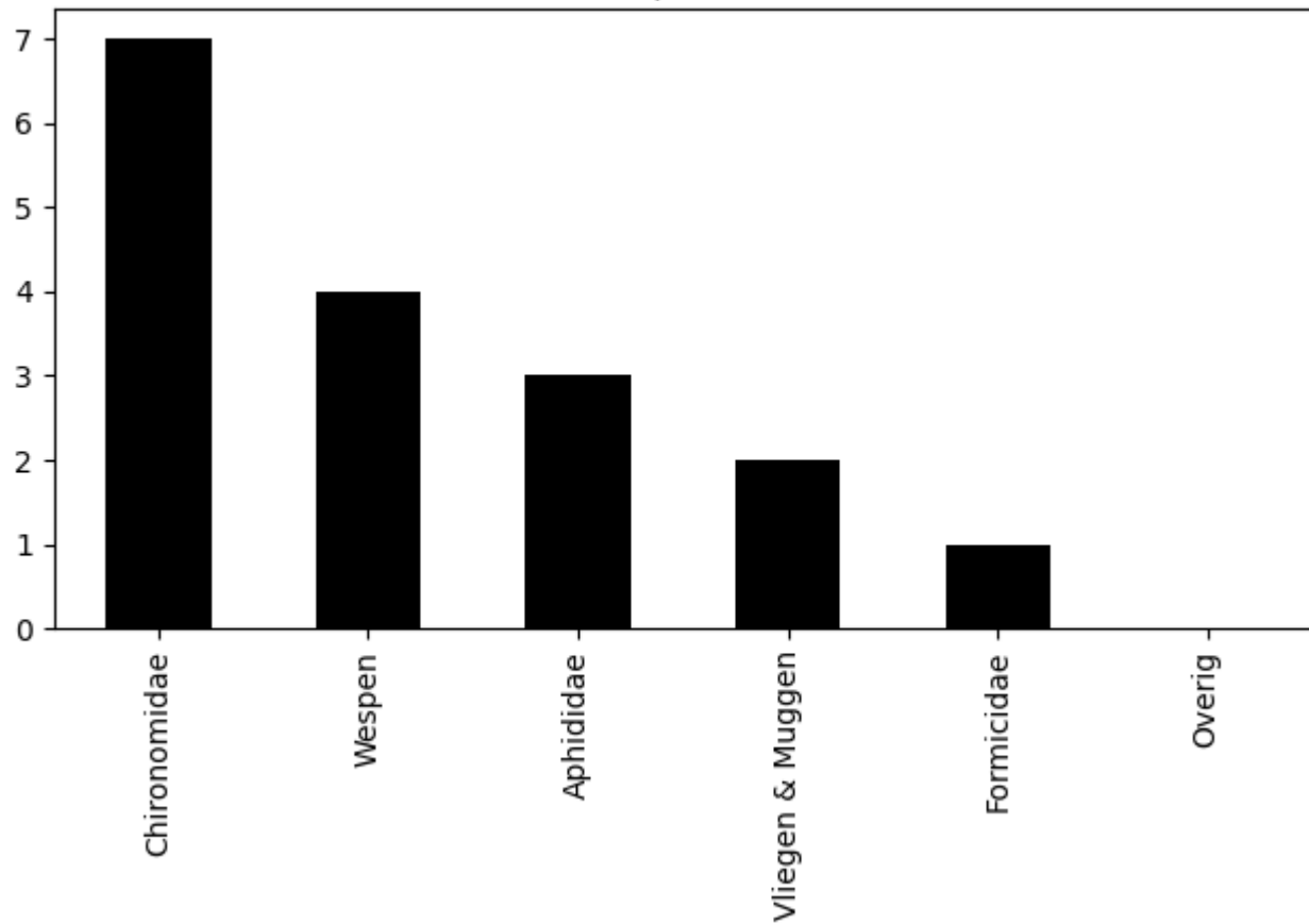
Voorkomen van ordes op 2020-07-23 (totaal = 17)
