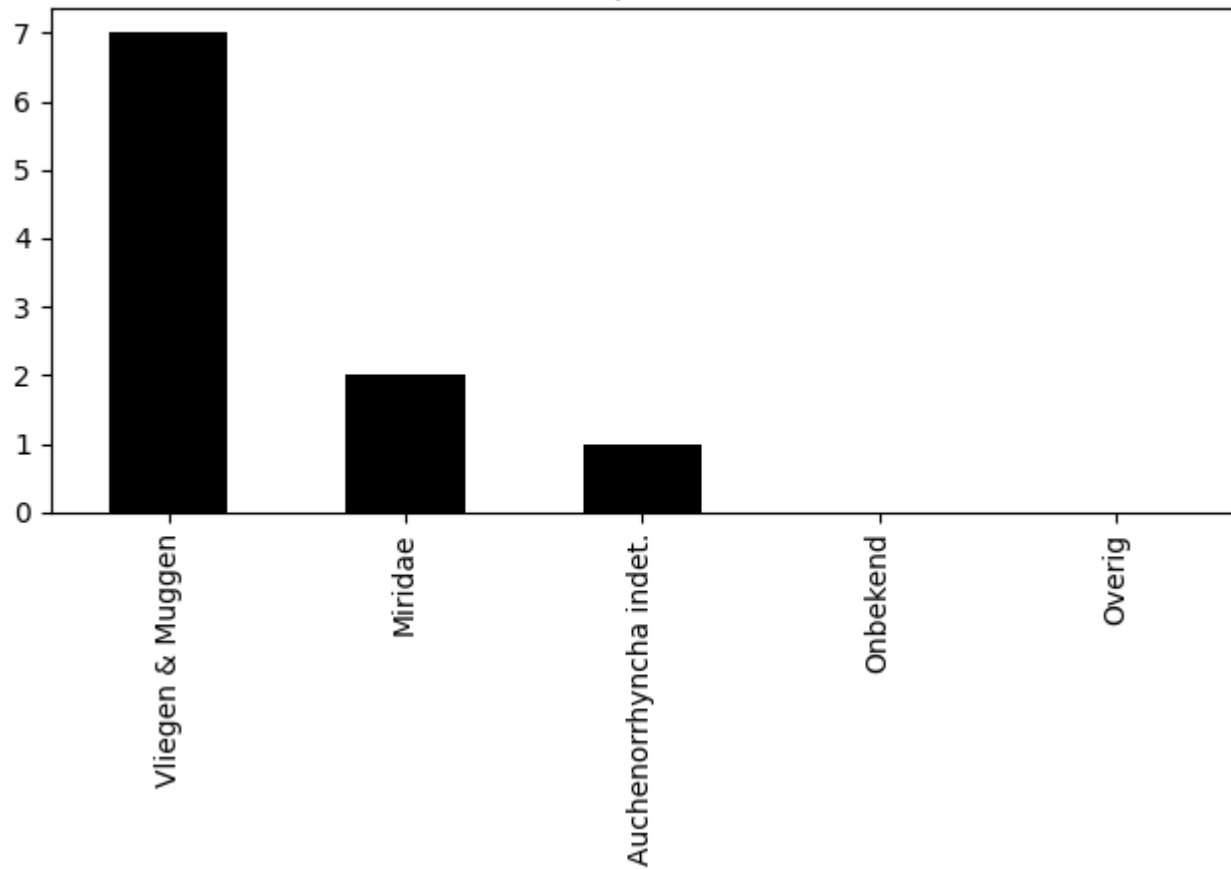
Voorkomen van ordes op 2020-07-28 (totaal = 10)
