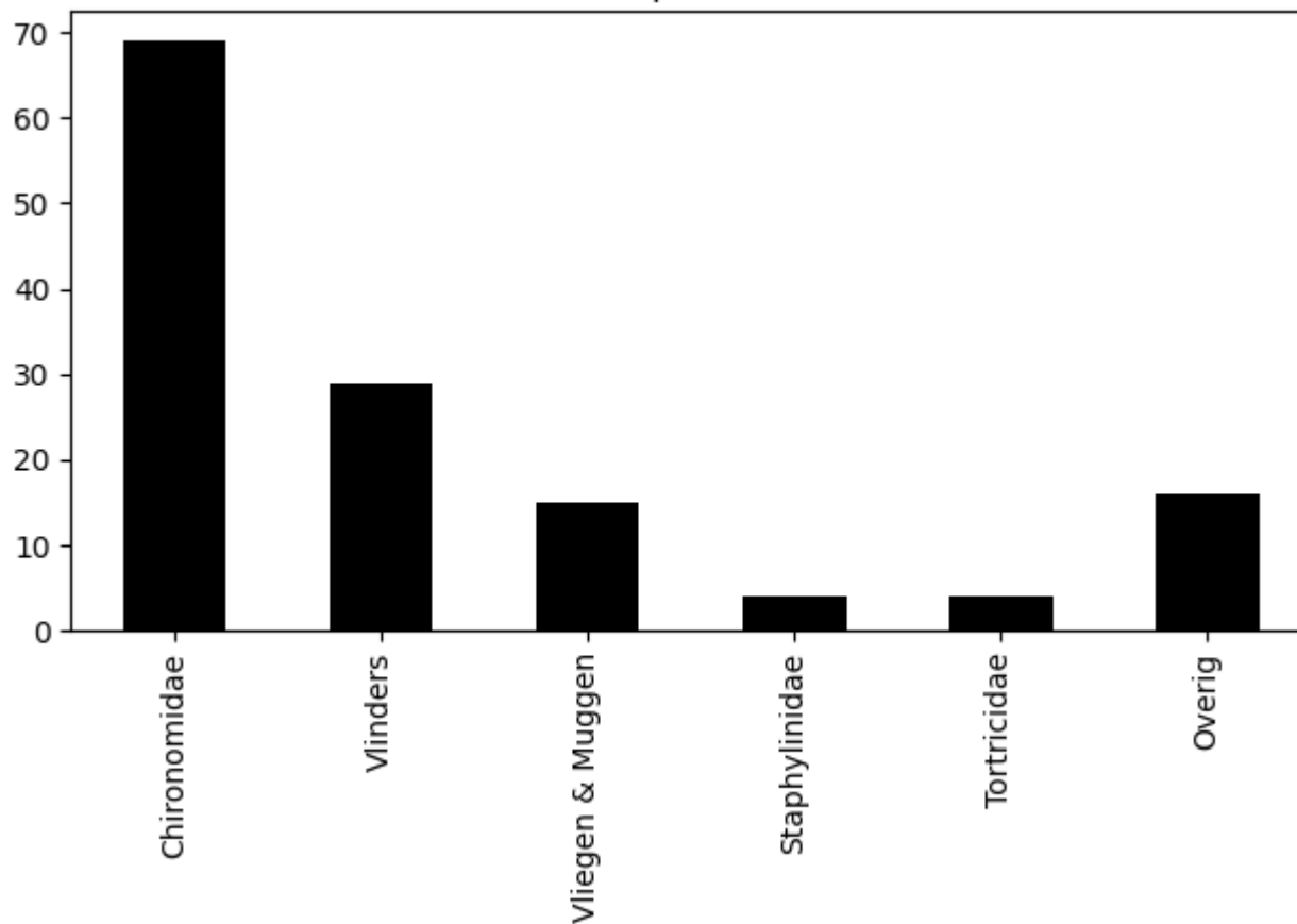
Voorkomen van ordes op 2020-08-08 (totaal = 137)
