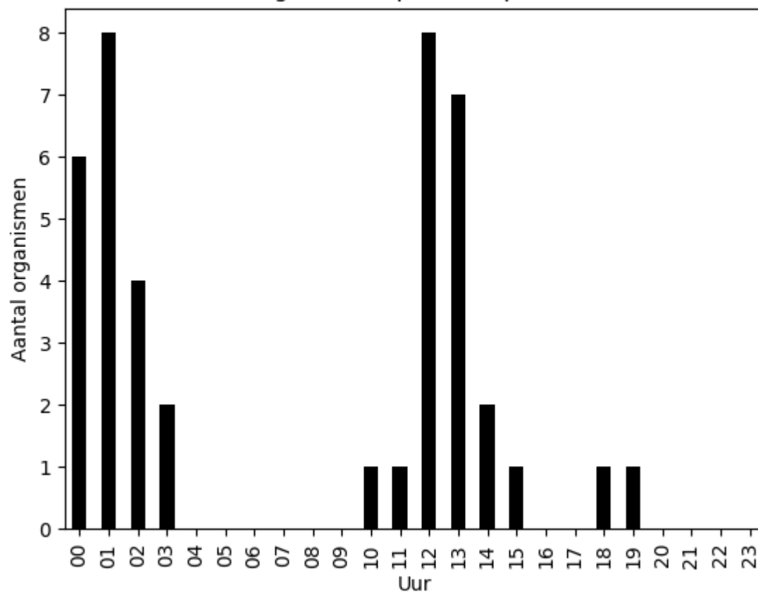
Aantal organismen per uur op 2020-09-05
