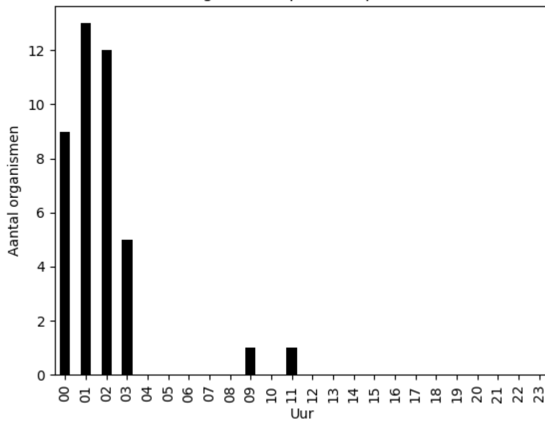
Aantal organismen per uur op 2020-09-17
