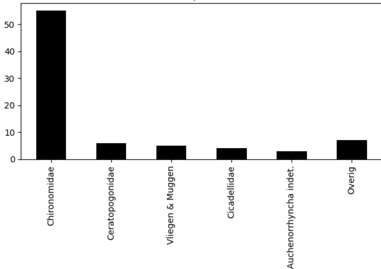
Voorkomen van ordes op 2020-08-21 (totaal = 80)
