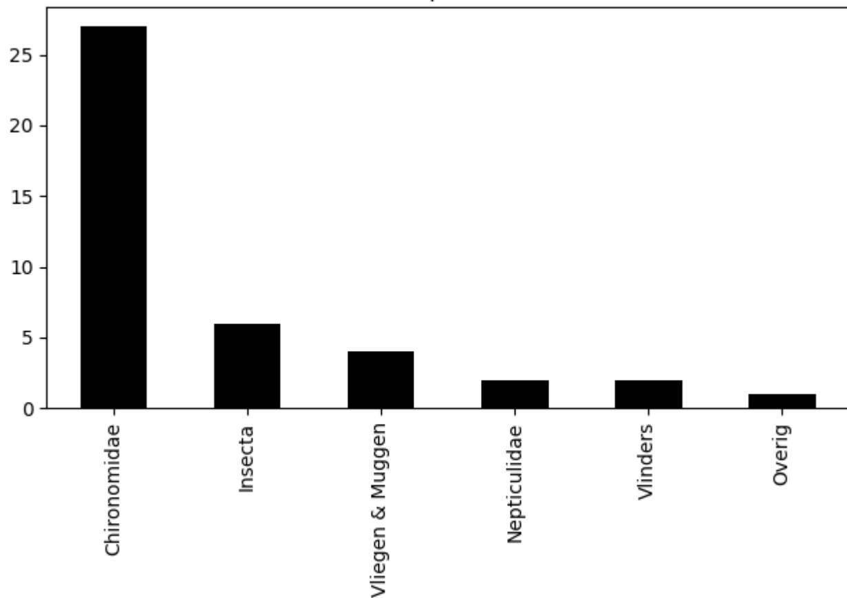
Voorkomen van ordes op 2020-07-26 (totaal = 42)
