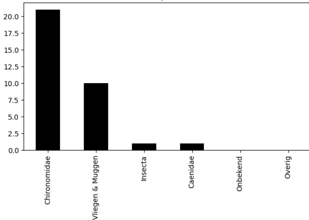
Voorkomen van ordes op 2020-08-24 (totaal = 33)
