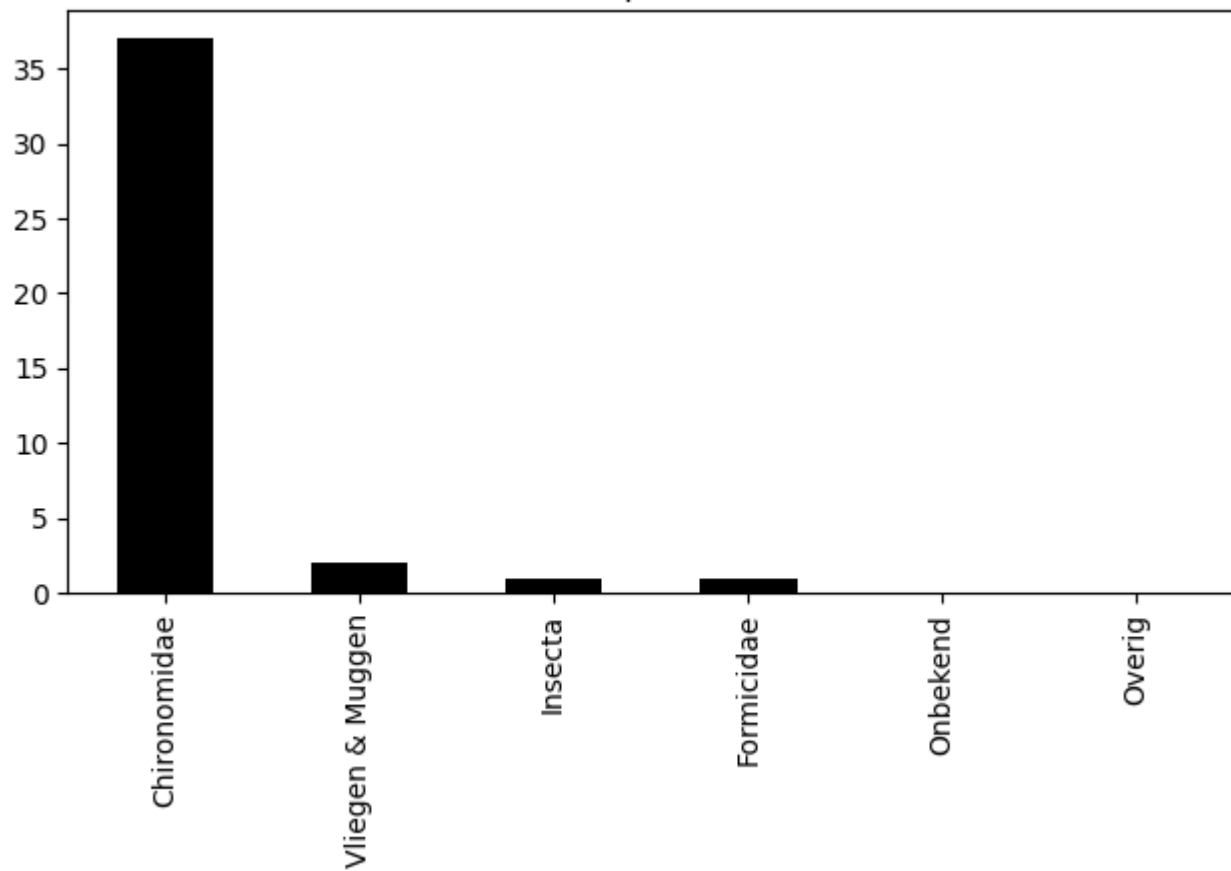
Voorkomen van ordes op 2020-09-17 (totaal = 41)
