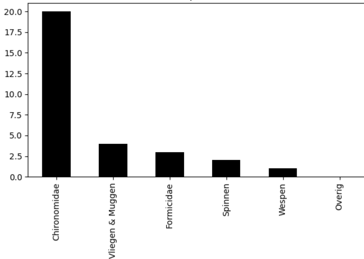
Voorkomen van ordes op 2020-09-11 (totaal = 30)
