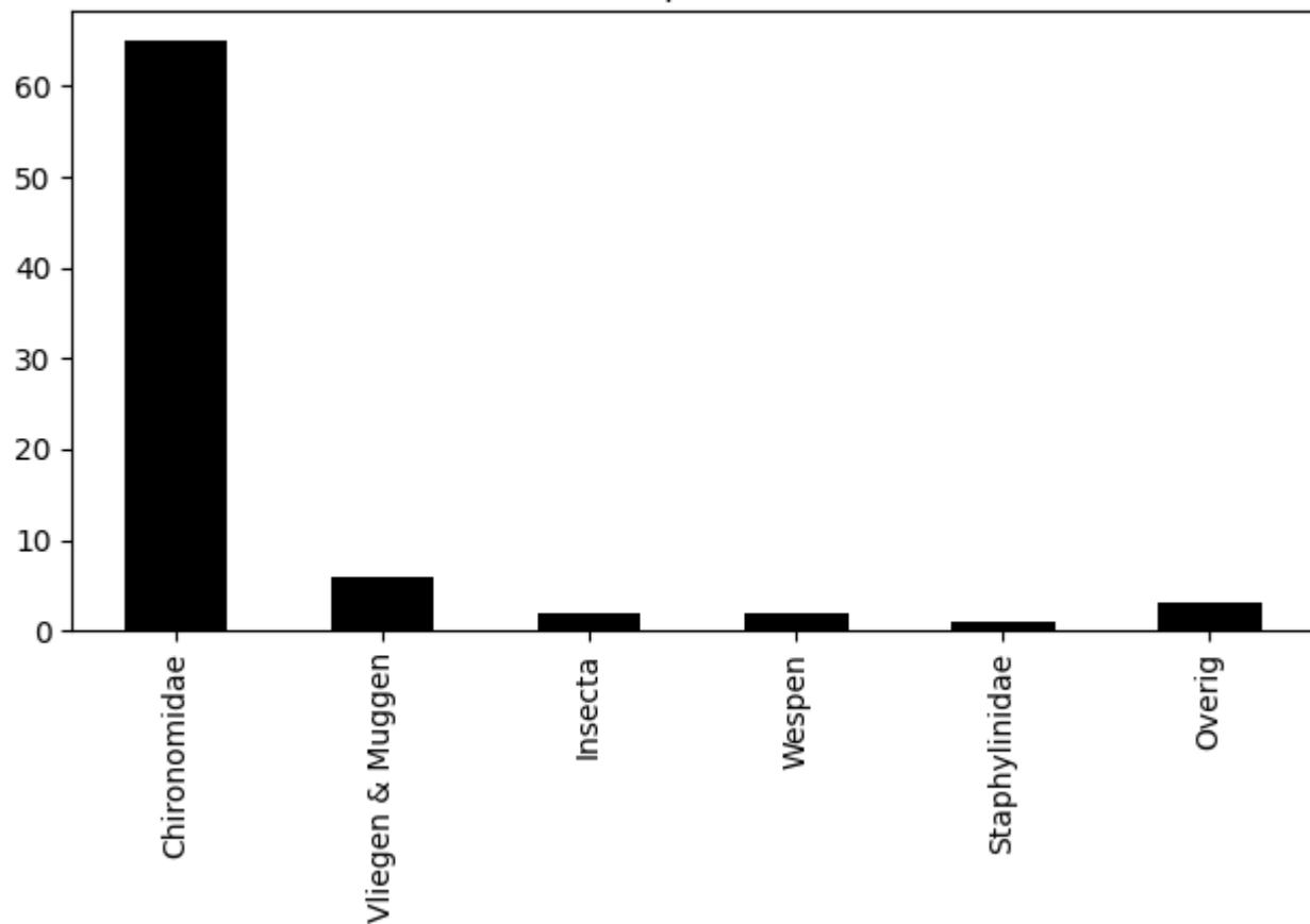
Voorkomen van ordes op 2020-07-19 (totaal = 79)
