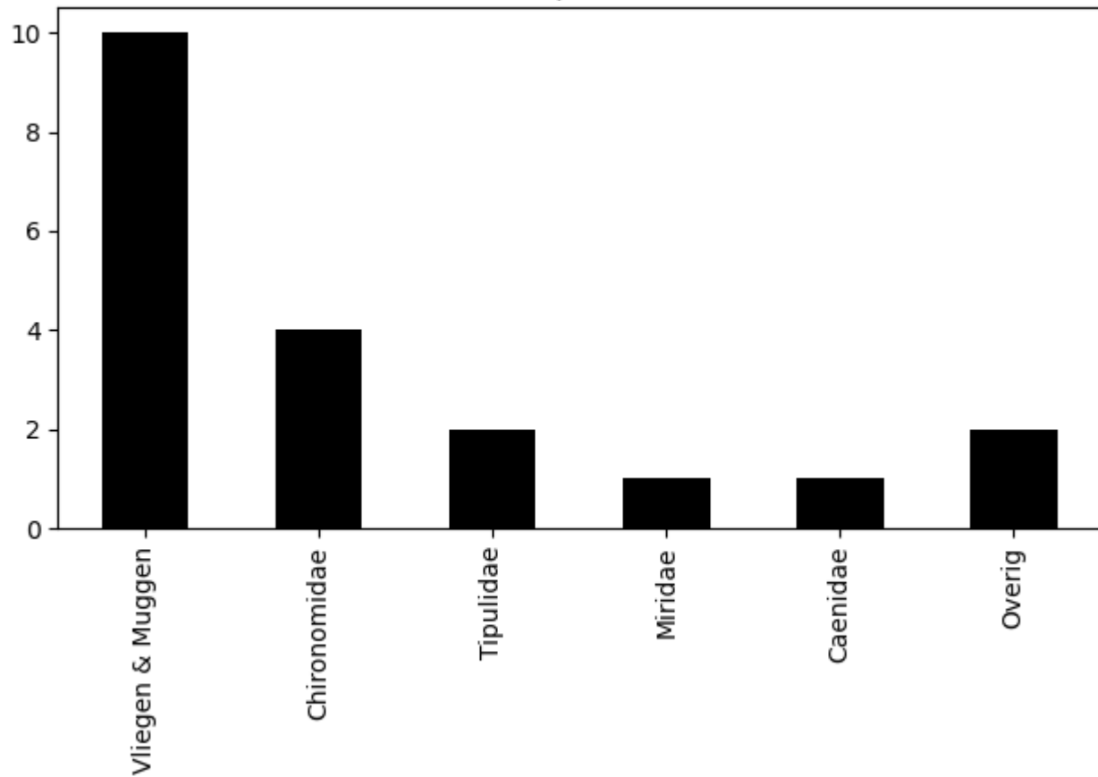
Voorkomen van ordes op 2020-07-16 (totaal = 20)
