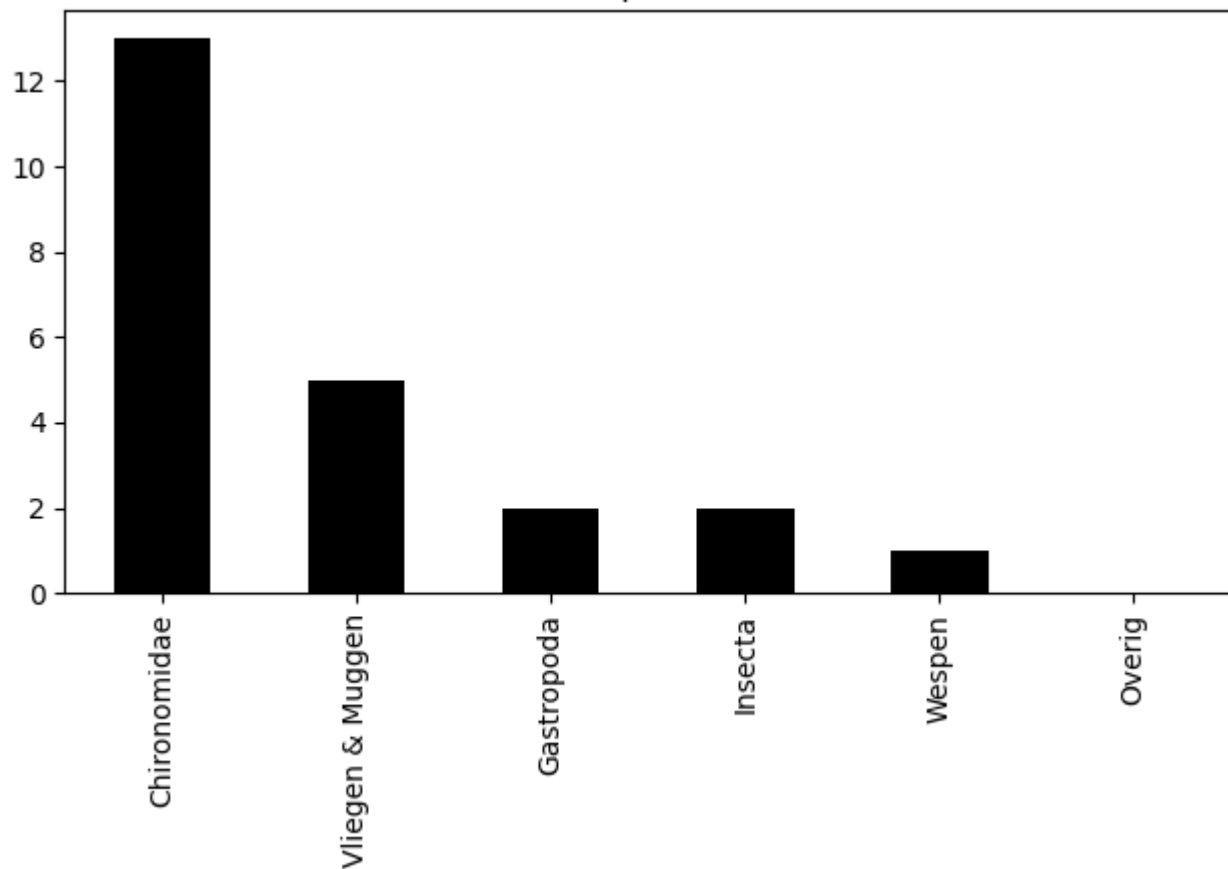
Voorkomen van ordes op 2020-08-28 (totaal = 23)
