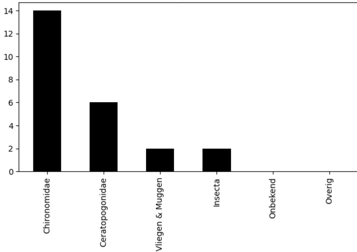
Voorkomen van ordes op 2020-08-27 (totaal = 24)
