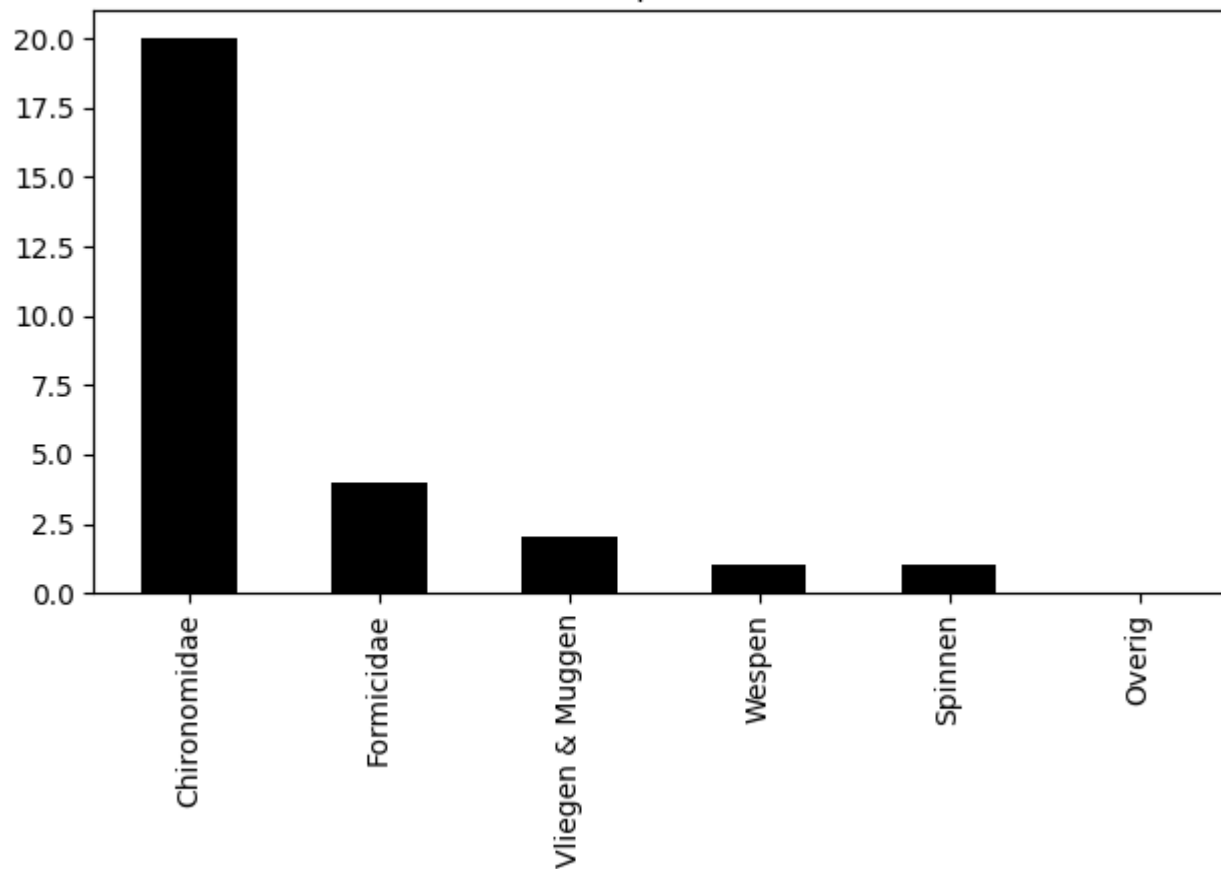
Voorkomen van ordes op 2020-09-13 (totaal = 28)
