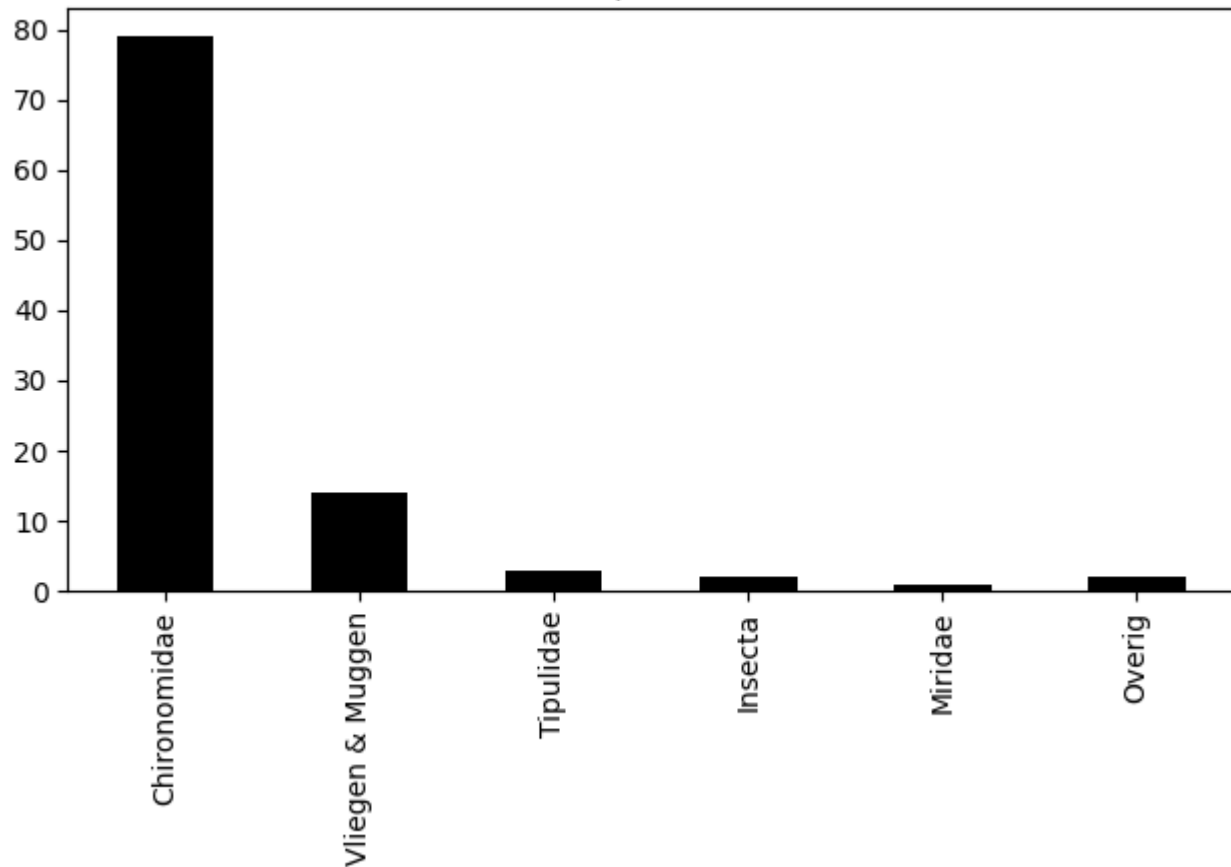
Voorkomen van ordes op 2020-08-03 (totaal = 101)
