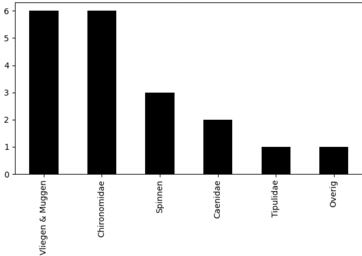
Voorkomen van ordes op 2020-09-10 (totaal = 19)
