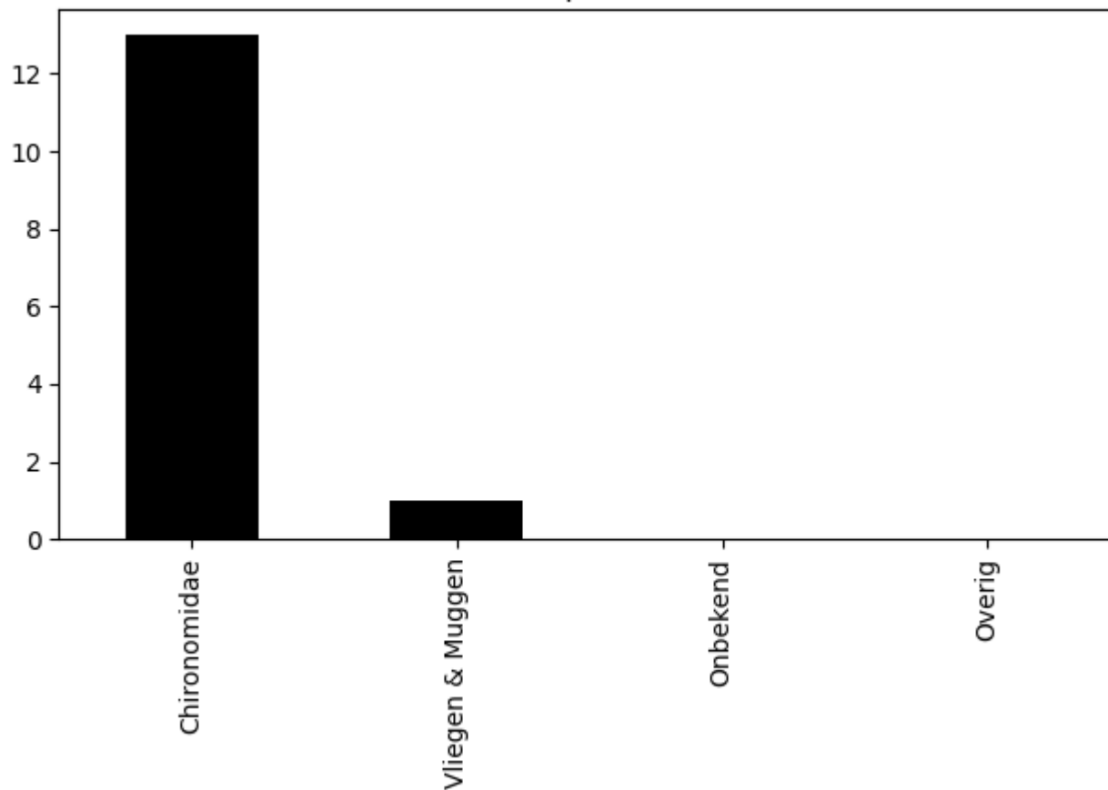
Voorkomen van ordes op 2020-08-26 (totaal = 14)
