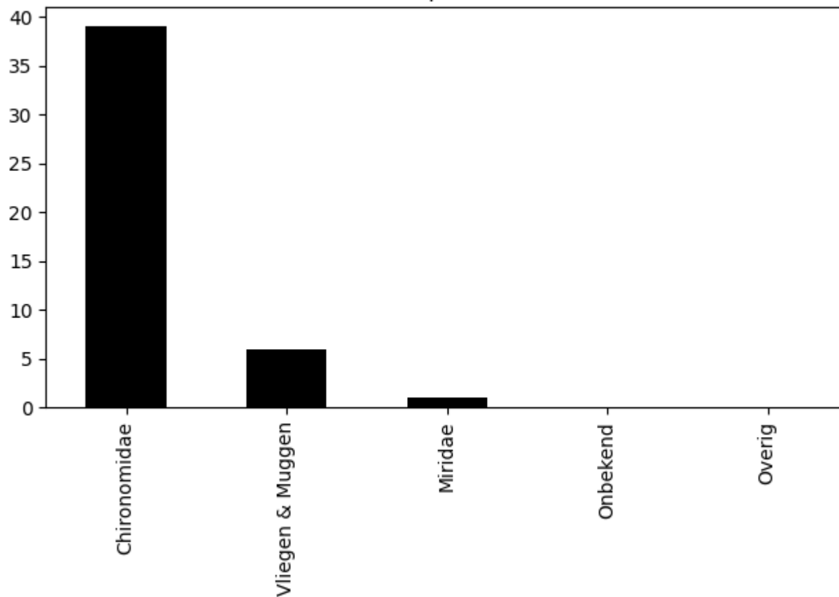
Voorkomen van ordes op 2020-07-23 (totaal = 46)
