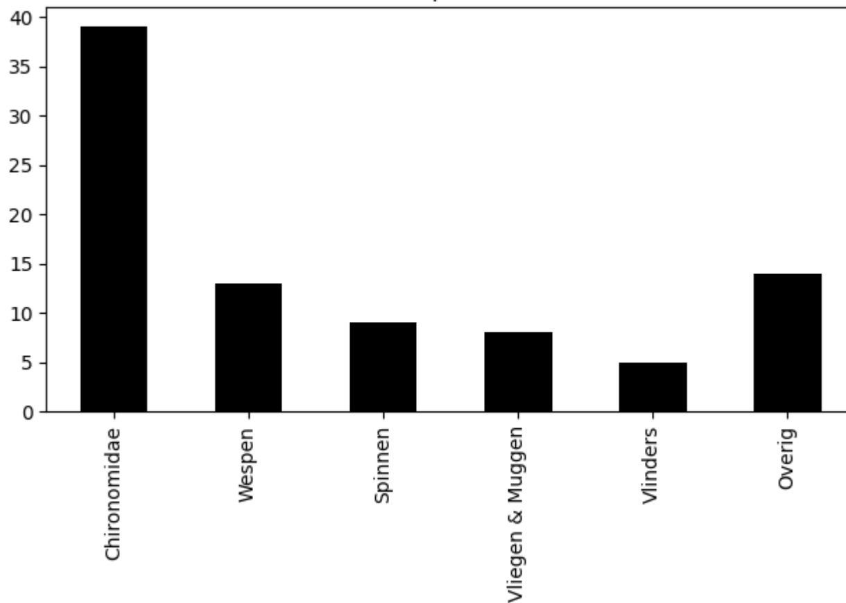
Voorkomen van ordes op 2020-08-17 (totaal = 88)
