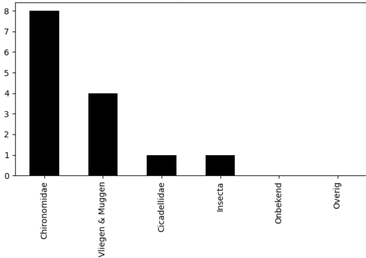
Voorkomen van ordes op 2020-08-25 (totaal = 14)
