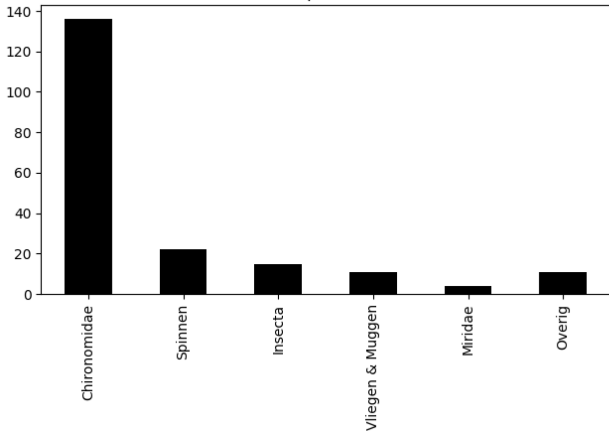
Voorkomen van ordes op 2020-08-18 (totaal = 199)
