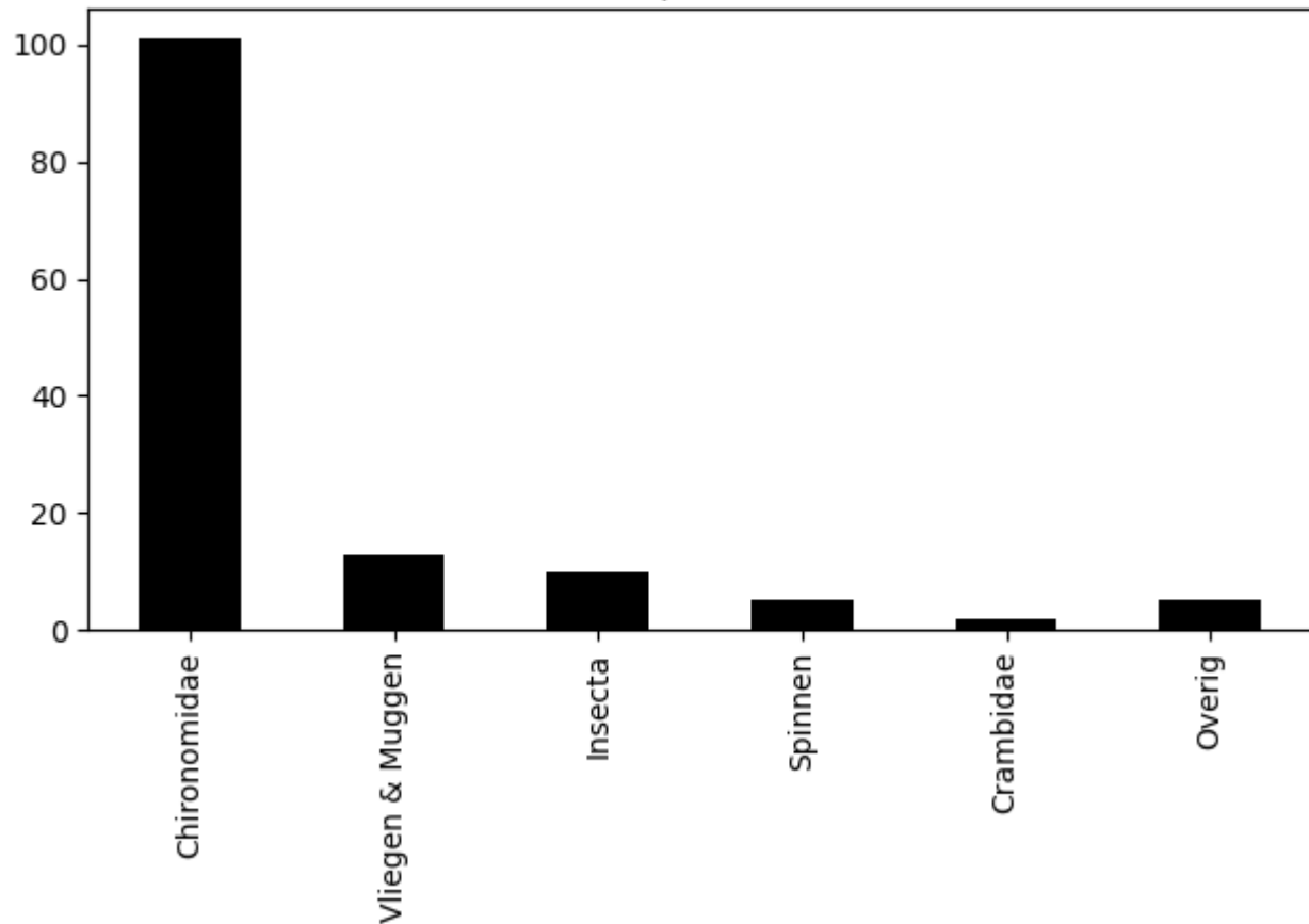
Voorkomen van ordes op 2020-07-22 (totaal = 136)
