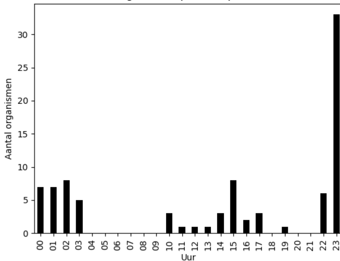
Aantal organismen per uur op 2020-07-10
