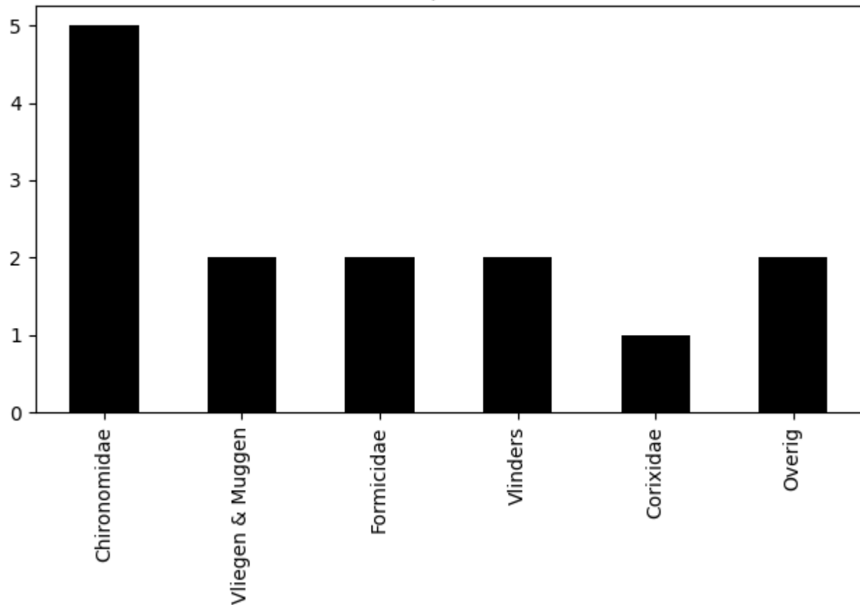
Voorkomen van ordes op 2020-09-08 (totaal = 14)
