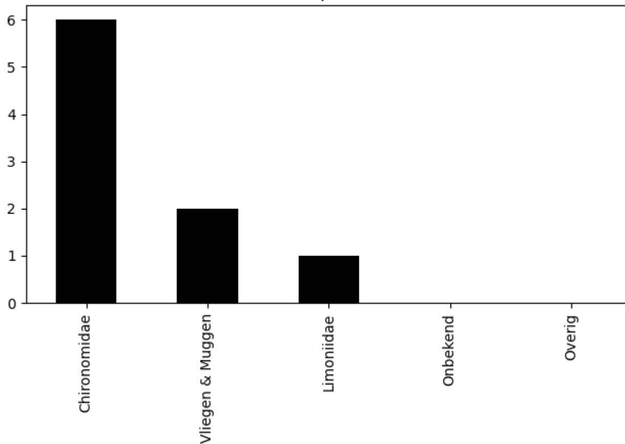
Voorkomen van ordes op 2020-07-09 (totaal = 9)
