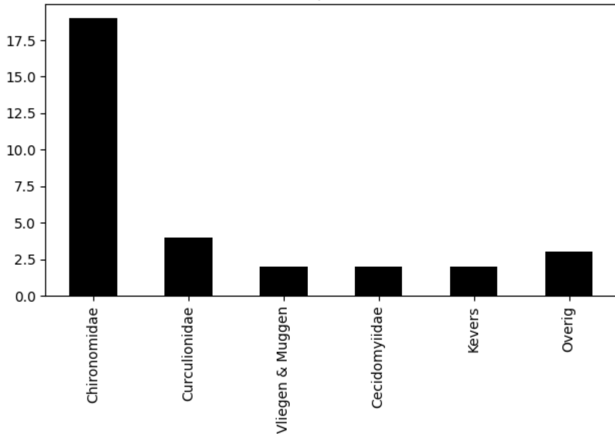
Voorkomen van ordes op 2020-07-18 (totaal = 32)
