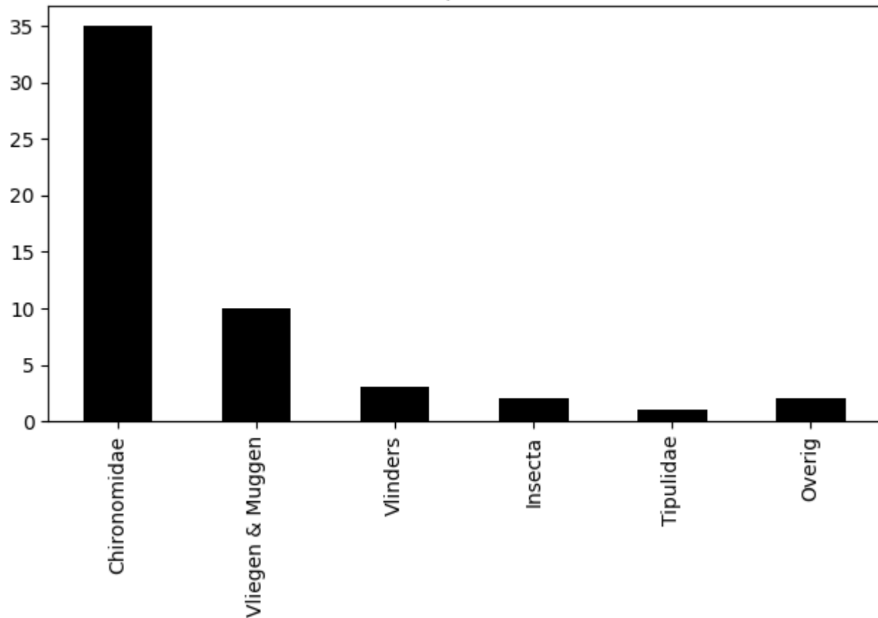
Voorkomen van ordes op 2020-07-20 (totaal = 53)
