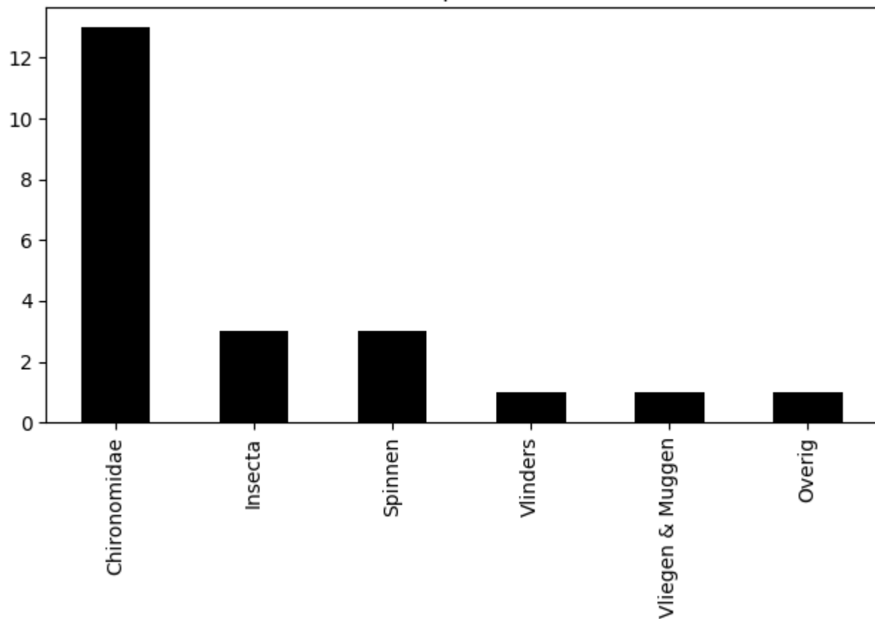
Voorkomen van ordes op 2020-09-16 (totaal = 22)
