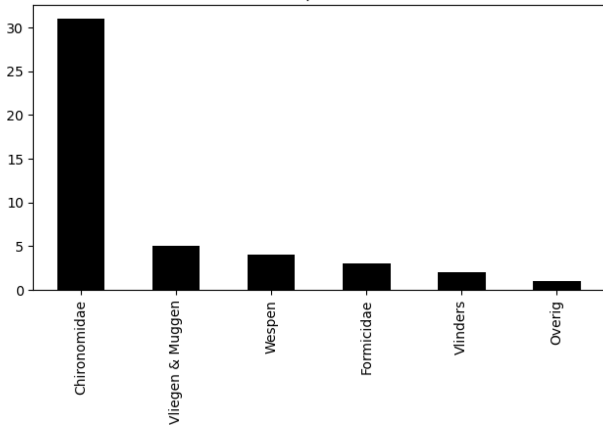
Voorkomen van ordes op 2020-08-23 (totaal = 46)
