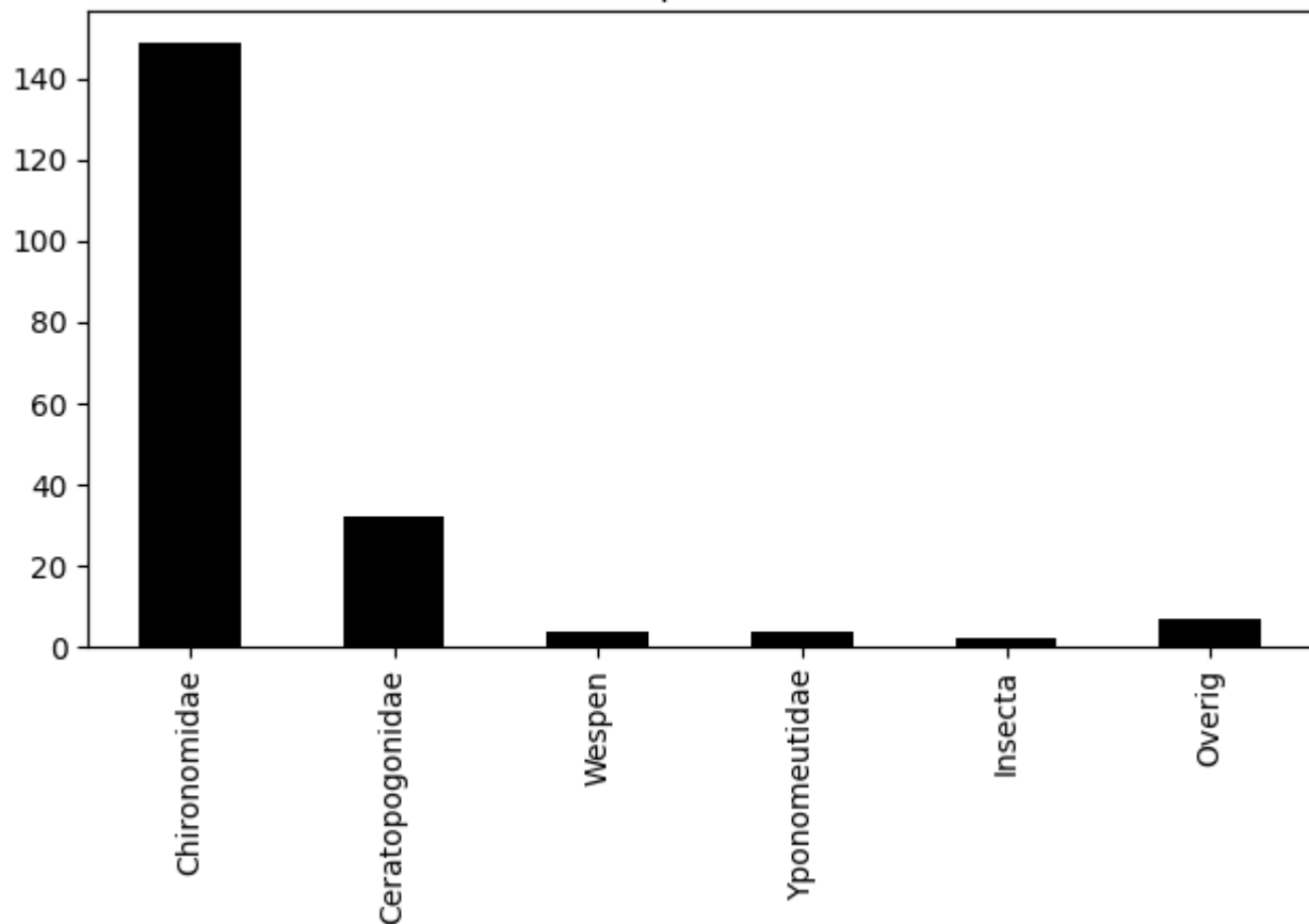
Voorkomen van ordes op 2020-08-09 (totaal = 198)
