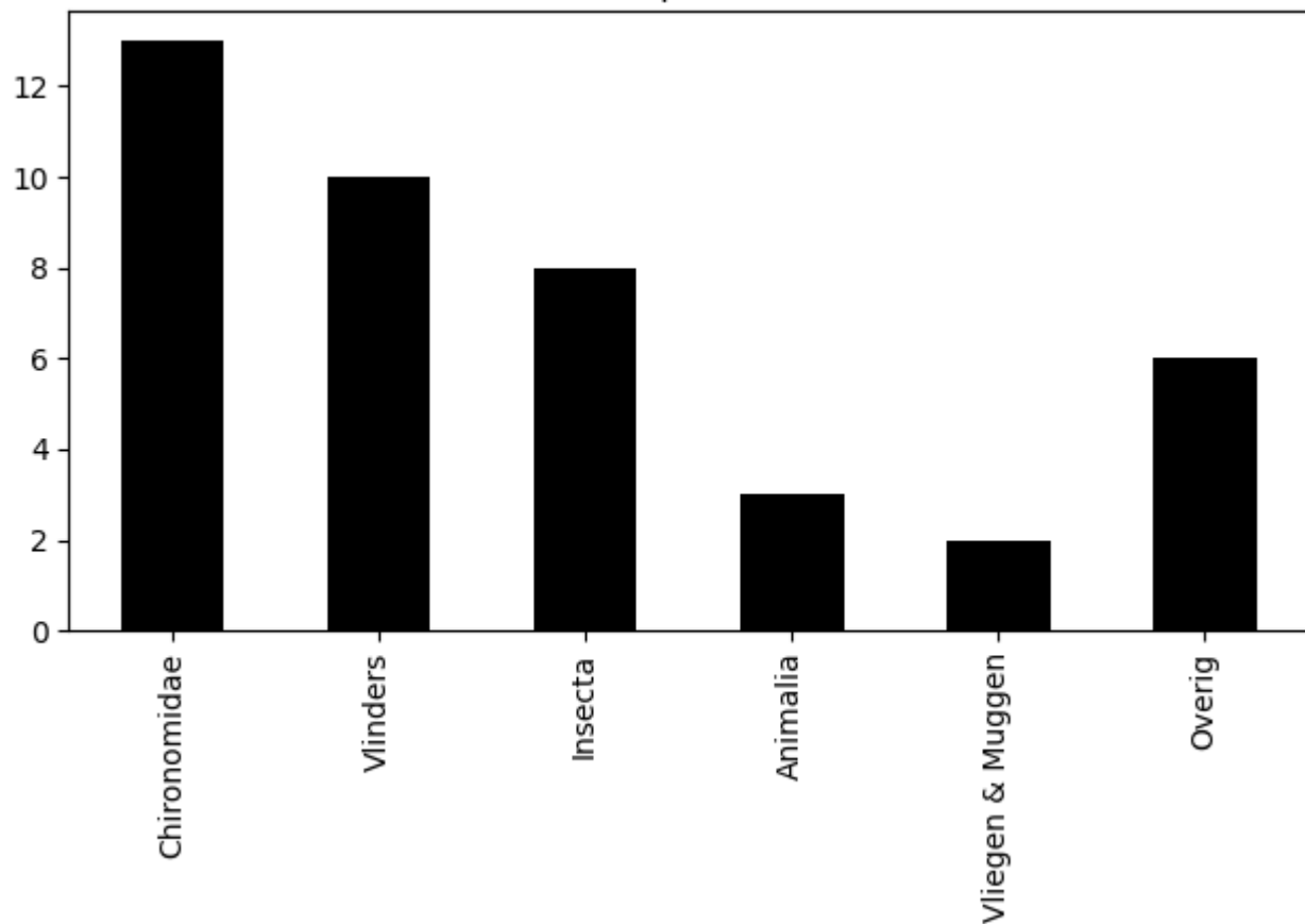
Voorkomen van ordes op 2020-08-06 (totaal = 42)
