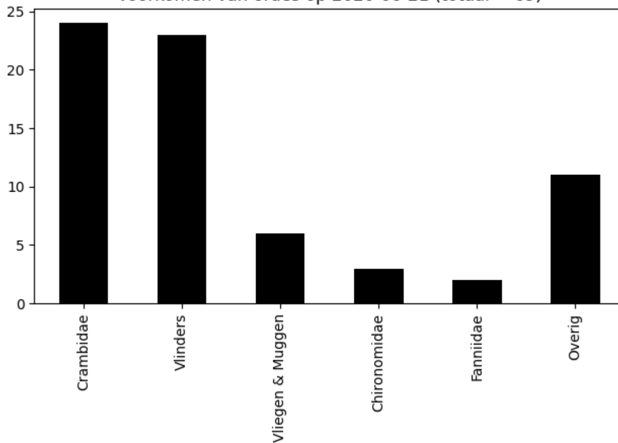
Voorkomen van ordes op 2020-06-21 (totaal = 69)
