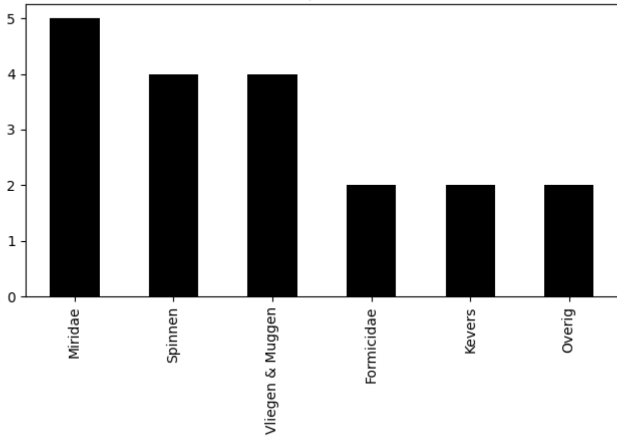
Voorkomen van ordes op 2020-06-10 (totaal = 19)
