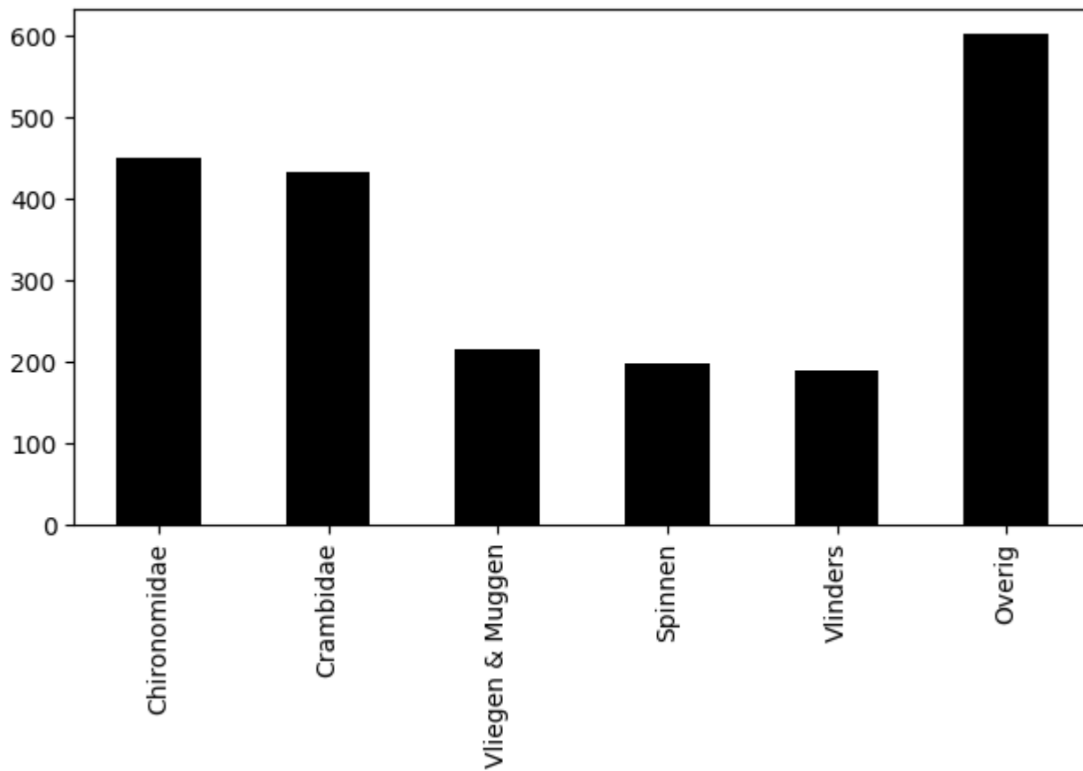
Voorkomen van ordes (totaal = 2088)
