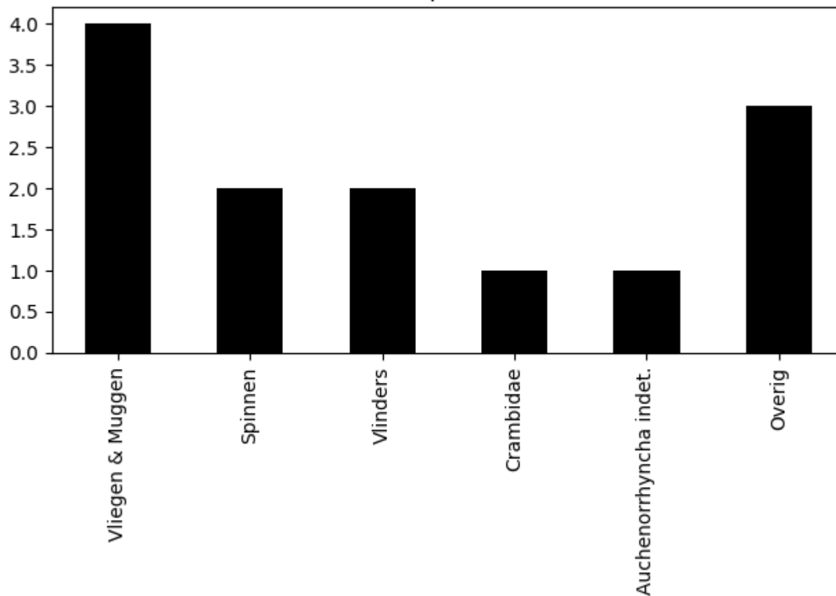
Voorkomen van ordes op 2020-07-05 (totaal = 13)
