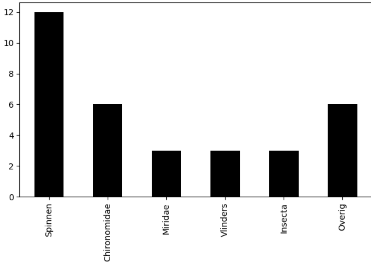
Voorkomen van ordes op 2020-07-06 (totaal = 33)
