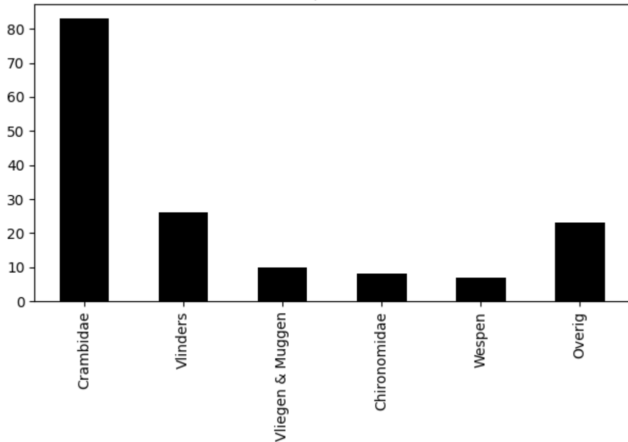
Voorkomen van ordes op 2020-07-03 (totaal = 157)
