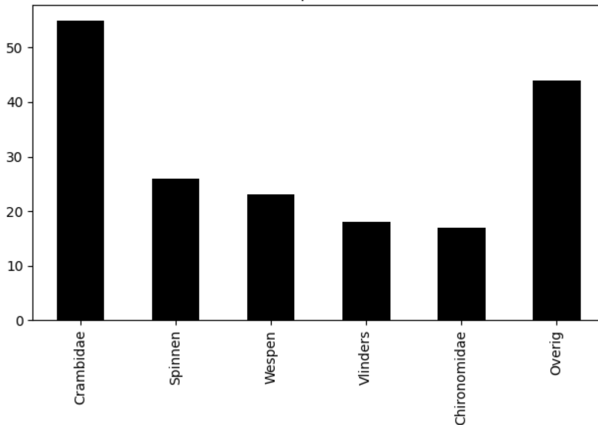
Voorkomen van ordes op 2020-06-20 (totaal = 183)
