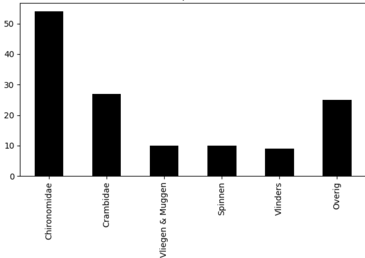
Voorkomen van ordes op 2020-06-19 (totaal = 135)
