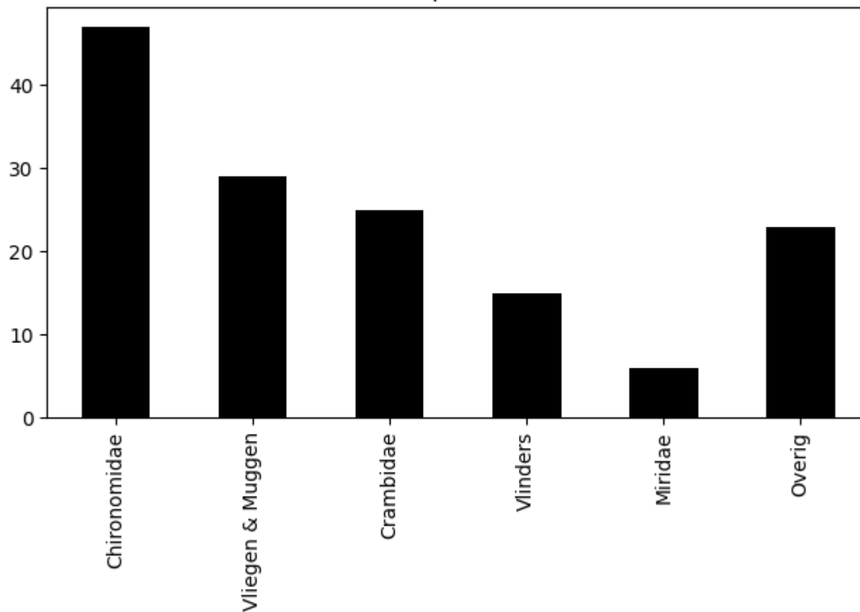
Voorkomen van ordes op 2020-06-13 (totaal = 145)
