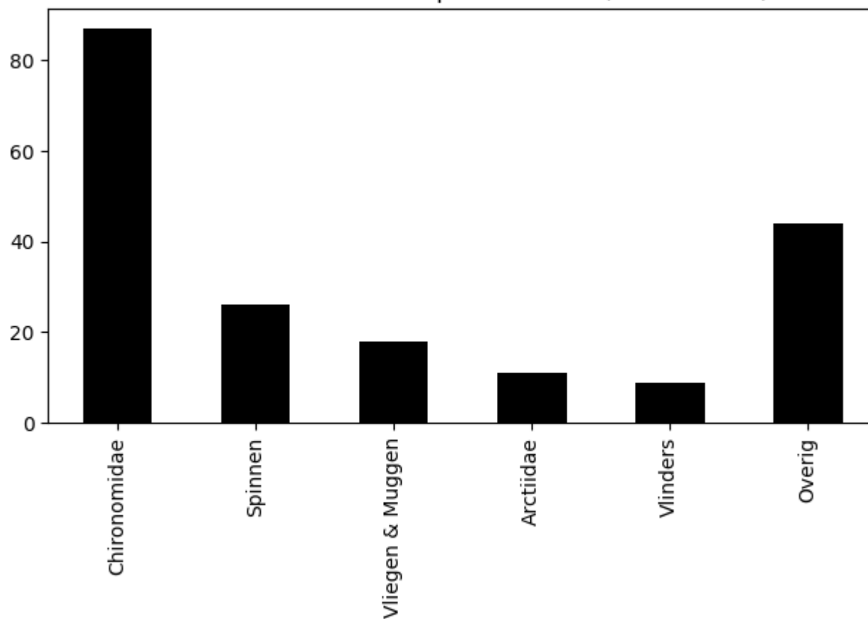
Voorkomen van ordes op 2020-06-14 (totaal = 195)
