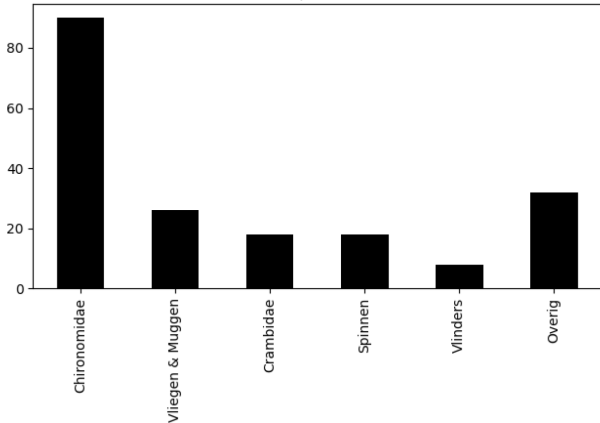
Voorkomen van ordes op 2020-06-15 (totaal = 192)
