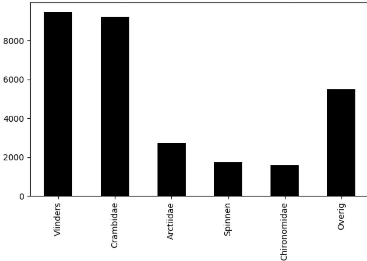
Verdeling biomassa per orde (totaal = 30 gram)
