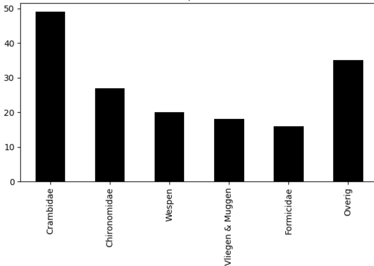
Voorkomen van ordes op 2020-06-18 (totaal = 165)
