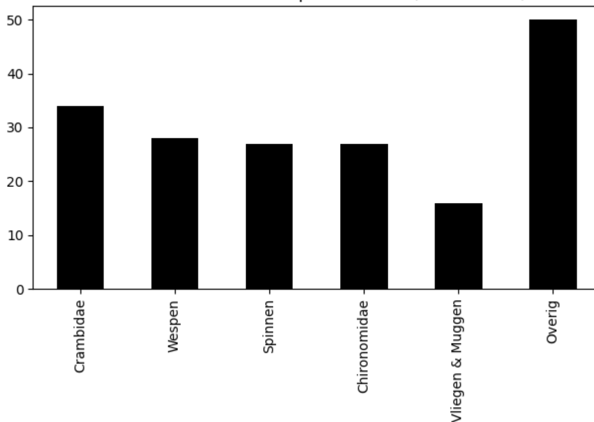
Voorkomen van ordes op 2020-06-17 (totaal = 182)
