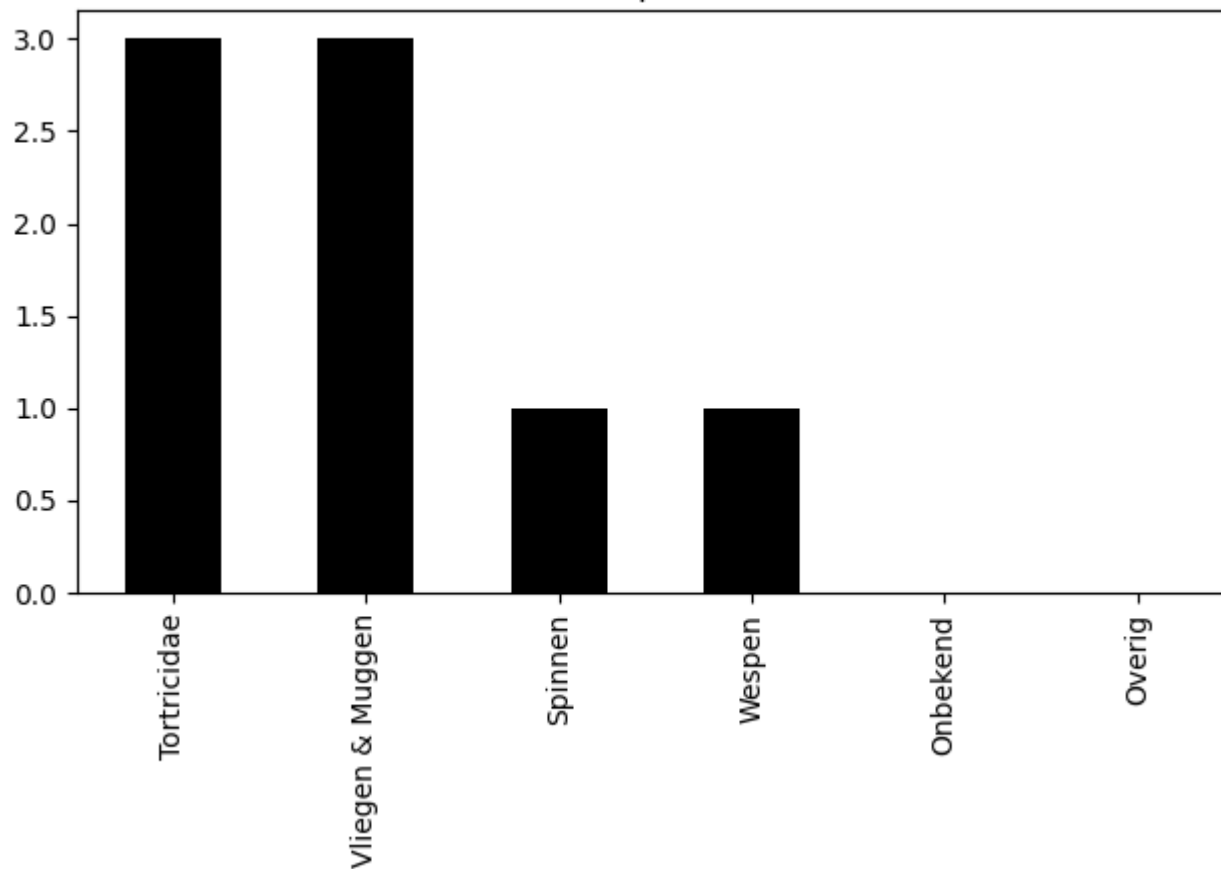
Voorkomen van ordes op 2020-07-02 (totaal = 8)
