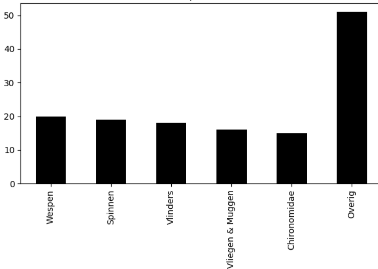
Voorkomen van ordes op 2020-06-11 (totaal = 139)
