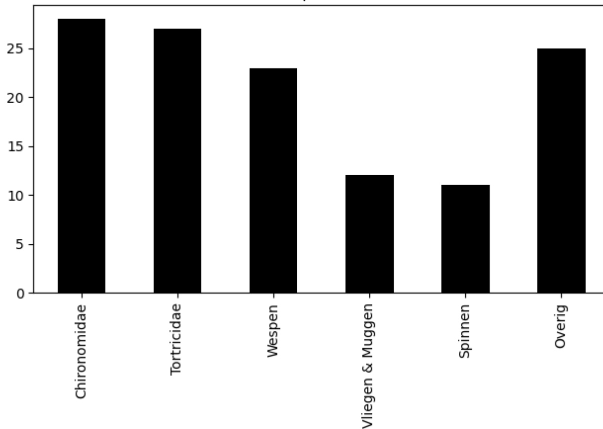
Voorkomen van ordes op 2020-06-12 (totaal = 126)
