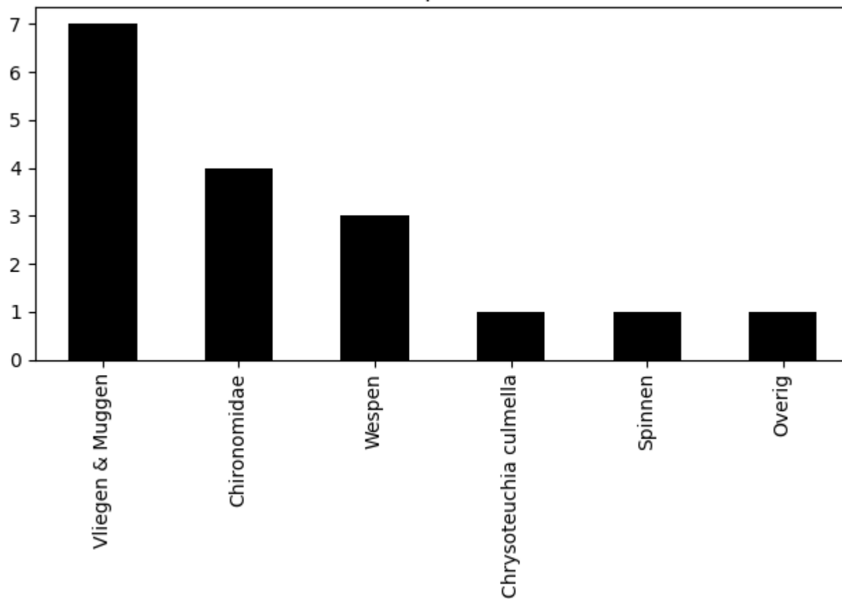
Voorkomen van ordes op 2020-07-04 (totaal = 17)
