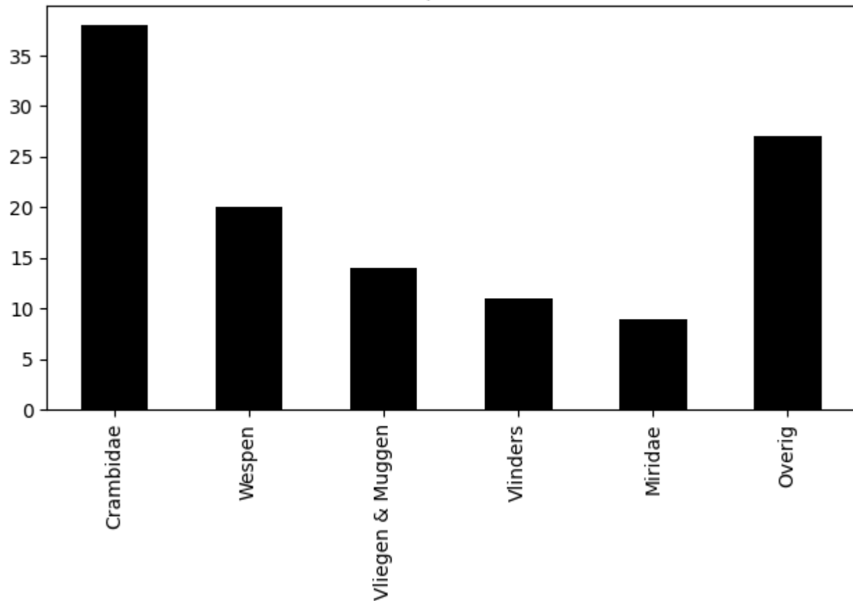
Voorkomen van ordes op 2020-07-07 (totaal = 119)
