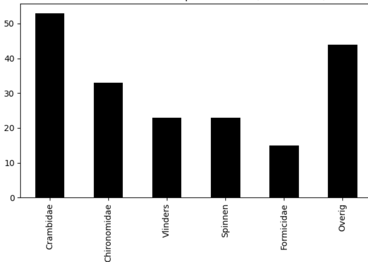
Voorkomen van ordes op 2020-06-16 (totaal = 191)
