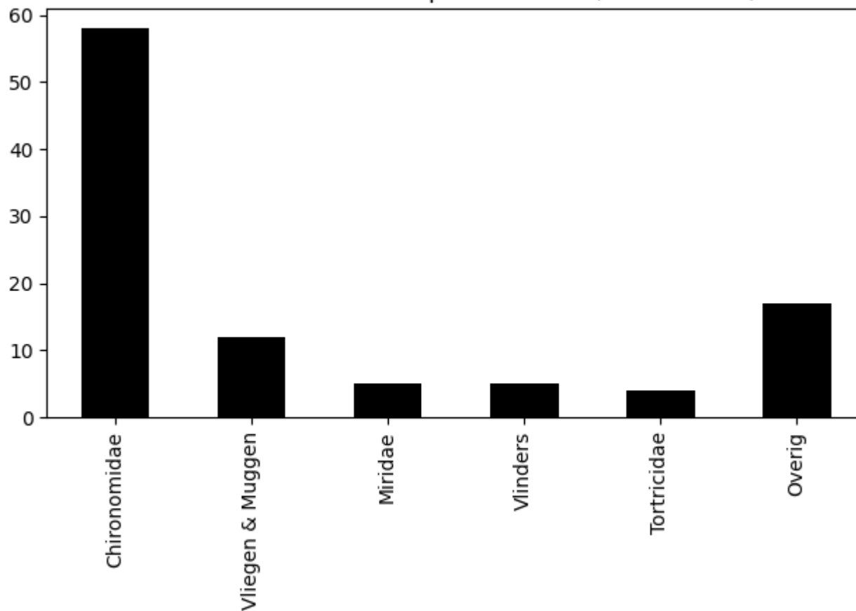
Voorkomen van ordes op 2020-07-23 (totaal = 101)
