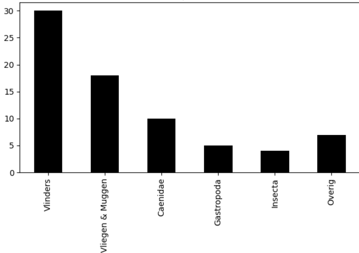
Voorkomen van ordes op 2020-07-11 (totaal = 74)
