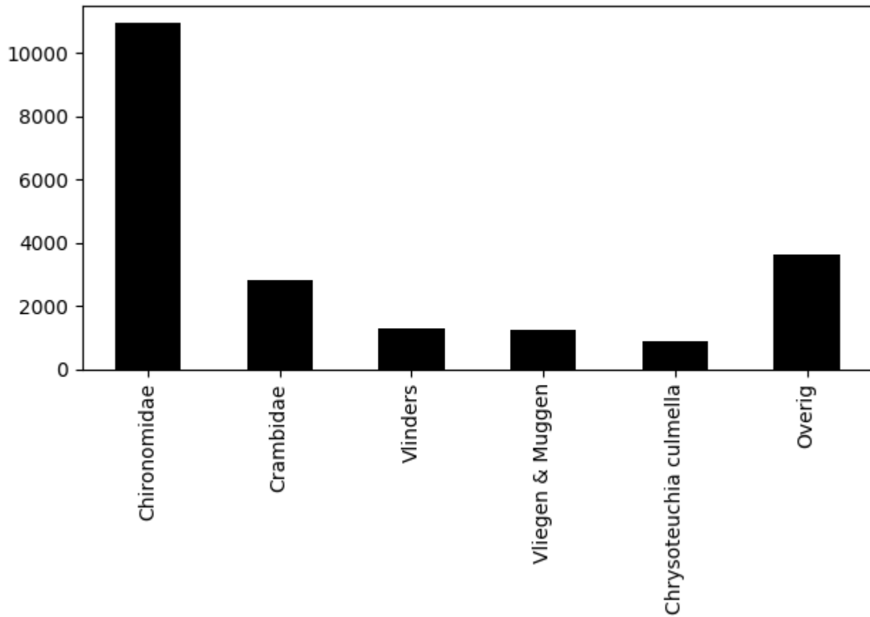
Voorkomen van ordes (totaal = 20791)
