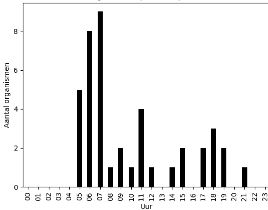
Aantal organismen per uur op 2020-07-07
