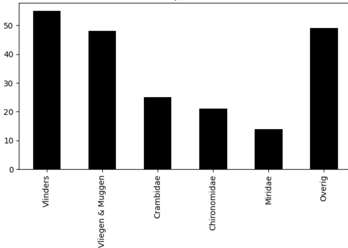
Voorkomen van ordes op 2020-06-28 (totaal = 212)
