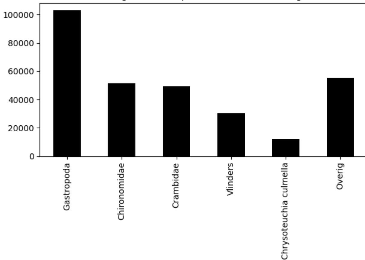
Verdeling biomassa per orde (totaal = 301 gram)
