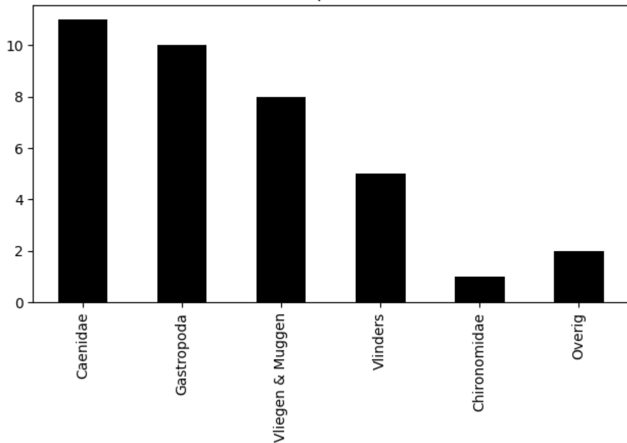
Voorkomen van ordes op 2020-07-22 (totaal = 37)
