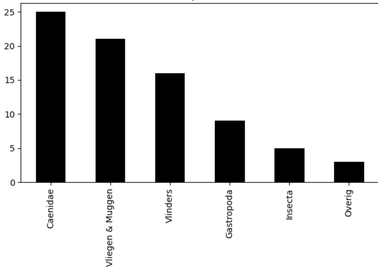
Voorkomen van ordes op 2020-07-12 (totaal = 79)
