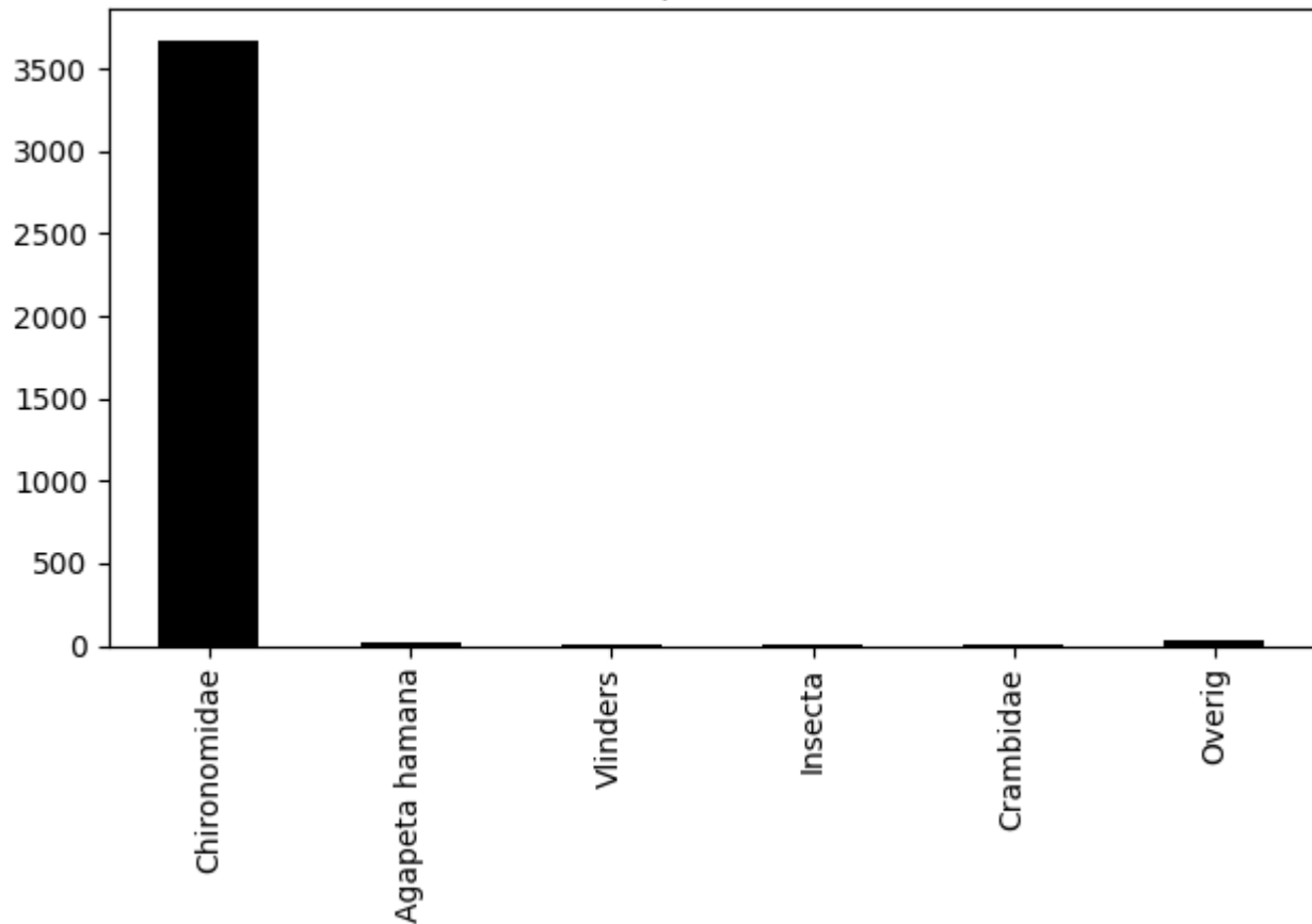
Voorkomen van ordes op 2020-08-01 (totaal = 3749)
