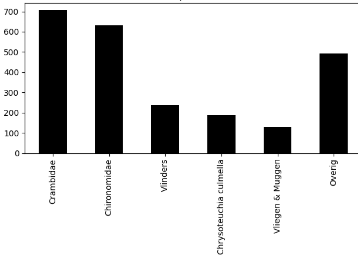
Voorkomen van ordes op 2020-06-27 (totaal = 2383)
