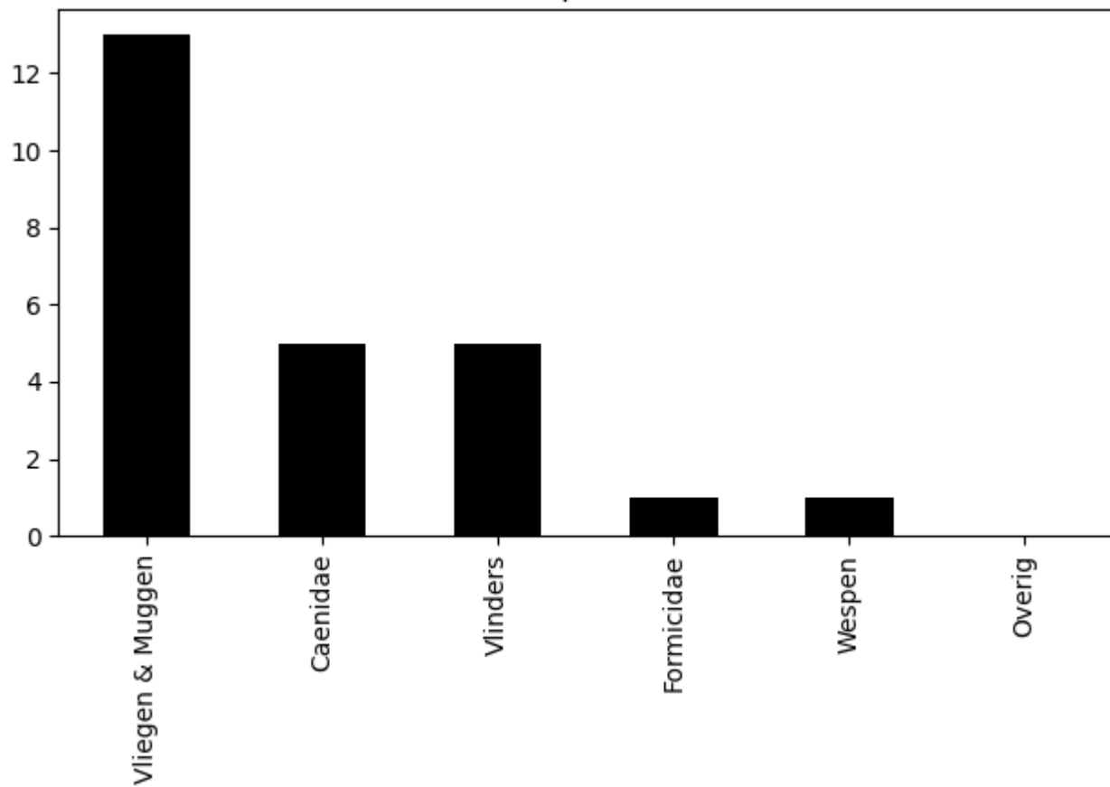
Voorkomen van ordes op 2020-07-15 (totaal = 25)
