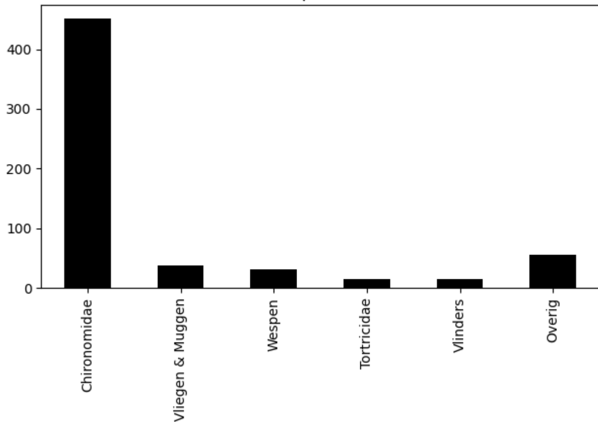
Voorkomen van ordes op 2020-07-26 (totaal = 605)
