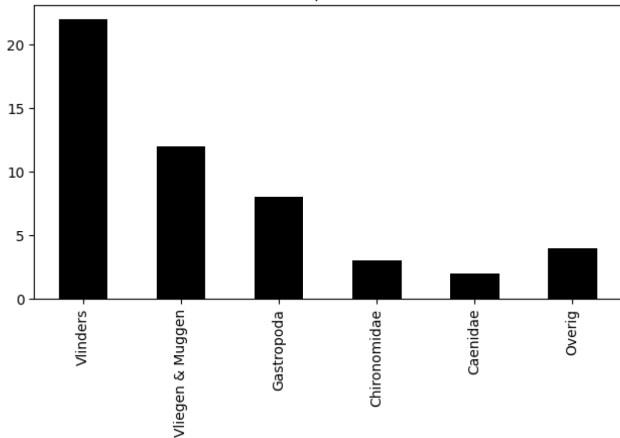
Voorkomen van ordes op 2020-07-05 (totaal = 51)
