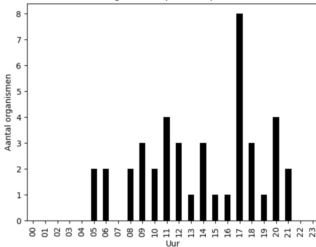
Aantal organismen per uur op 2020-07-19
