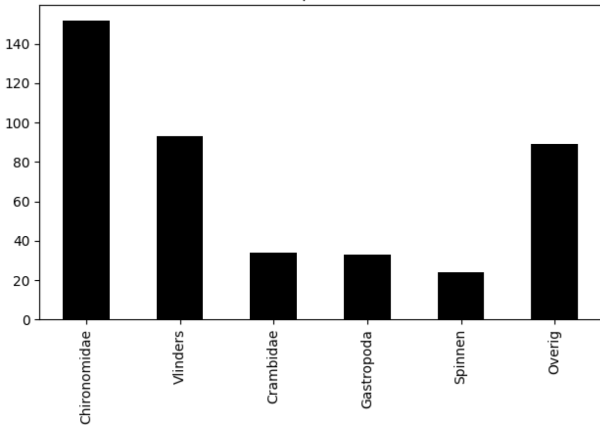
Voorkomen van ordes op 2020-07-29 (totaal = 425)
