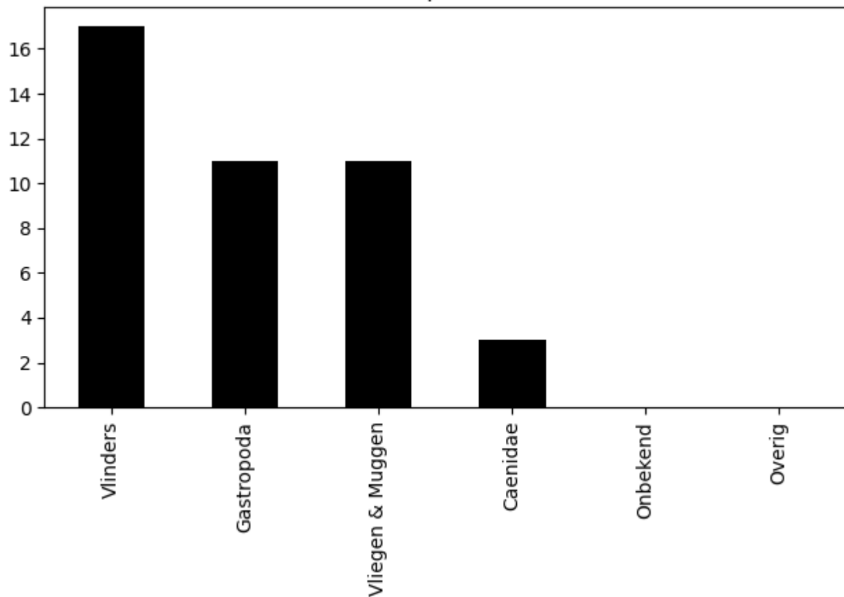
Voorkomen van ordes op 2020-07-07 (totaal = 42)
