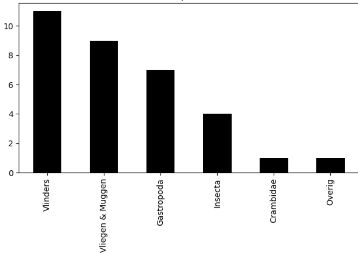
Voorkomen van ordes op 2020-07-21 (totaal = 33)
