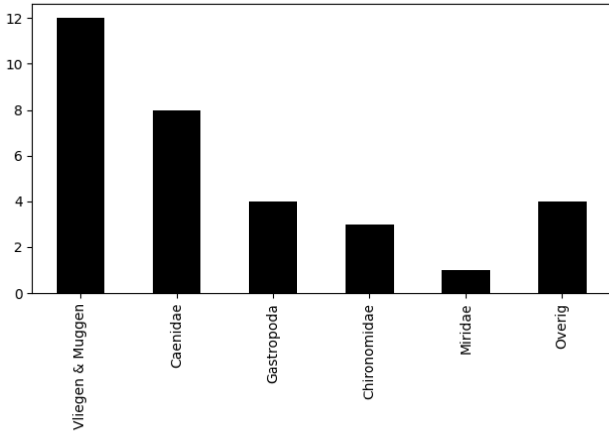
Voorkomen van ordes op 2020-07-17 (totaal = 32)
