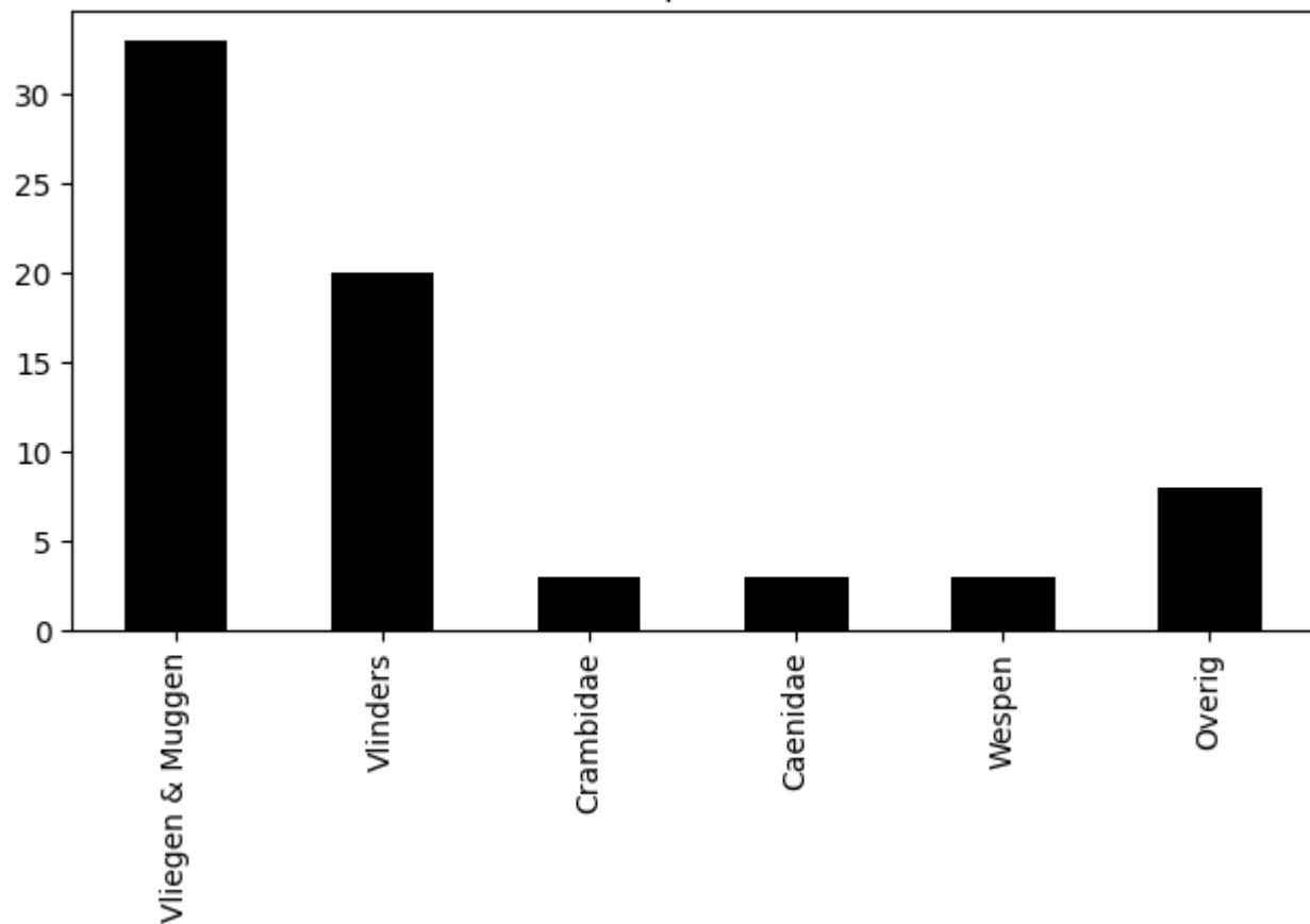
Voorkomen van ordes op 2020-07-10 (totaal = 70)
