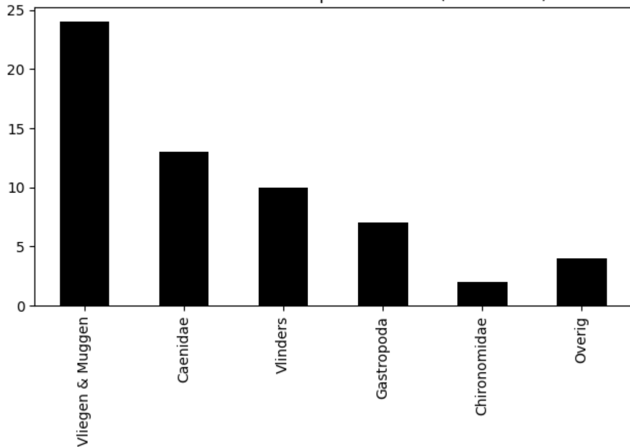
Voorkomen van ordes op 2020-07-08 (totaal = 60)
