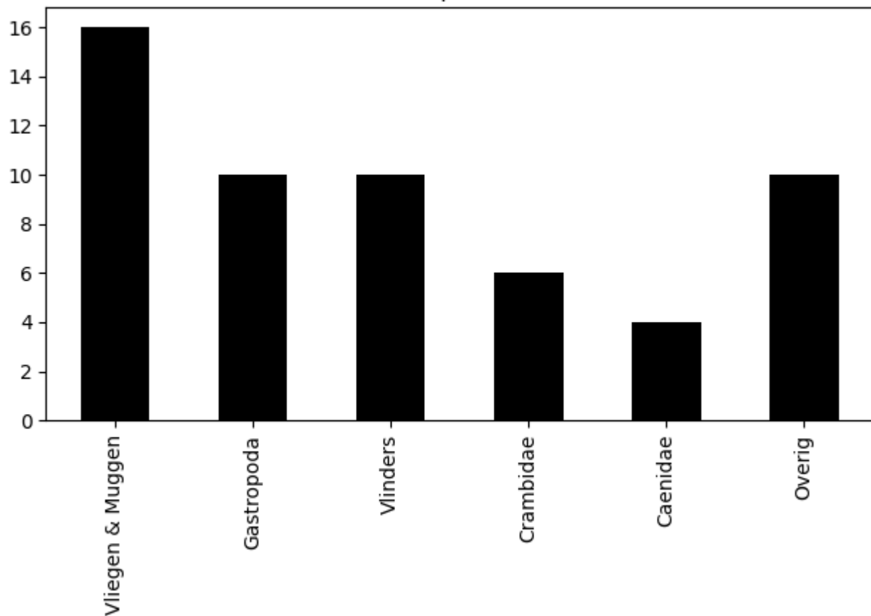
Voorkomen van ordes op 2020-07-16 (totaal = 56)
