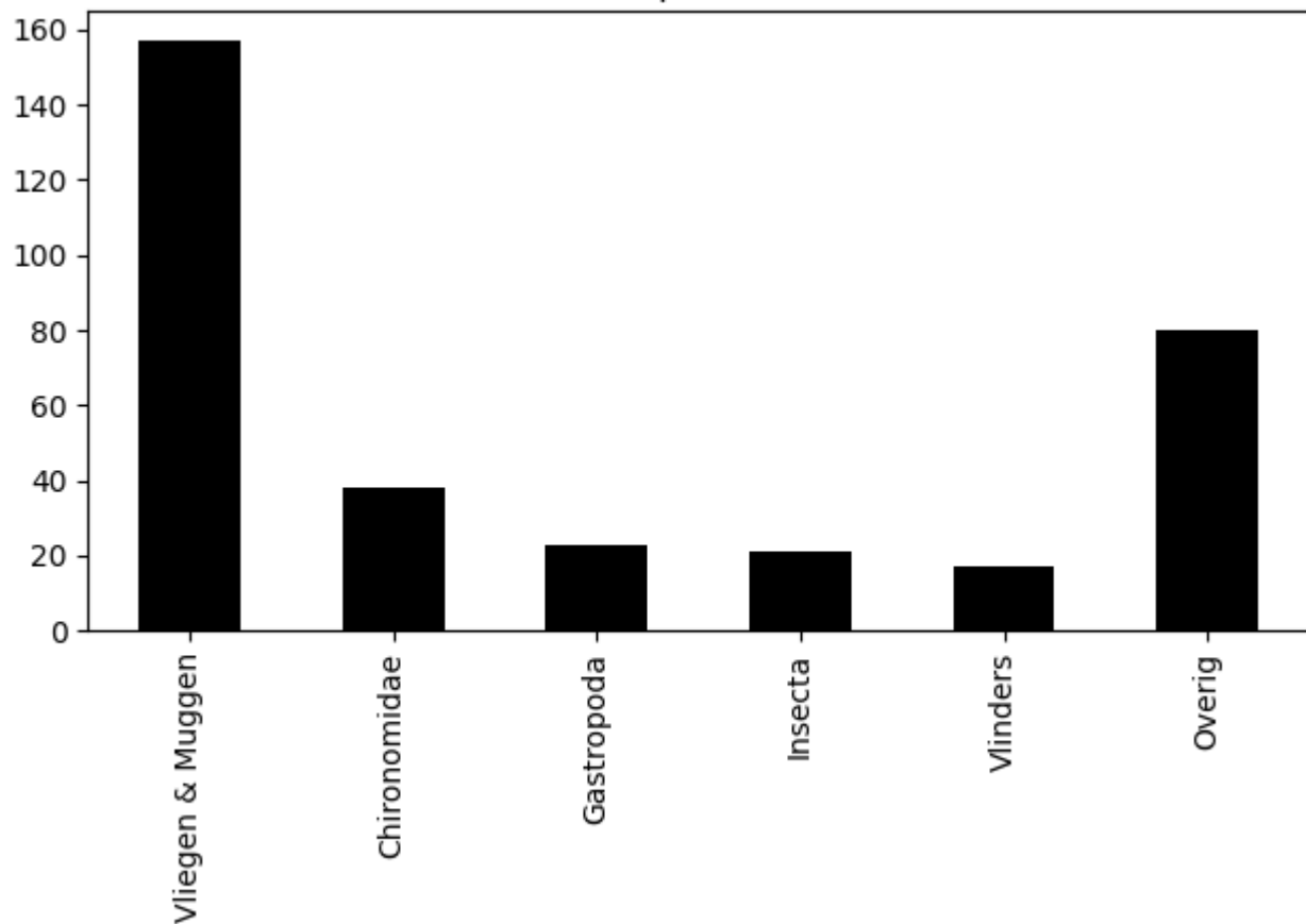
Voorkomen van ordes op 2020-06-30 (totaal = 336)
