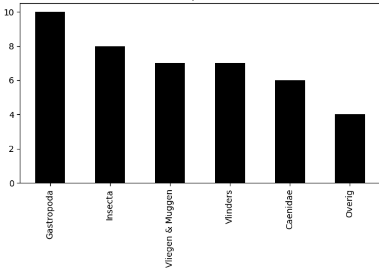
Voorkomen van ordes op 2020-07-13 (totaal = 42)
