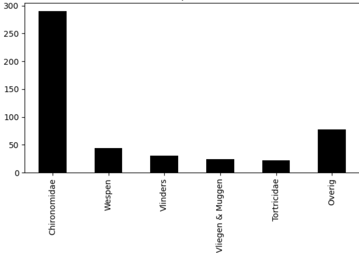
Voorkomen van ordes op 2020-07-28 (totaal = 489)
