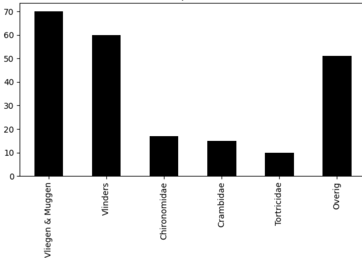
Voorkomen van ordes op 2020-06-29 (totaal = 223)
