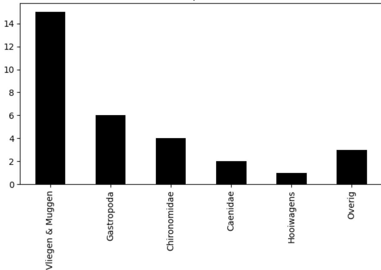
Voorkomen van ordes op 2020-07-04 (totaal = 31)
