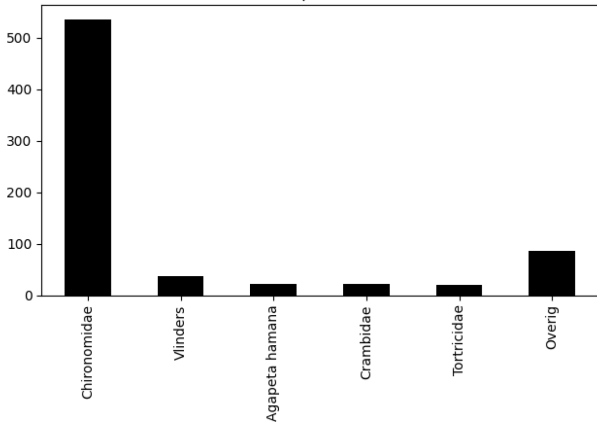
Voorkomen van ordes op 2020-07-25 (totaal = 719)
