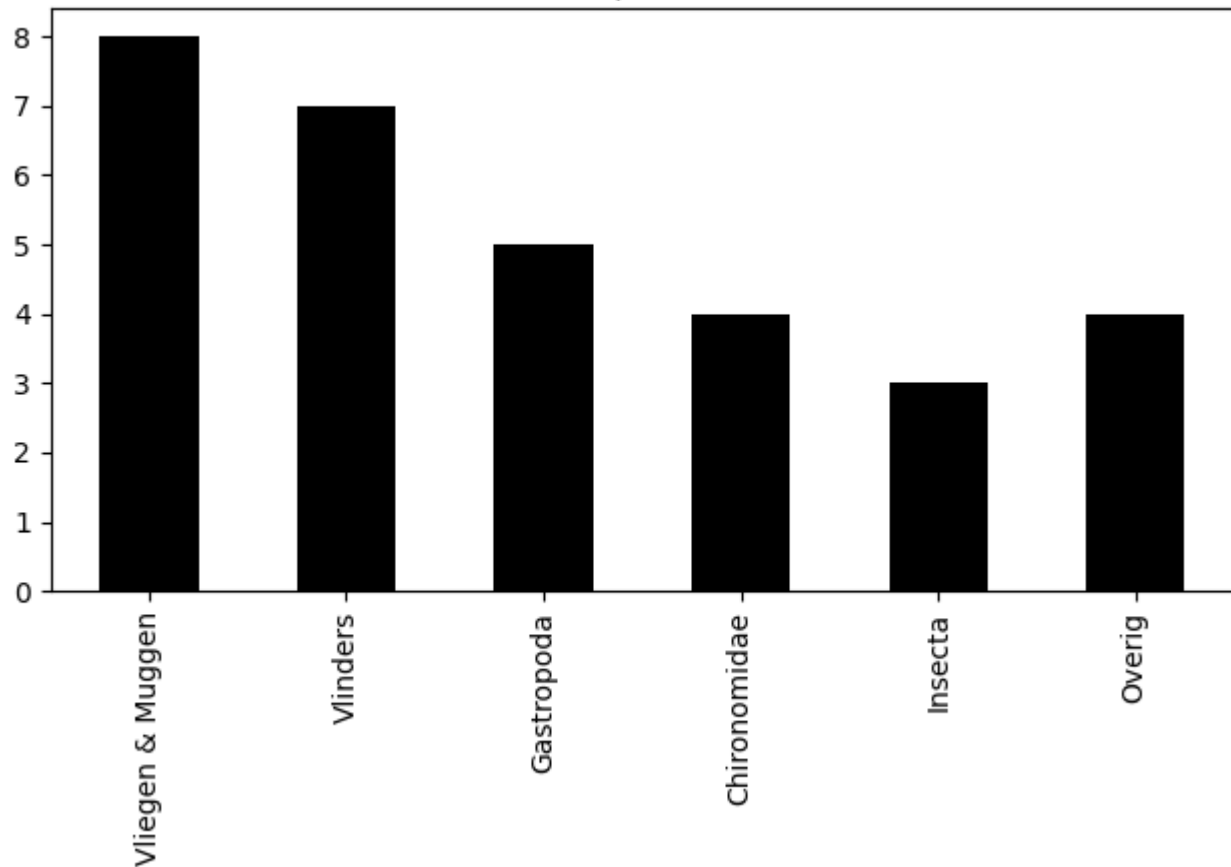
Voorkomen van ordes op 2020-07-20 (totaal = 31)
