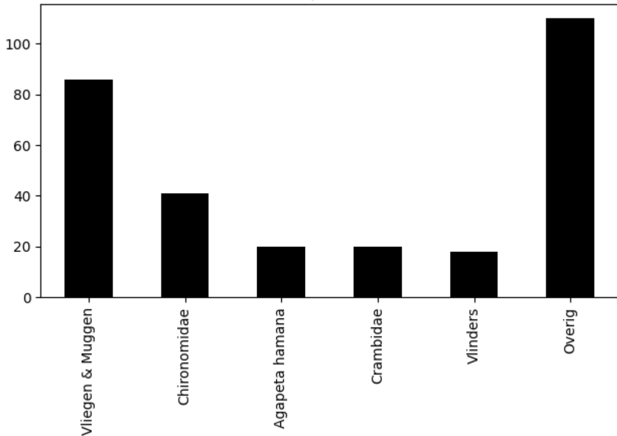
Voorkomen van ordes op 2020-07-01 (totaal = 295)
