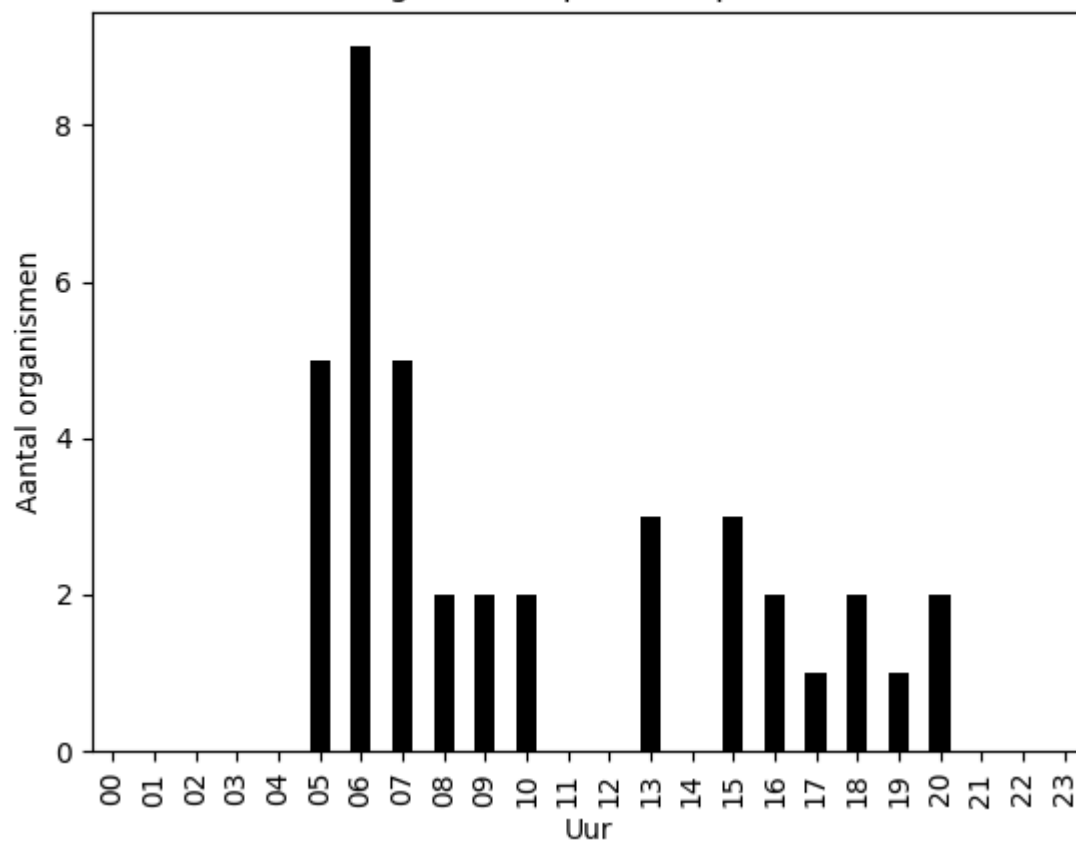
Aantal organismen per uur op 2020-07-18
