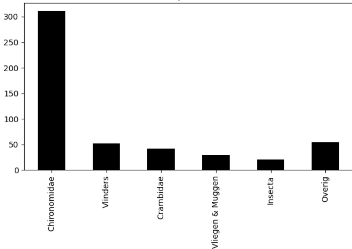
Voorkomen van ordes op 2020-07-27 (totaal = 508)
