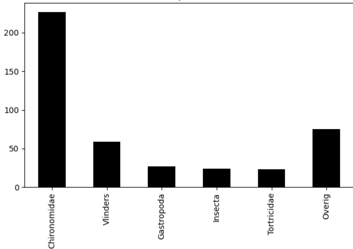
Voorkomen van ordes op 2020-07-30 (totaal = 435)
