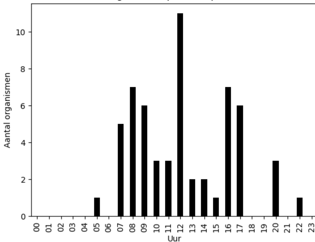
Aantal organismen per uur op 2020-07-06
