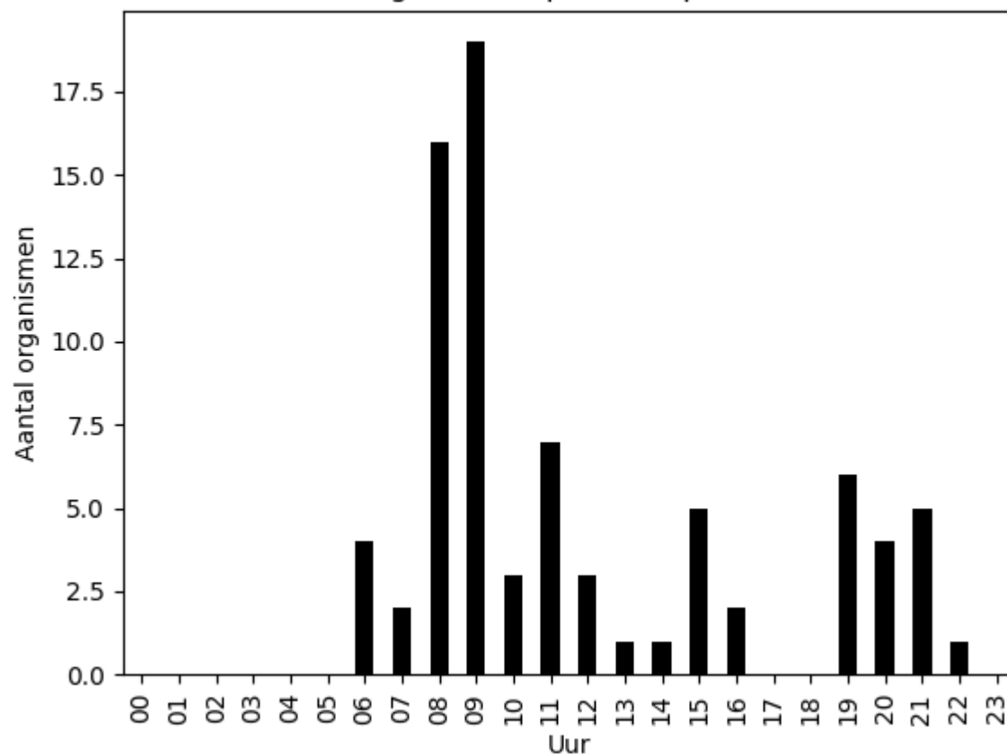
Aantal organismen per uur op 2020-07-12
