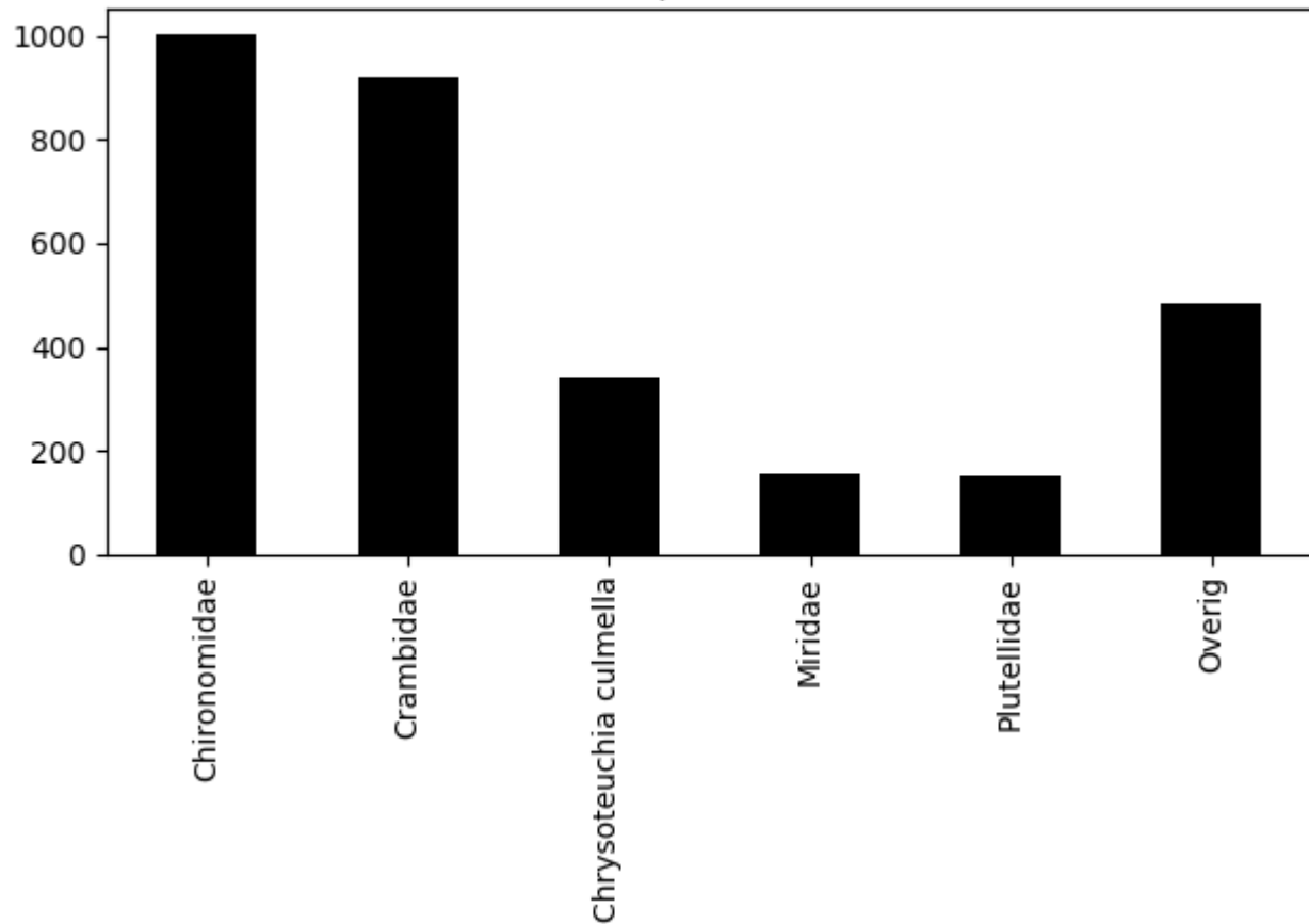
Voorkomen van ordes op 2020-06-26 (totaal = 3051)
