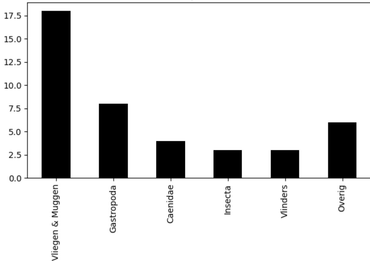
Voorkomen van ordes op 2020-07-19 (totaal = 42)
