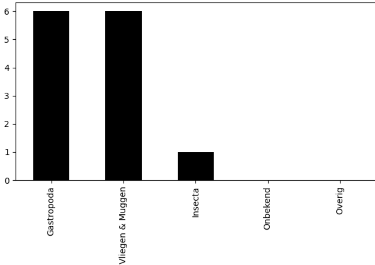
Voorkomen van ordes op 2020-07-14 (totaal = 13)
