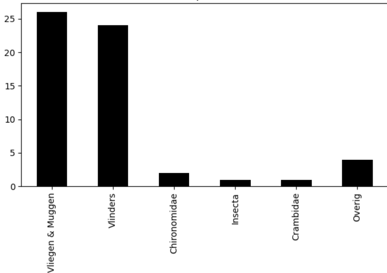
Voorkomen van ordes op 2020-07-06 (totaal = 58)
