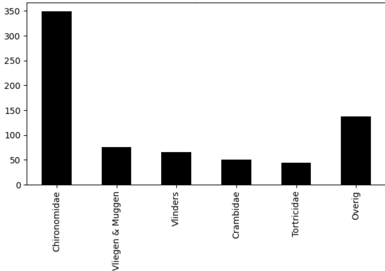
Voorkomen van ordes op 2020-07-24 (totaal = 722)
