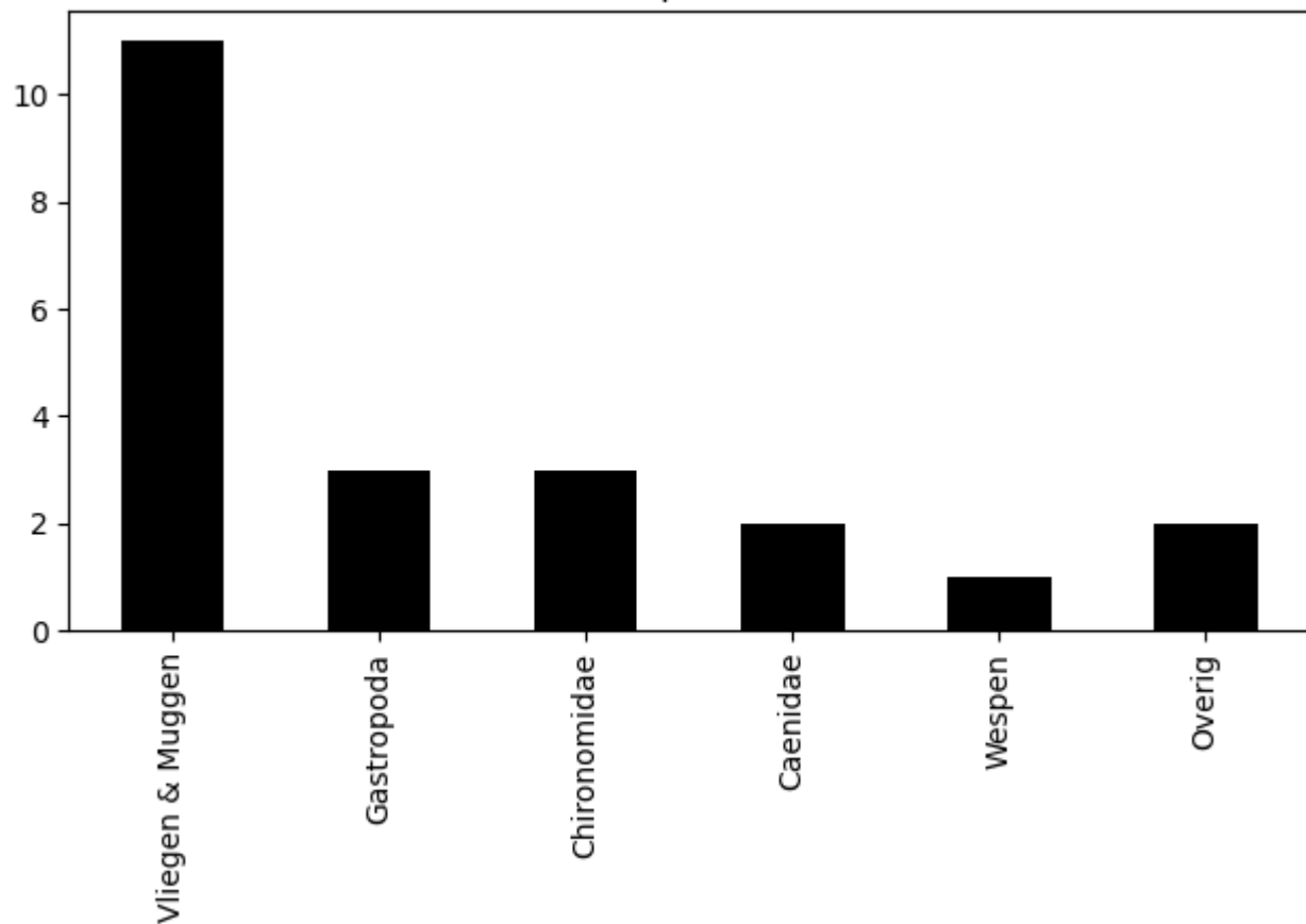
Voorkomen van ordes op 2020-07-09 (totaal = 22)
