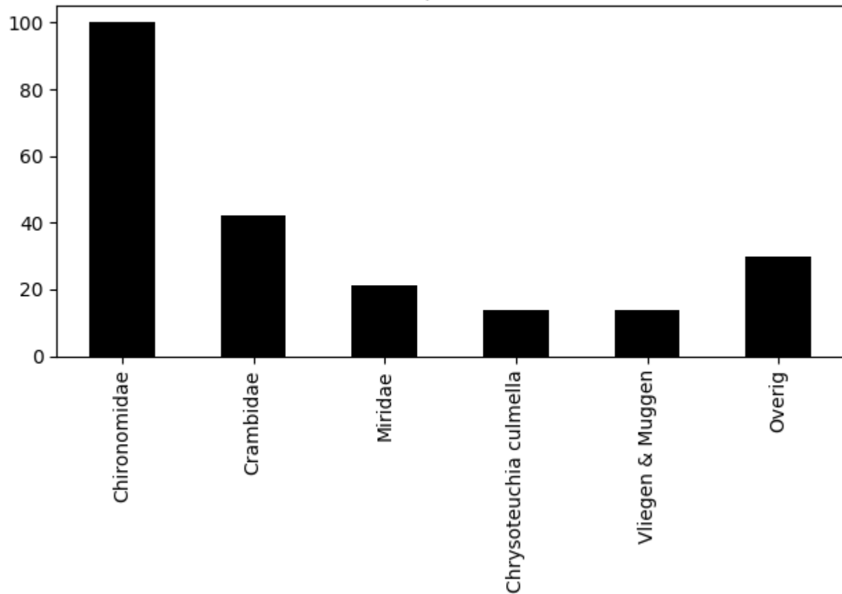
Voorkomen van ordes op 2020-06-24 (totaal = 221)
