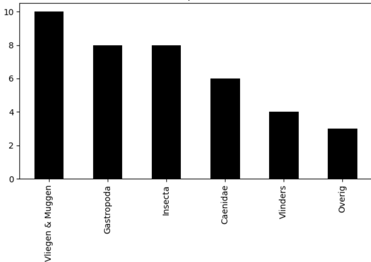
Voorkomen van ordes op 2020-07-18 (totaal = 39)
