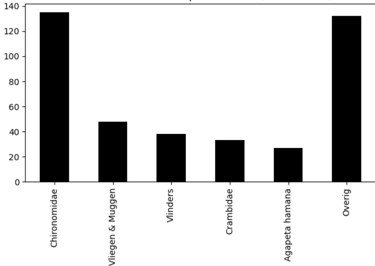
Voorkomen van ordes op 2020-07-02 (totaal = 413)
