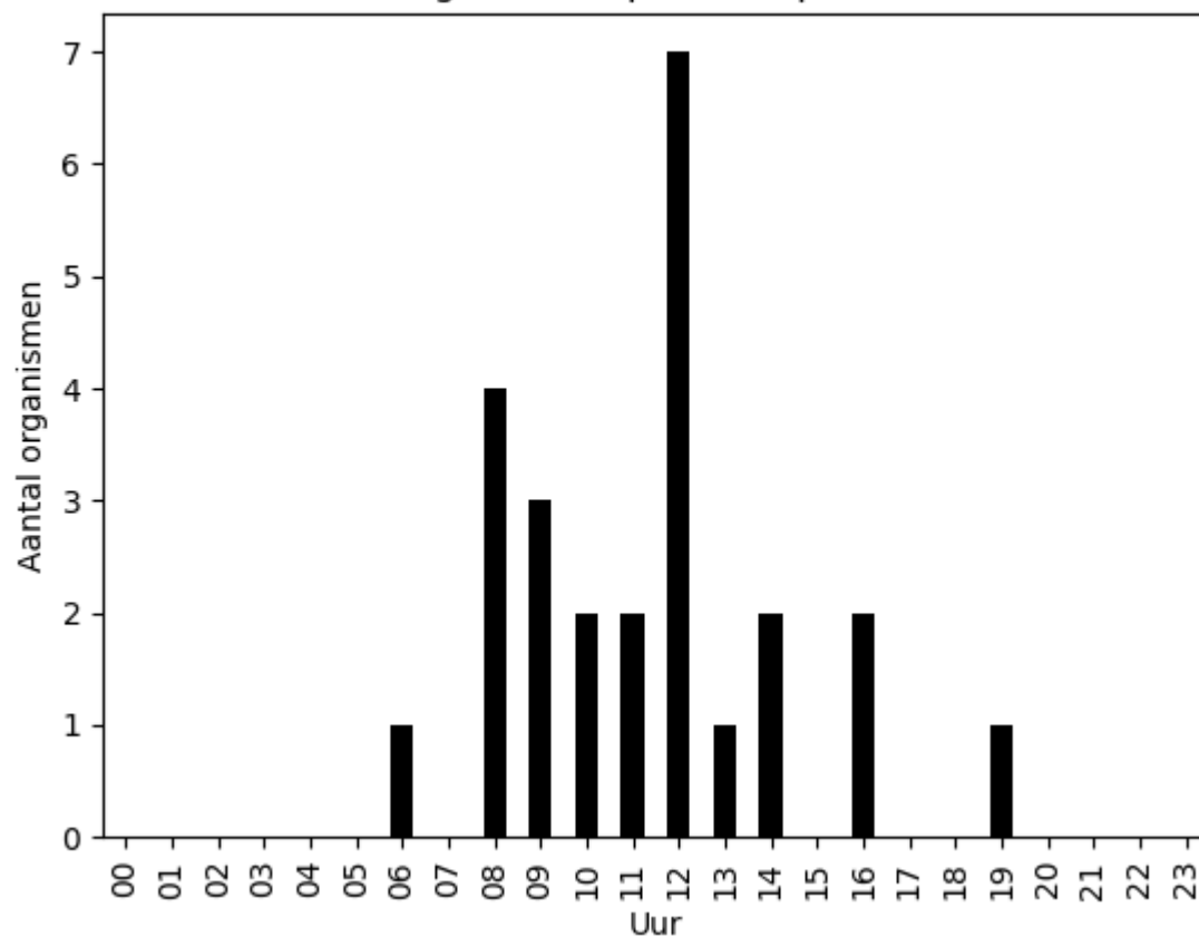
Aantal organismen per uur op 2020-07-15
