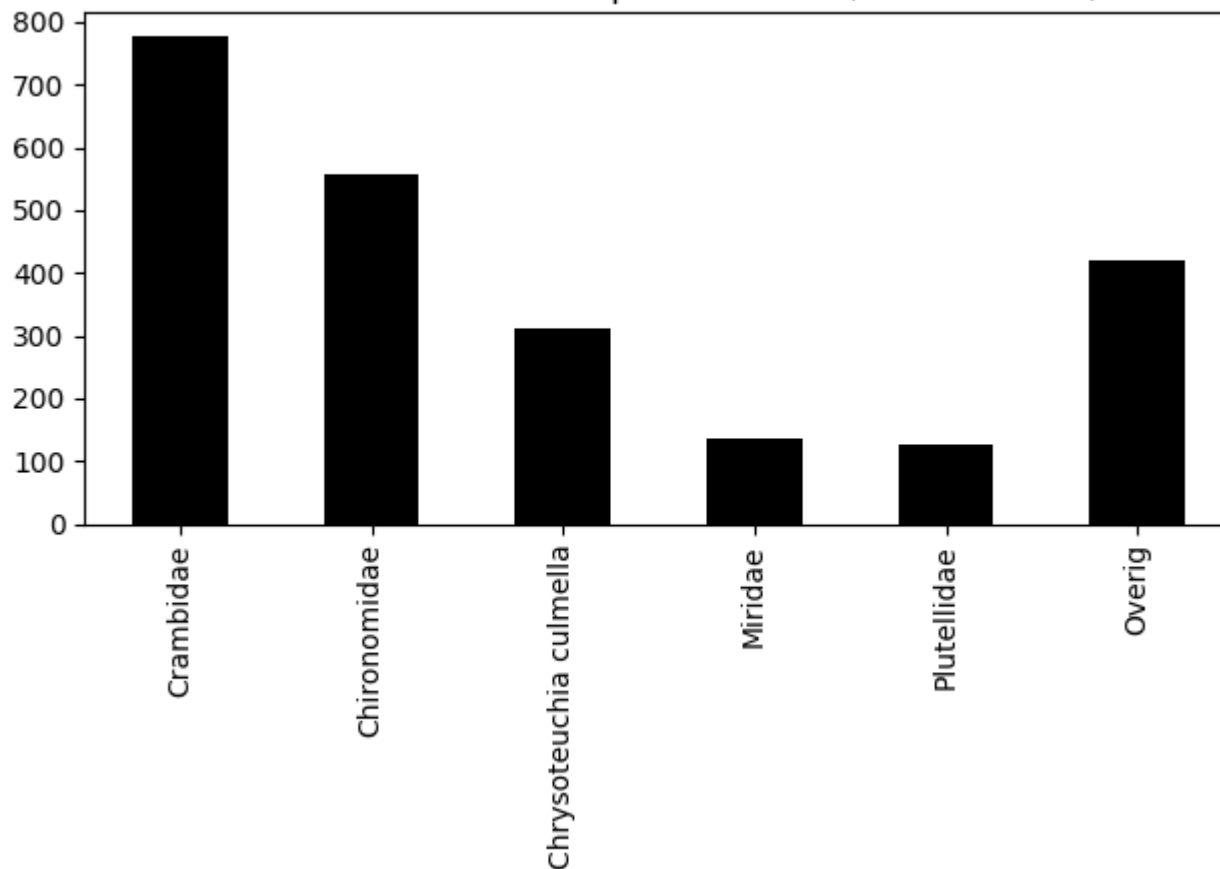
Voorkomen van ordes op 2020-06-25 (totaal = 2324)
