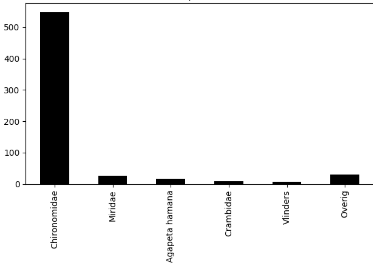
Voorkomen van ordes op 2020-07-03 (totaal = 637)
