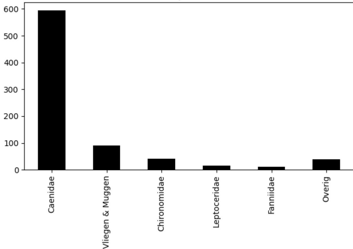
Voorkomen van ordes op 2020-06-05 (totaal = 792)
