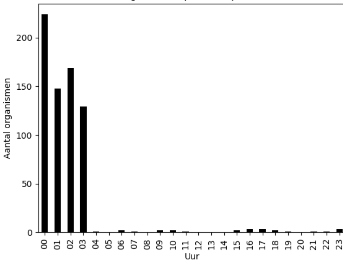
Aantal organismen per uur op 2020-06-18
