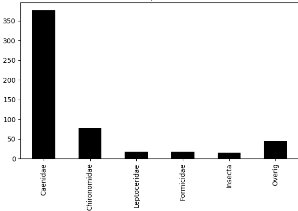
Voorkomen van ordes op 2020-08-07 (totaal = 550)
