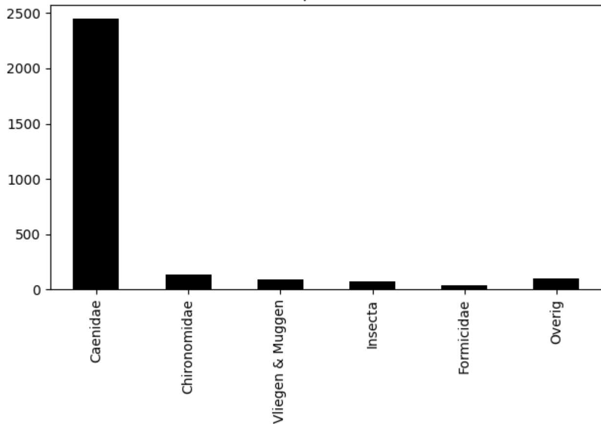
Voorkomen van ordes op 2020-06-10 (totaal = 2889)
