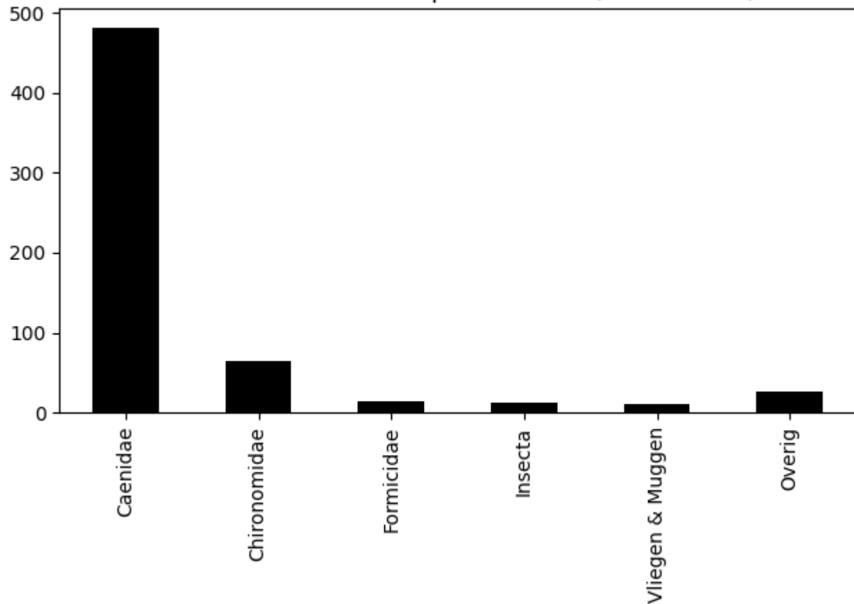
Voorkomen van ordes op 2020-08-06 (totaal = 610)
