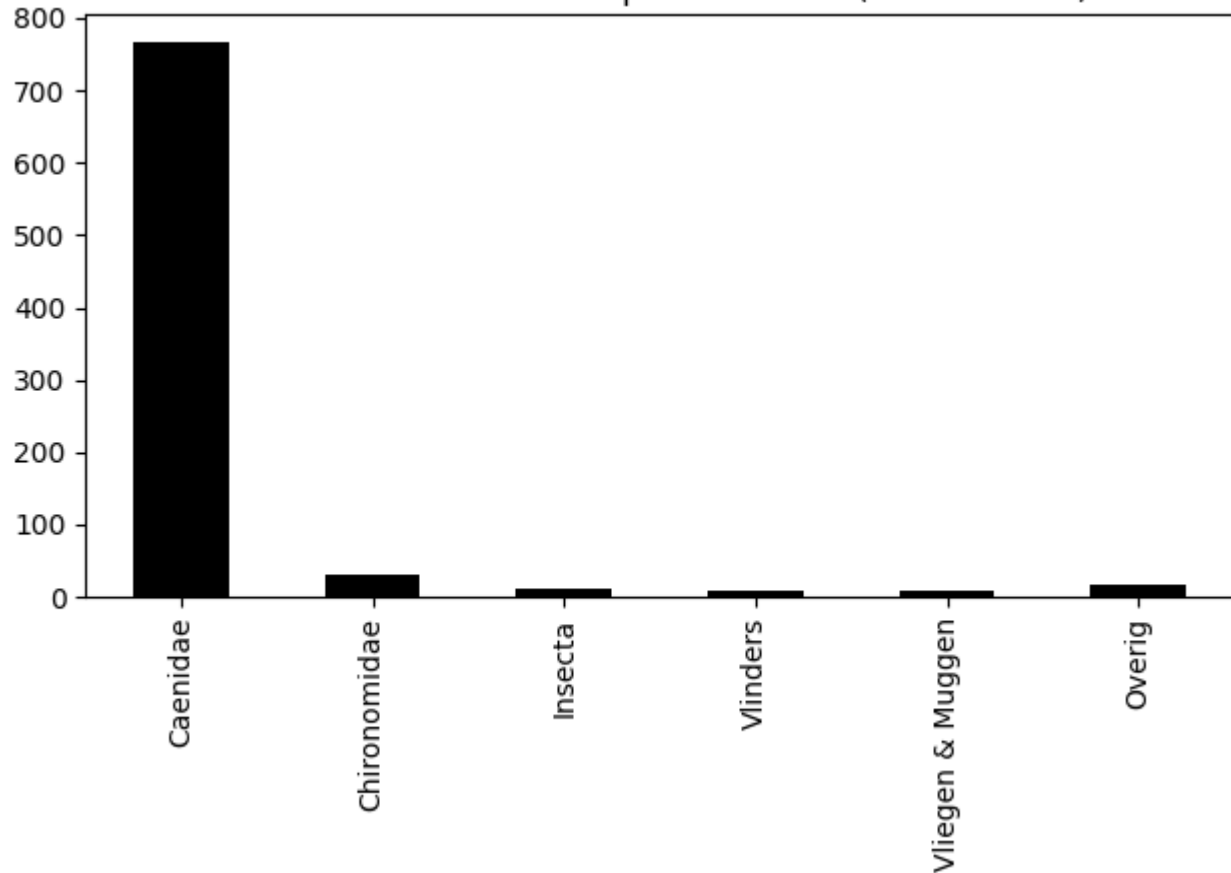
Voorkomen van ordes op 2020-08-05 (totaal = 845)
