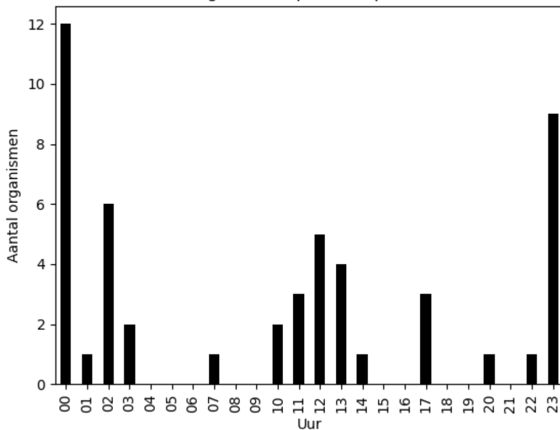
Aantal organismen per uur op 2020-06-16
