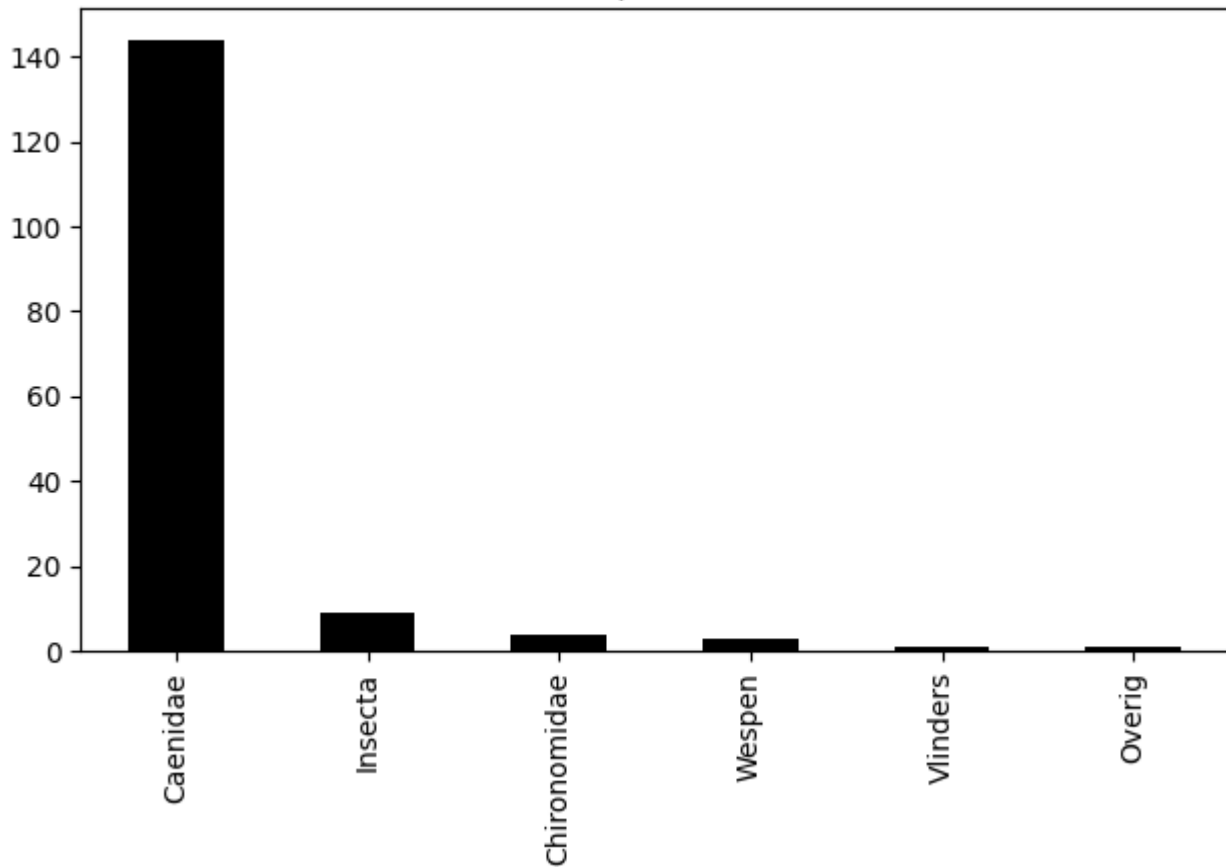
Voorkomen van ordes op 2020-06-21 (totaal = 162)
