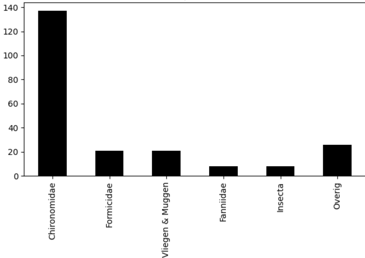
Voorkomen van ordes op 2020-06-15 (totaal = 221)
