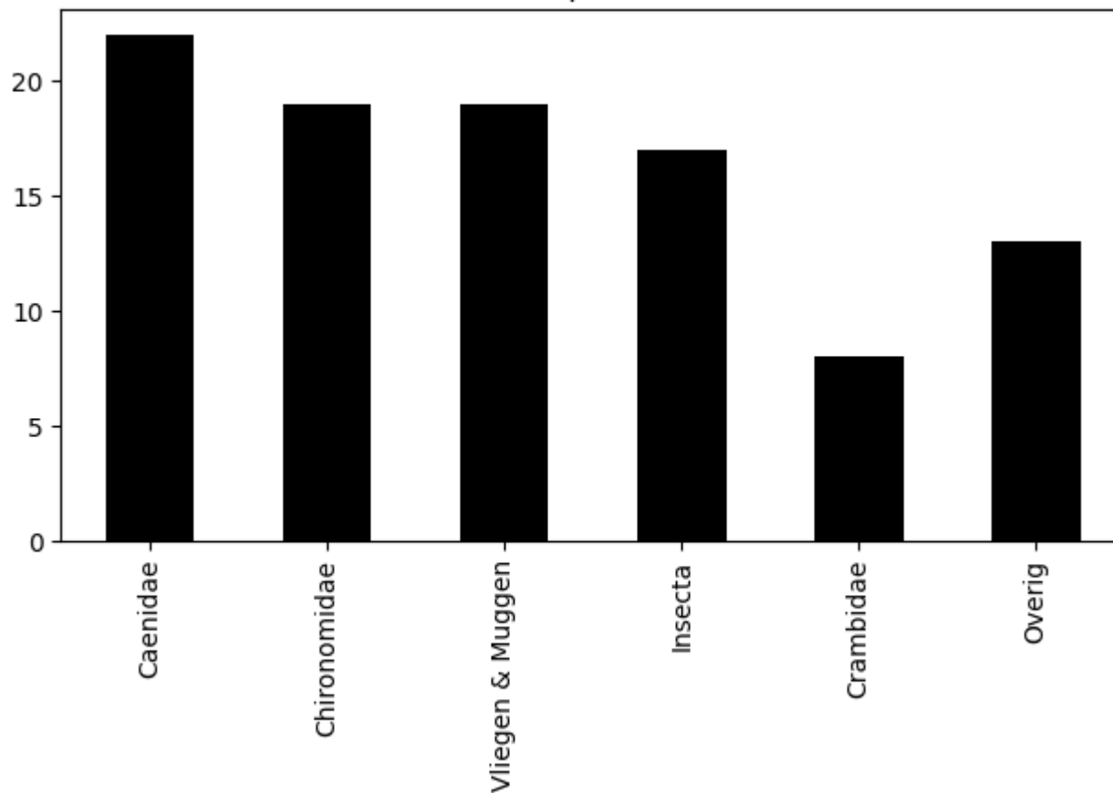
Voorkomen van ordes op 2020-06-12 (totaal = 98)
