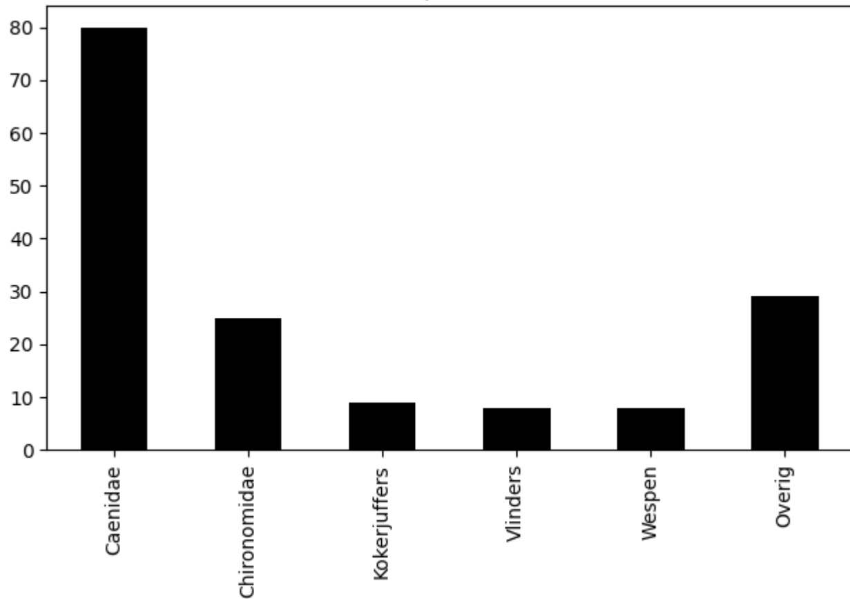
Voorkomen van ordes op 2020-08-08 (totaal = 159)
