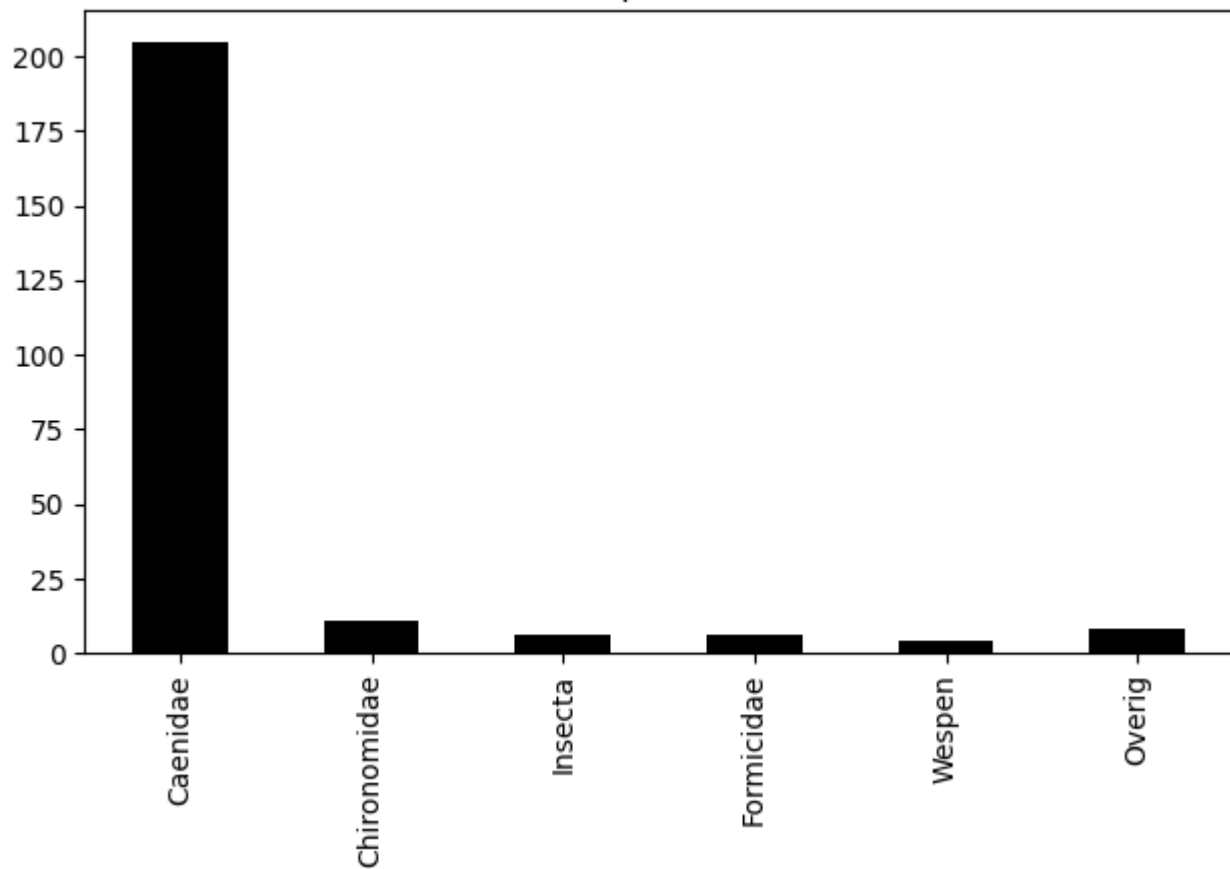
Voorkomen van ordes op 2020-06-19 (totaal = 240)
