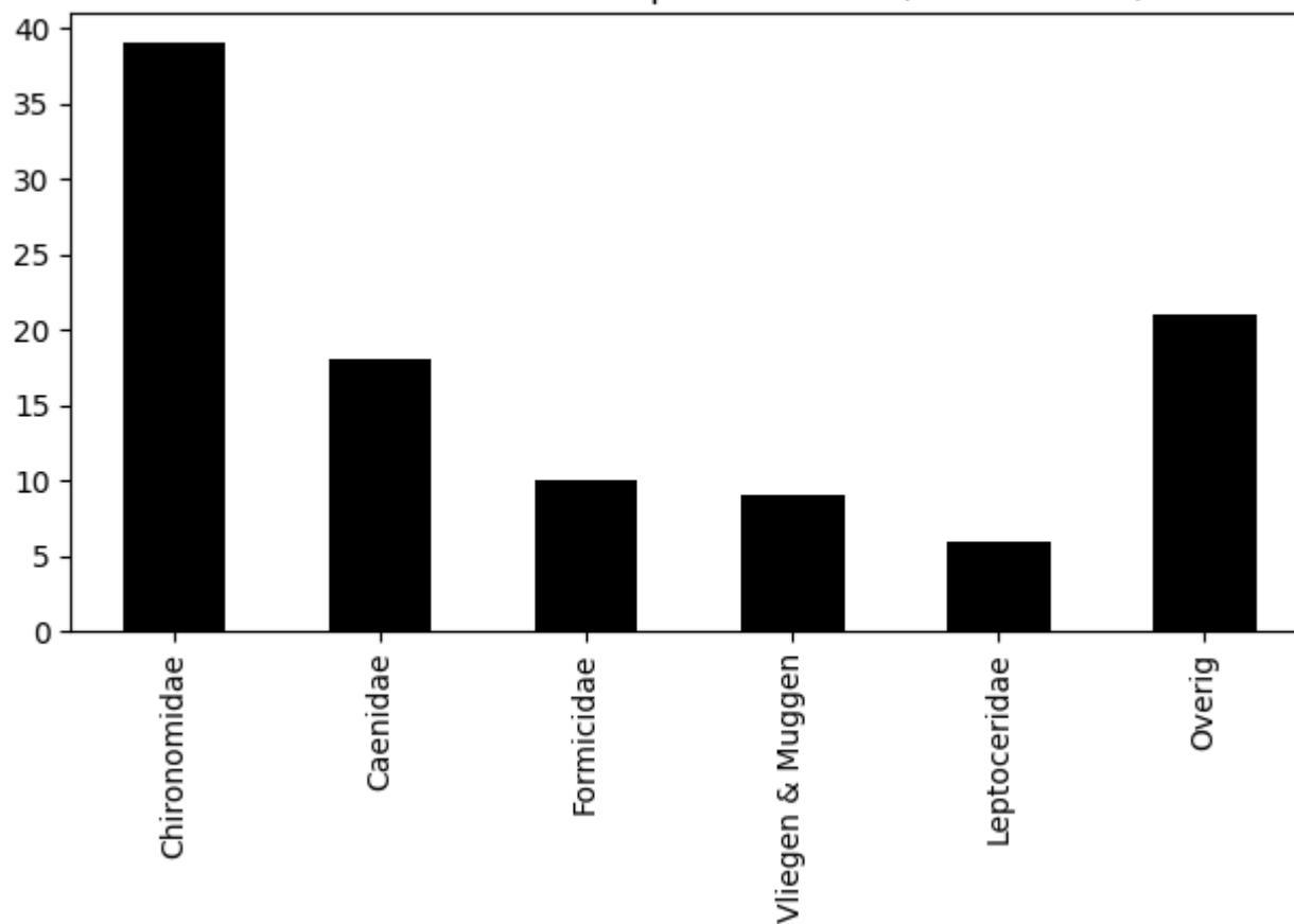
Voorkomen van ordes op 2020-06-17 (totaal = 103)
