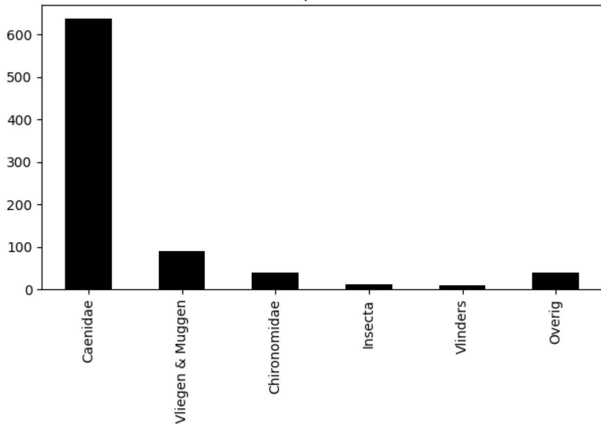
Voorkomen van ordes op 2020-06-04 (totaal = 830)
