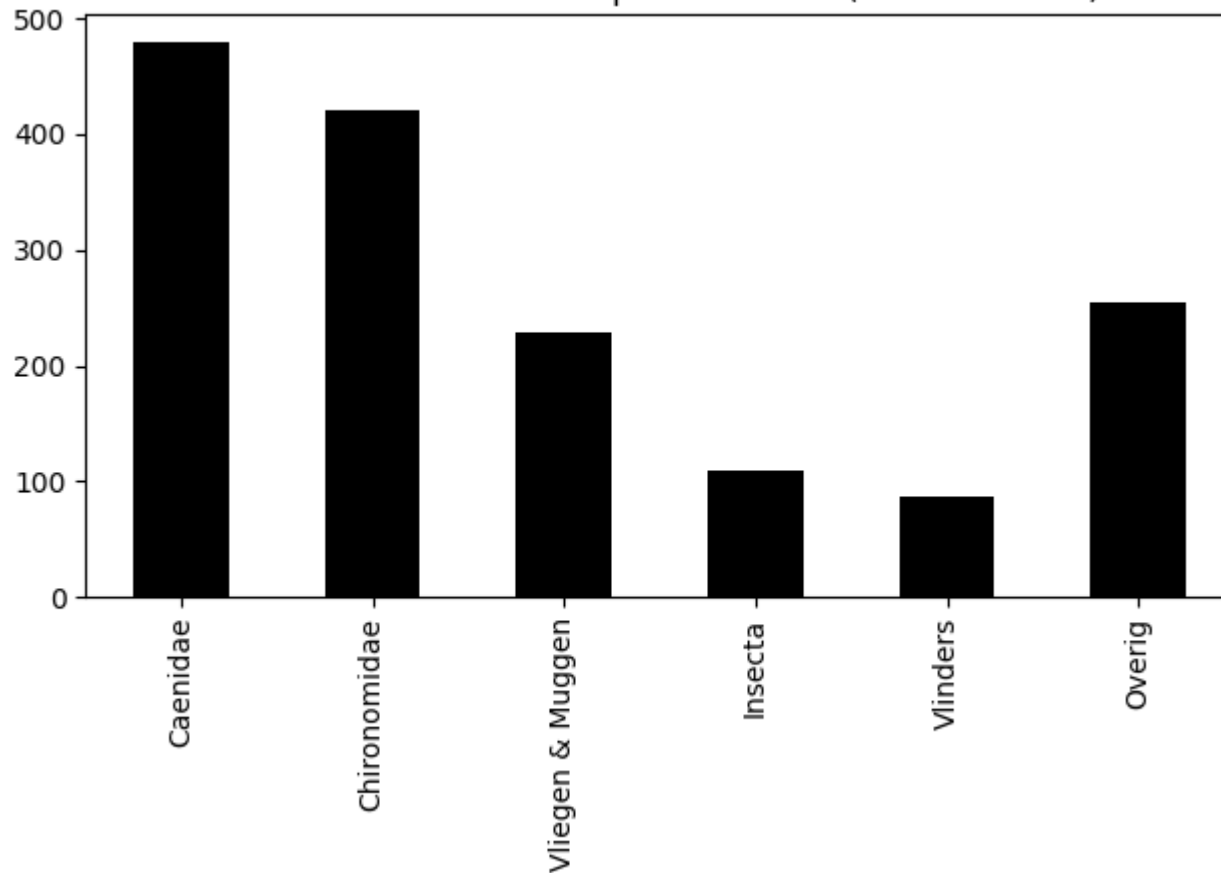
Voorkomen van ordes op 2020-06-06 (totaal = 1577)
