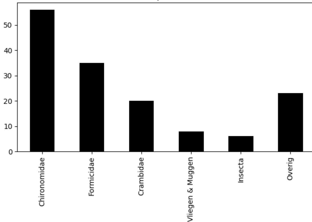
Voorkomen van ordes op 2020-06-14 (totaal = 148)
