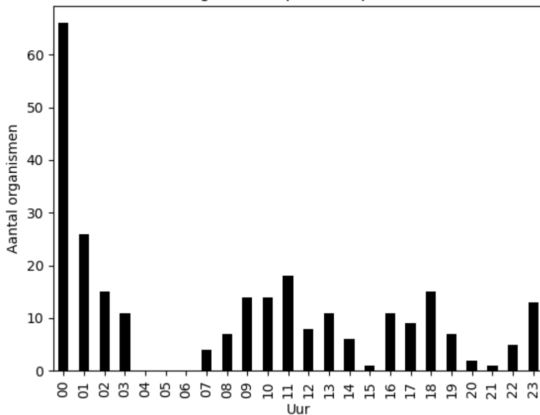
Aantal organismen per uur op 2020-06-13
