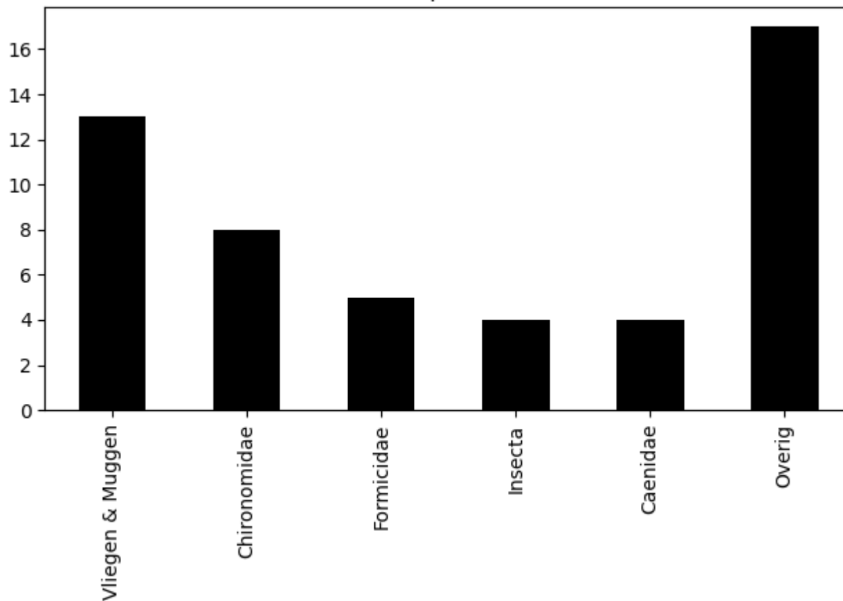
Voorkomen van ordes op 2020-06-16 (totaal = 51)
