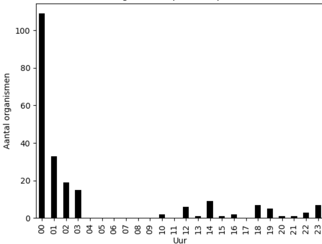
Aantal organismen per uur op 2020-06-15
