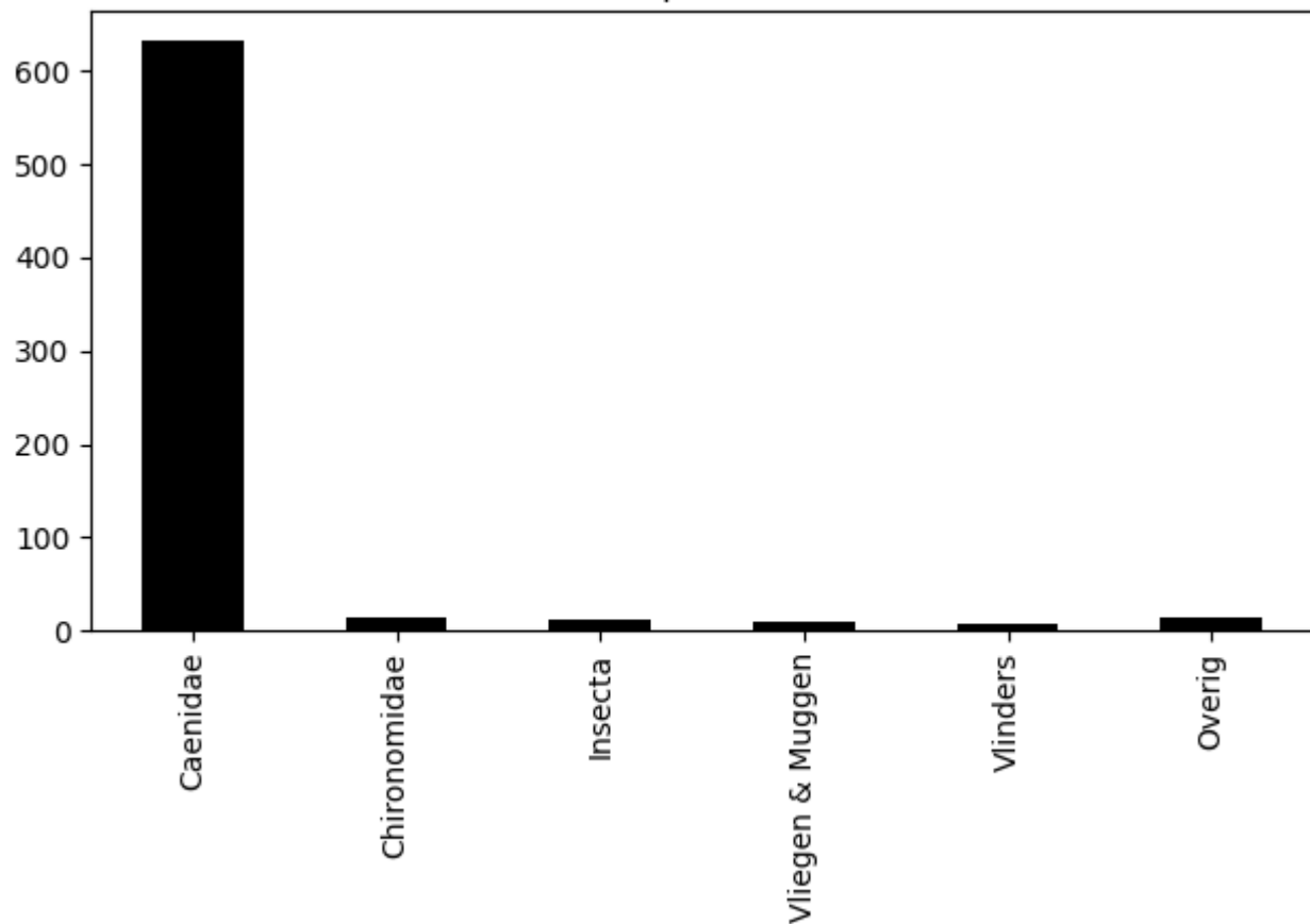
Voorkomen van ordes op 2020-08-04 (totaal = 687)
