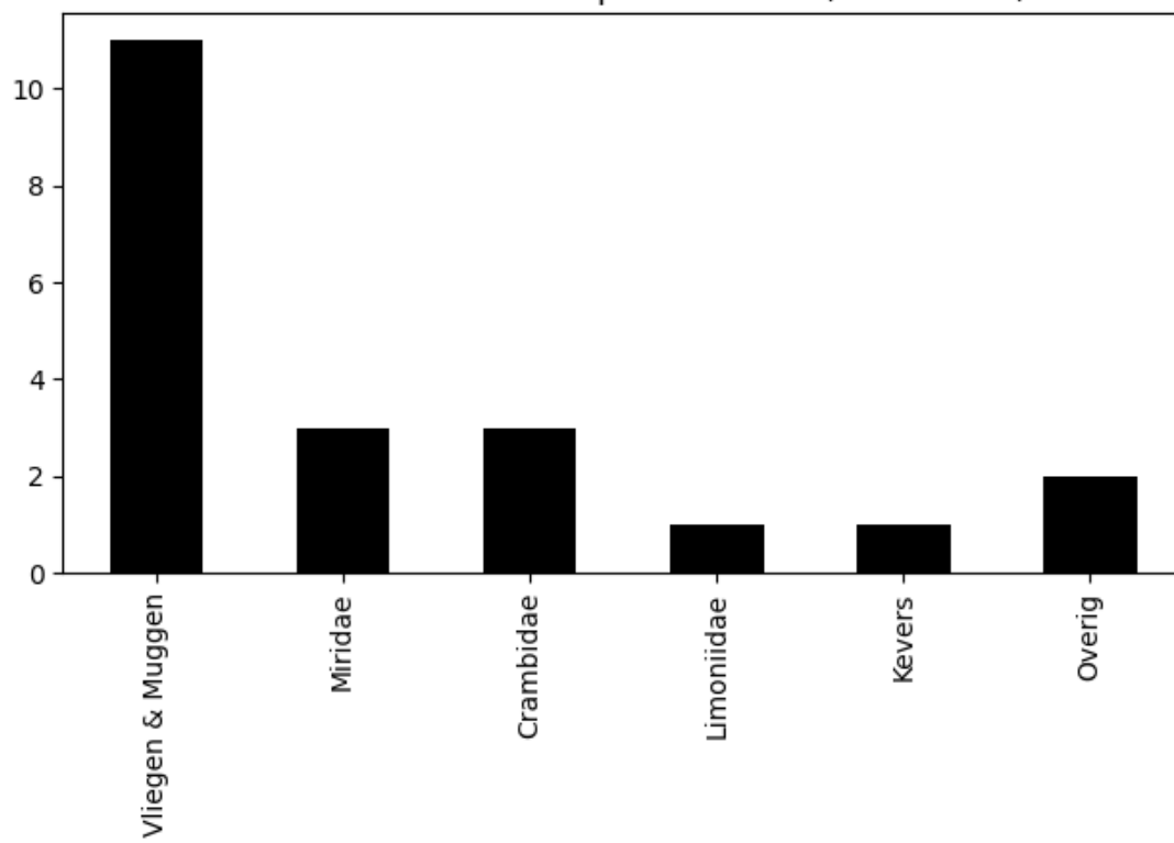
Voorkomen van ordes op 2022-07-16 (totaal = 21)
