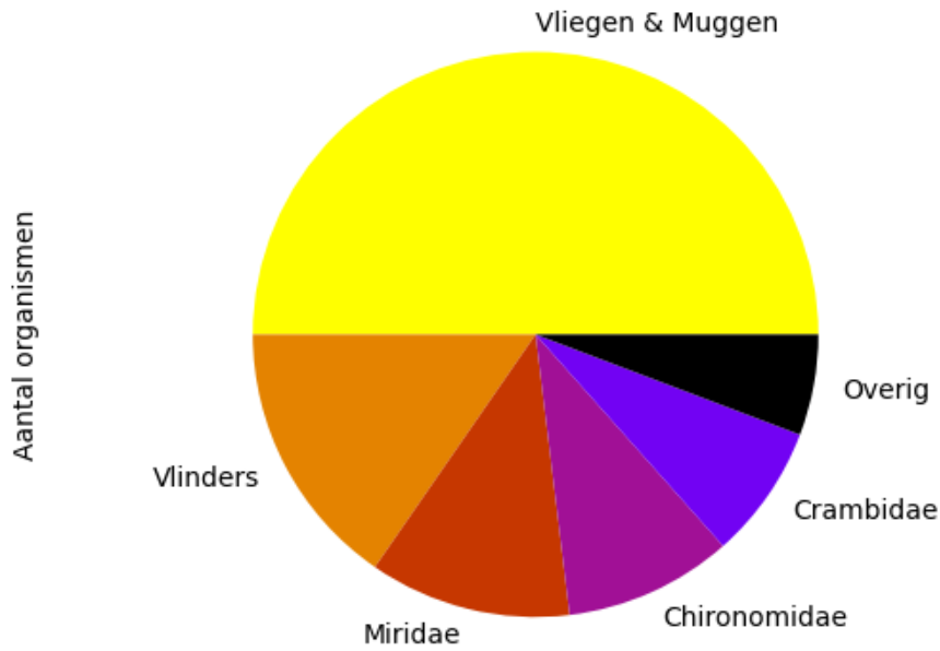
Voorkomen van ordes op 2022-07-22 (totaal = 52)
