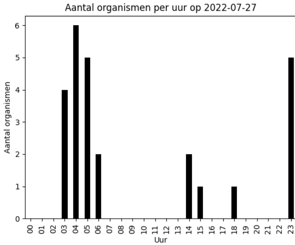
Voorkomen van ordes op 2022-07-27 (totaal = 26)
