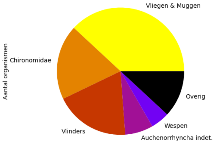
Voorkomen van ordes op 2022-06-23 (totaal = 42)
