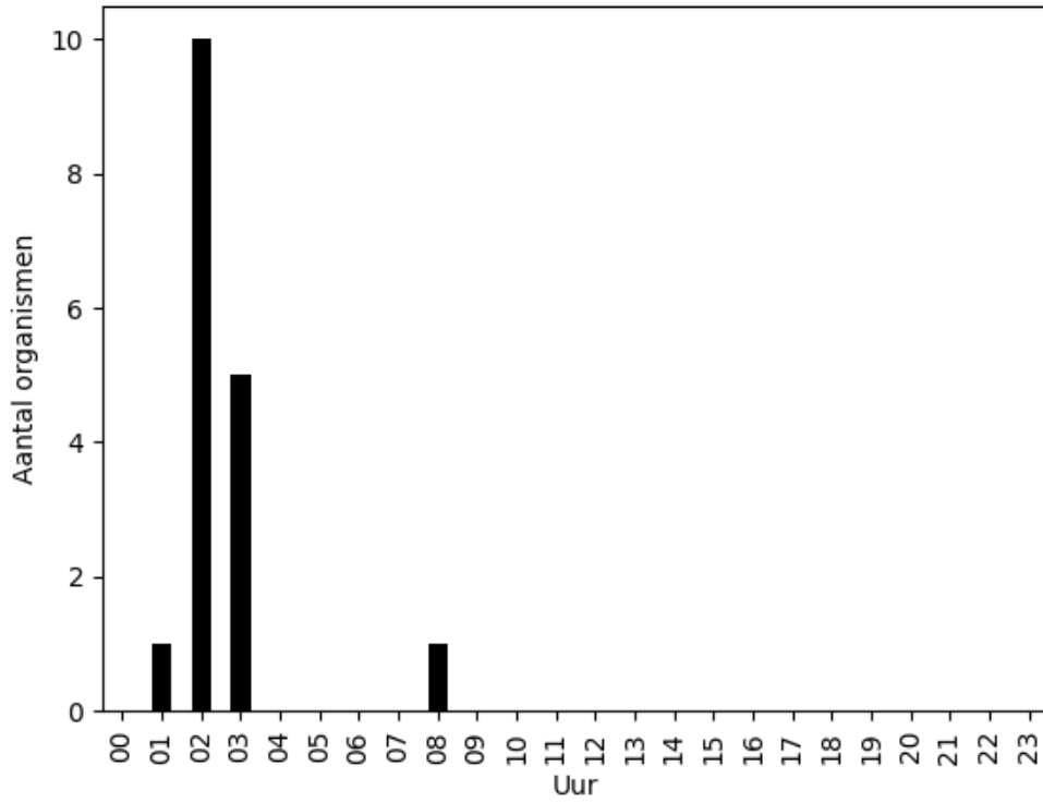
Aantal organismen per uur op 2022-07-01
