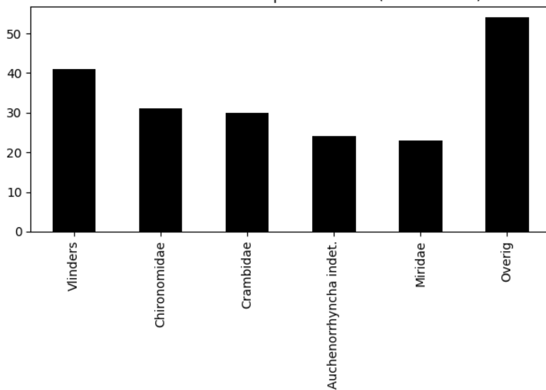
Voorkomen van ordes op 2022-07-25 (totaal = 203)
