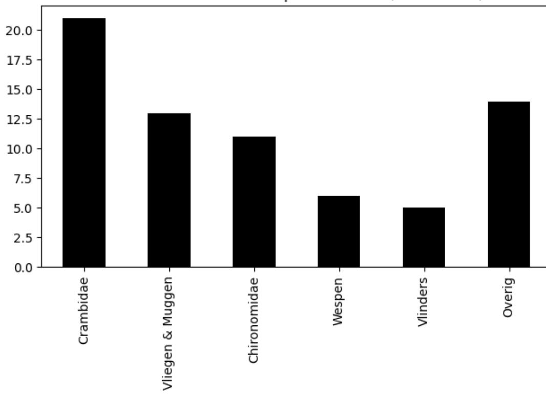
Voorkomen van ordes op 2022-07-14 (totaal = 70)
