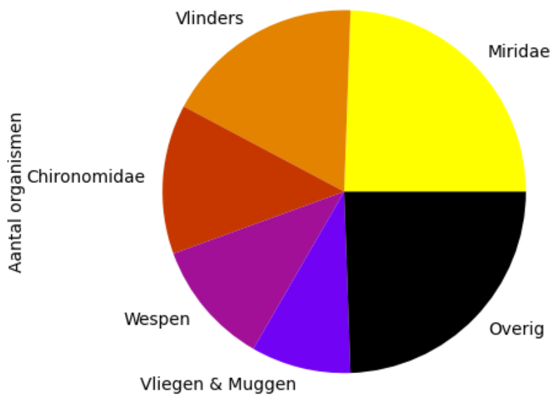
Voorkomen van ordes op 2022-07-21 (totaal = 45)
