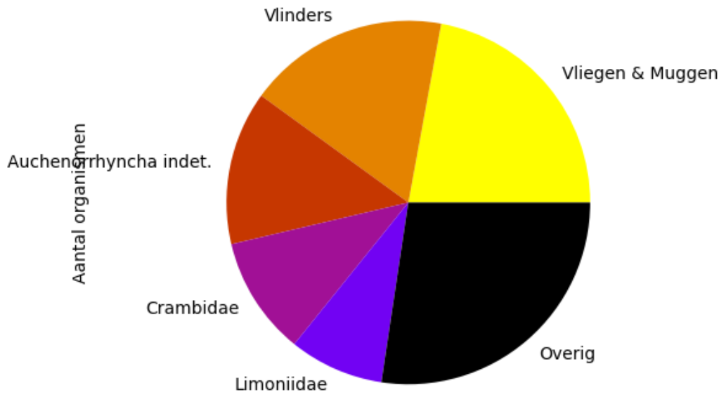
Voorkomen van ordes op 2022-07-24 (totaal = 95)
