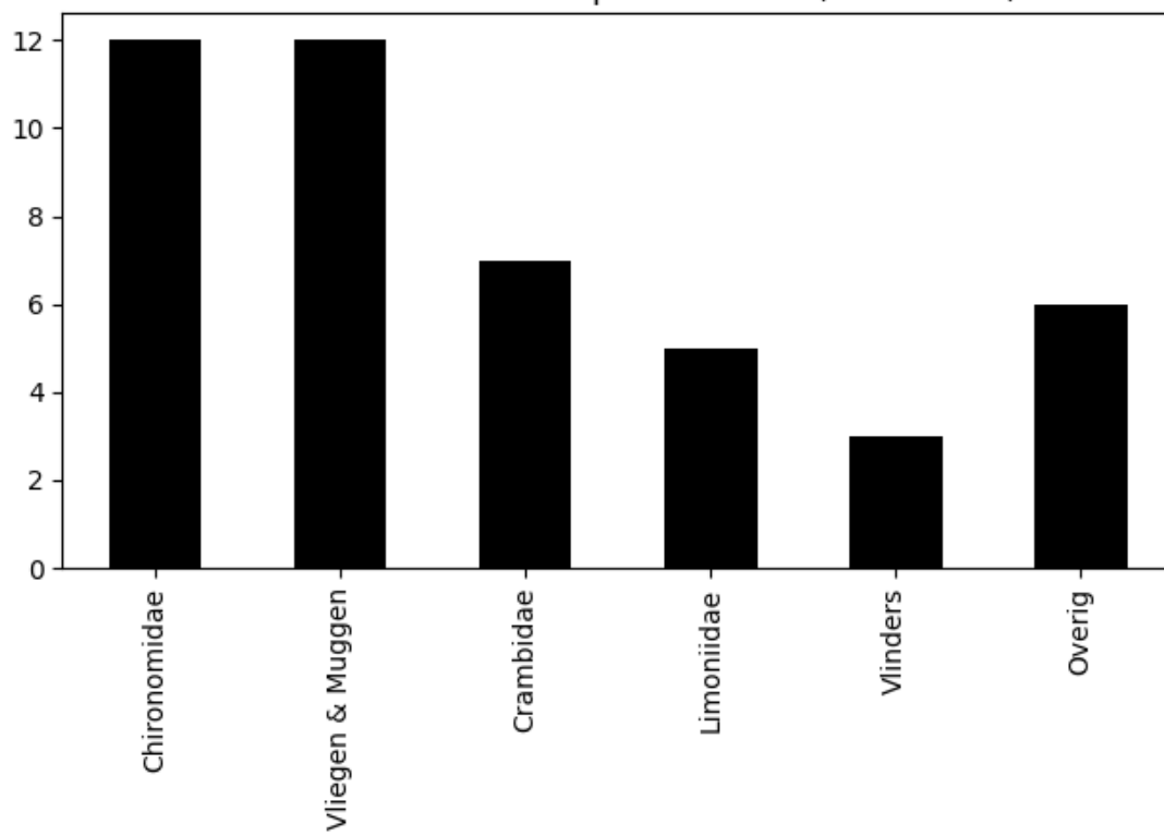
Voorkomen van ordes op 2022-07-15 (totaal = 45)
