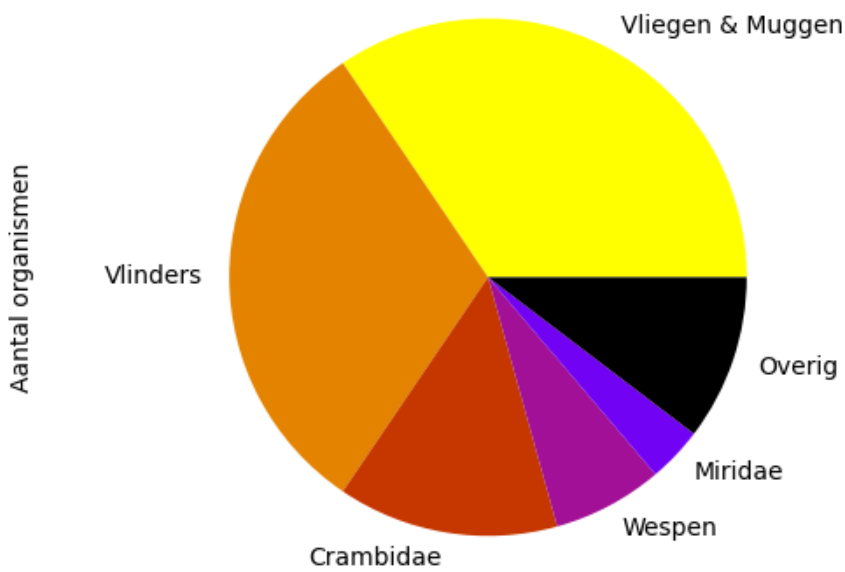
Voorkomen van ordes op 2022-07-28 (totaal = 29)
