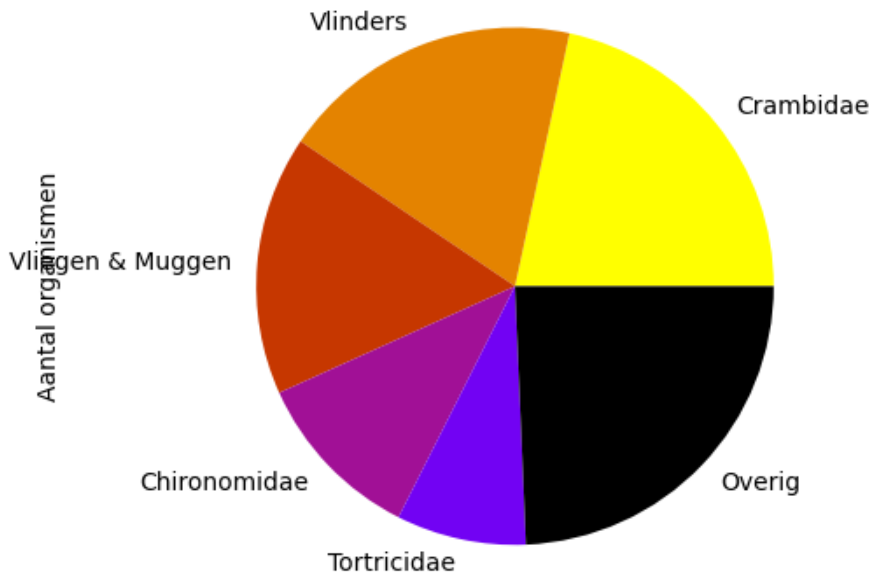
Voorkomen van ordes op 2022-07-09 (totaal = 37)
