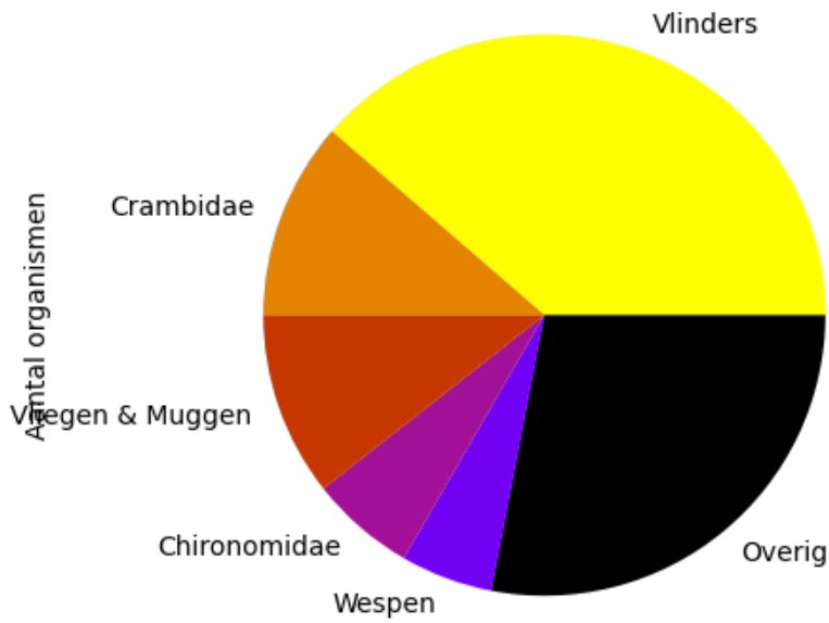
Voorkomen van ordes op 2022-06-24 (totaal = 132)
