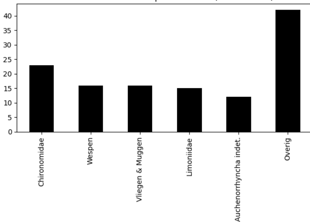
Voorkomen van ordes op 2022-07-12 (totaal = 124)
