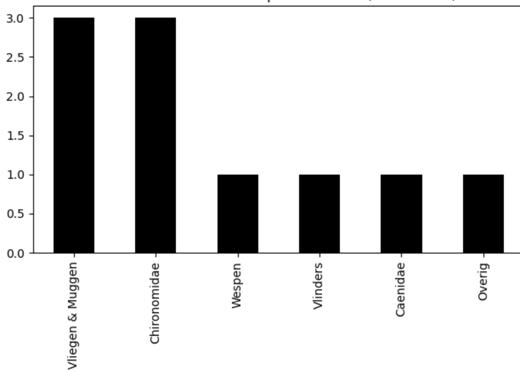
Voorkomen van ordes op 2022-06-28 (totaal = 10)
