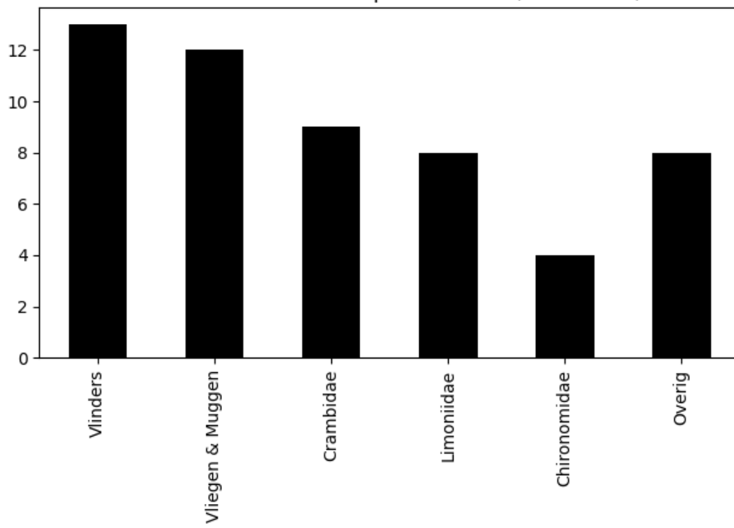
Voorkomen van ordes op 2022-07-29 (totaal = 54)
