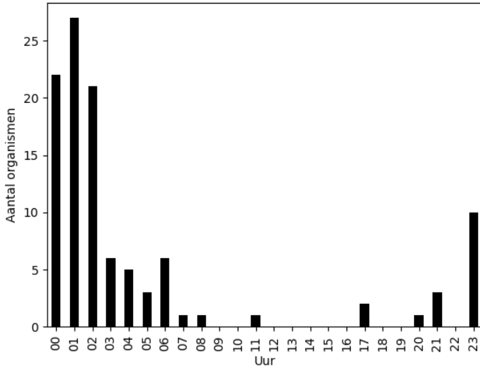
Aantal organismen per uur op 2022-07-18
