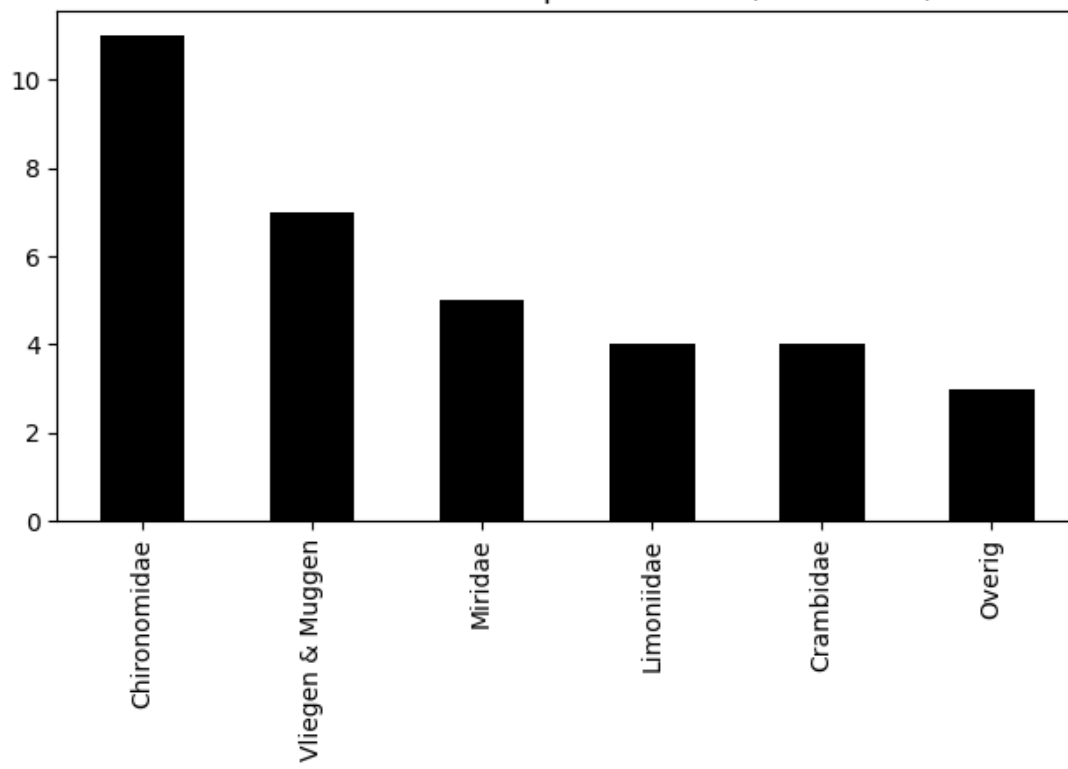
Voorkomen van ordes op 2022-06-30 (totaal = 34)
