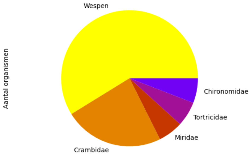
Voorkomen van ordes op 2022-07-01 (totaal = 17)
