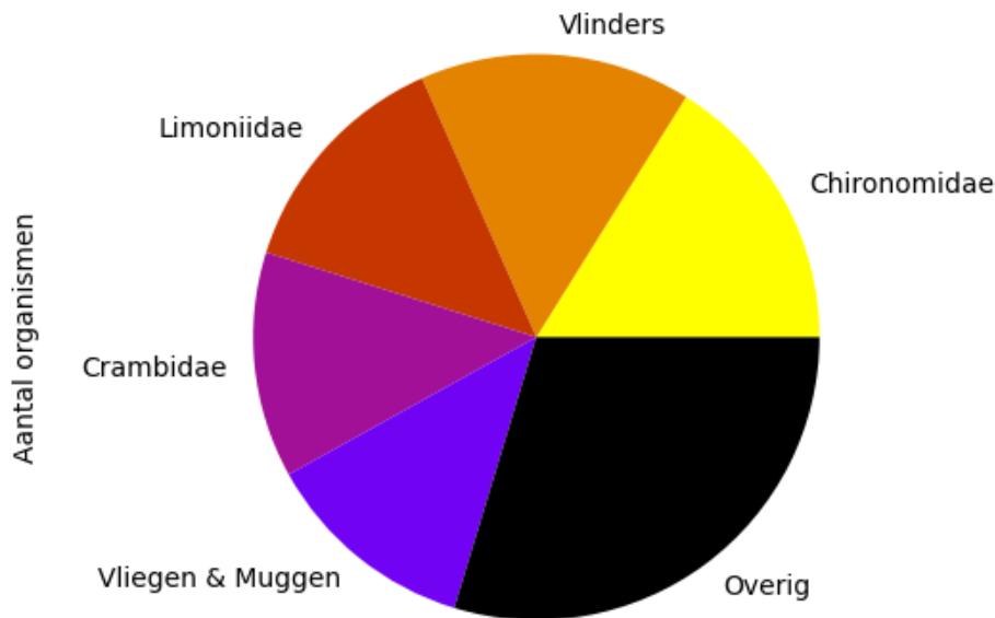
Voorkomen van ordes op 2022-07-19 (totaal = 155)
