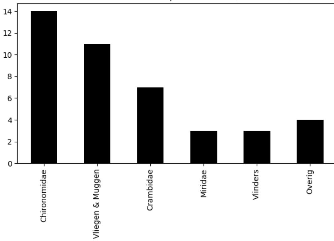
Voorkomen van ordes op 2022-07-17 (totaal = 42)
