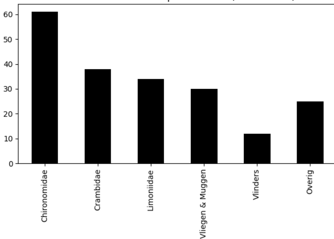
Voorkomen van ordes op 2022-07-05 (totaal = 200)
