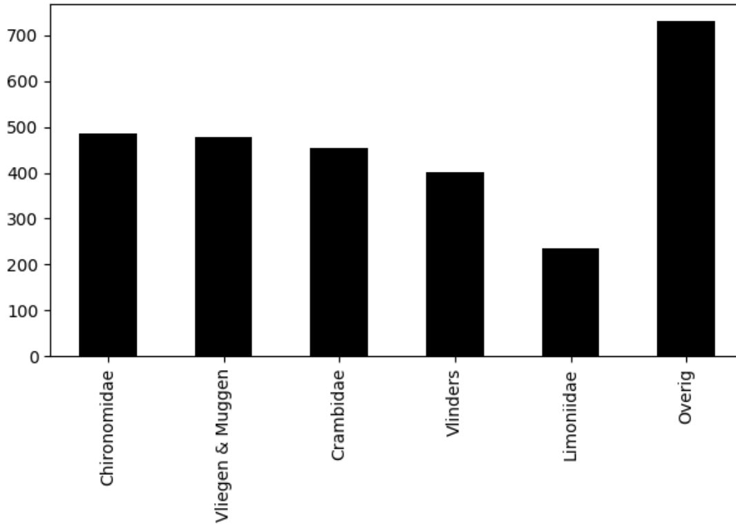
Voorkomen van ordes (totaal = 2786)
