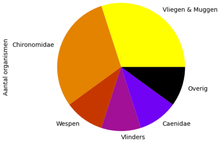
Voorkomen van ordes op 2022-06-28 (totaal = 10)
