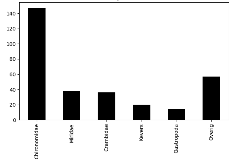
Voorkomen van ordes op 2023-09-08 (totaal = 312)
