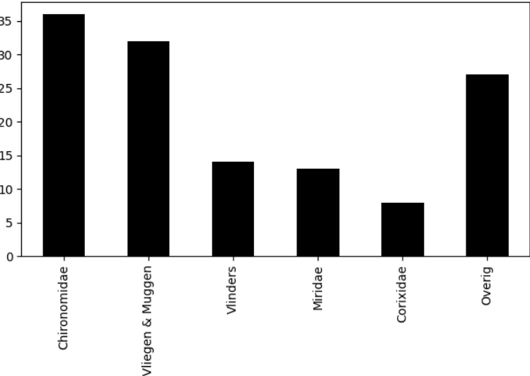
Voorkomen van ordes op 2023-09-27 (totaal = 130)
