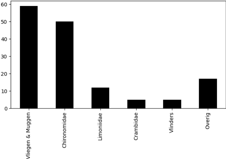
Voorkomen van ordes op 2023-08-27 (totaal = 148)
