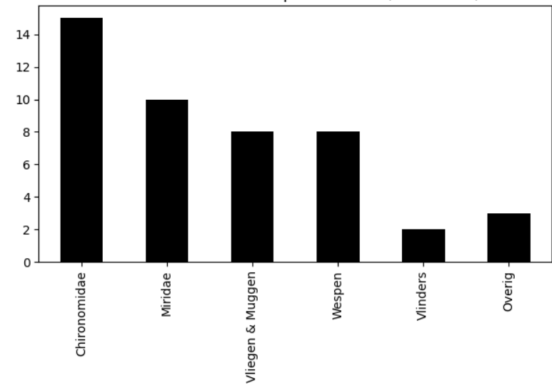
Voorkomen van ordes op 2023-09-15 (totaal = 46)
