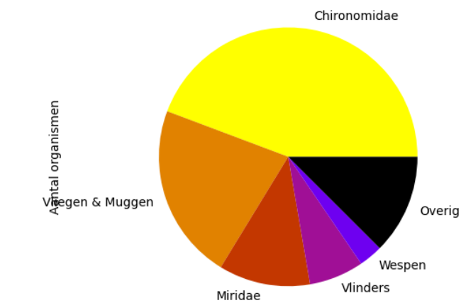
Voorkomen van ordes op 2023-09-17 (totaal = 673)
