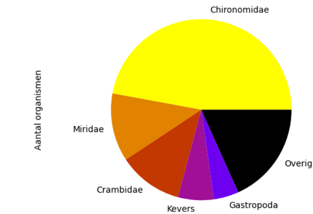
Voorkomen van ordes op 2023-09-08 (totaal = 312)
