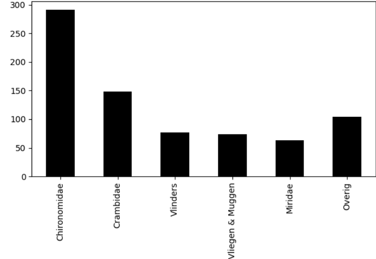
Voorkomen van ordes op 2023-08-21 (totaal = 757)
