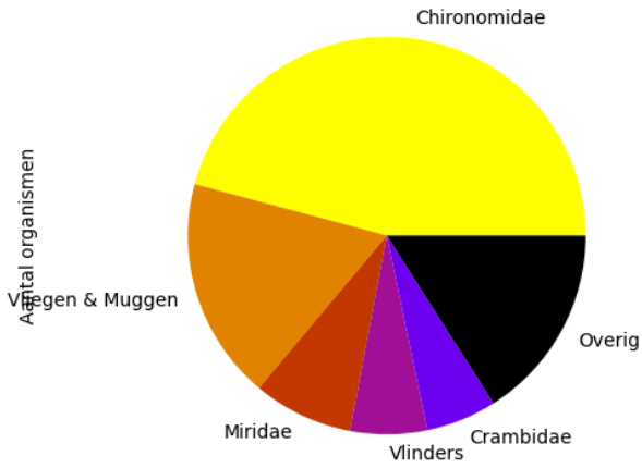
Voorkomen van ordes (totaal = 17041)
