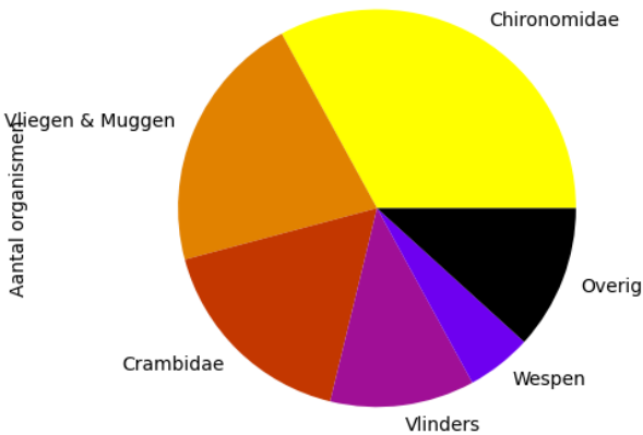
Voorkomen van ordes op 2023-08-29 (totaal = 264)
