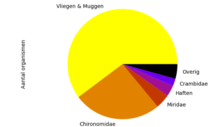
Voorkomen van ordes op 2023-09-25 (totaal = 93)
