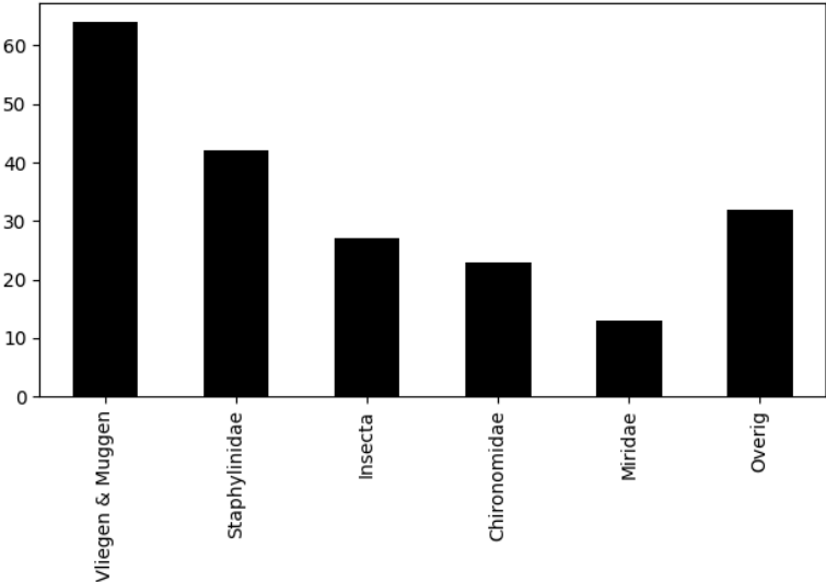
Voorkomen van ordes op 2023-08-11 (totaal = 201)
