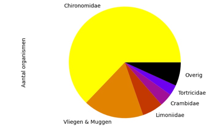
Voorkomen van ordes op 2023-08-31 (totaal = 132)
