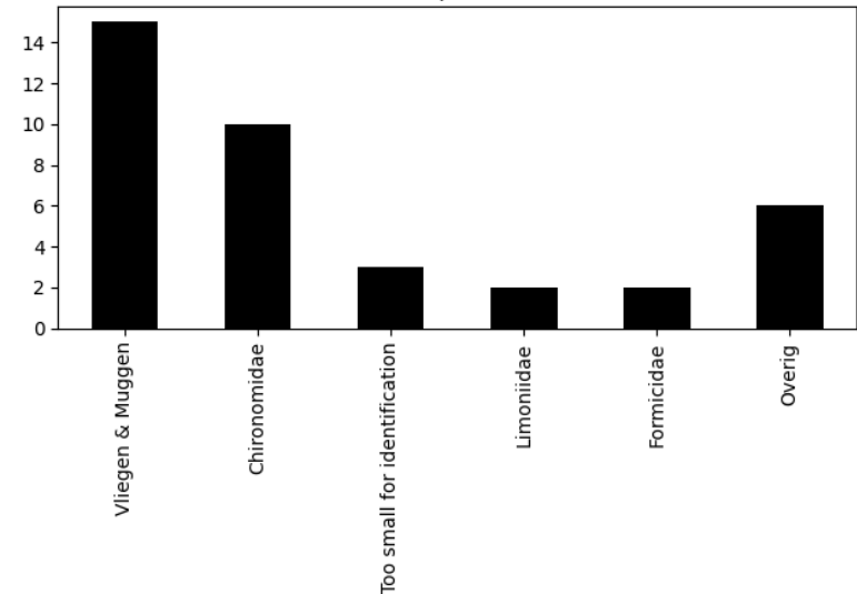
Voorkomen van ordes op 2023-09-30 (totaal = 38)
