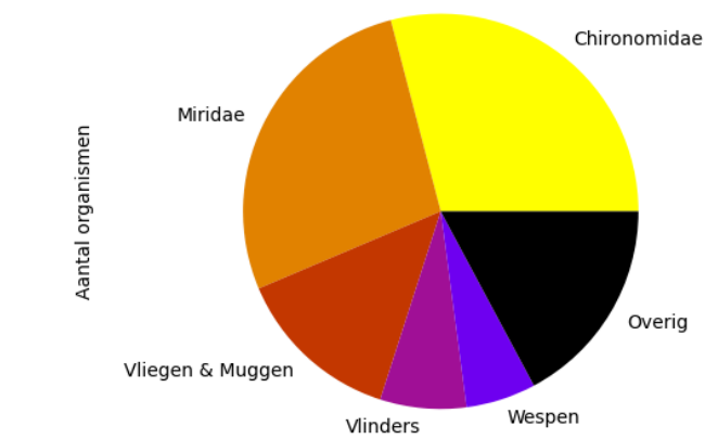
Voorkomen van ordes op 2023-10-02 (totaal = 227)
