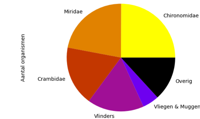
Voorkomen van ordes op 2023-09-05 (totaal = 385)
