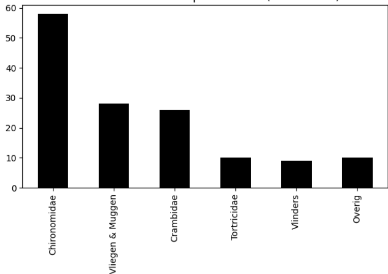
Voorkomen van ordes op 2023-08-25 (totaal = 141)
