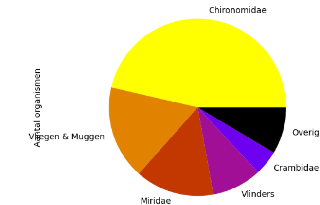
Voorkomen van ordes op 2023-08-17 (totaal = 375)
