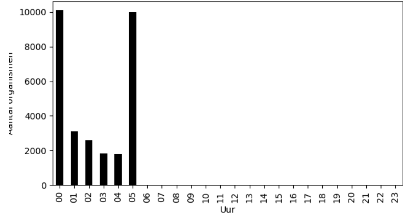
Aantal organismen per uur op 2023-04-21
