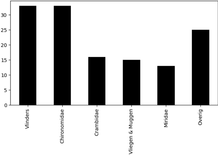
Voorkomen van ordes op 2023-09-14 (totaal = 135)
