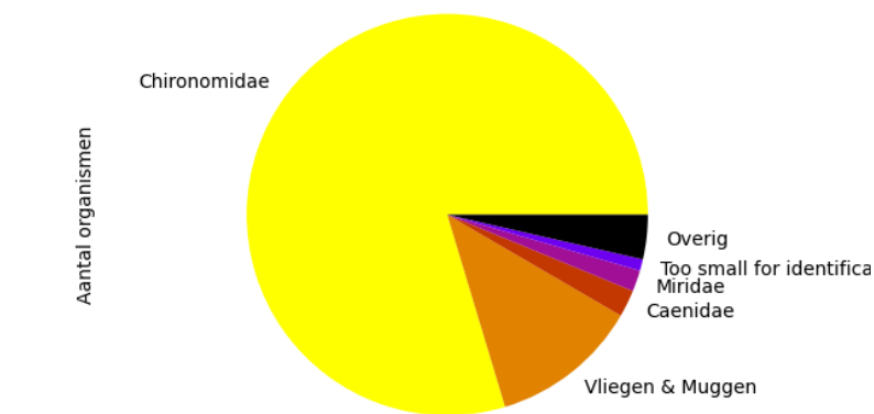
Voorkomen van ordes op 2023-07-16 (totaal = 644)
