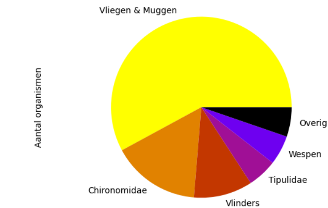
Voorkomen van ordes op 2023-09-24 (totaal = 19)
