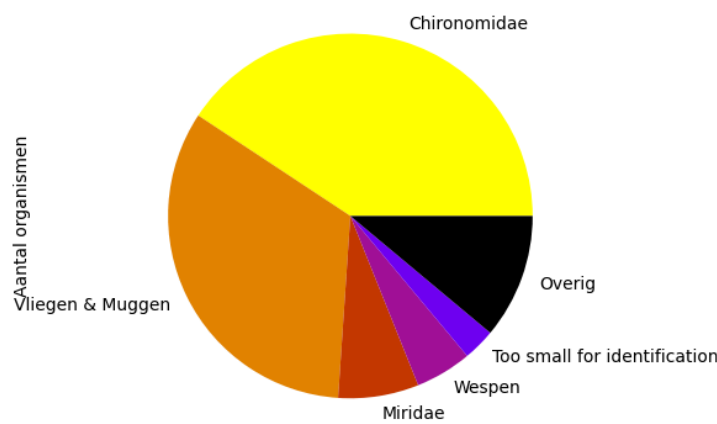
Voorkomen van ordes op 2023-09-11 (totaal = 280)
