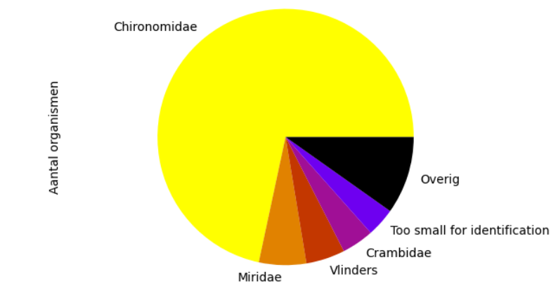
Voorkomen van ordes op 2023-09-06 (totaal = 469)
