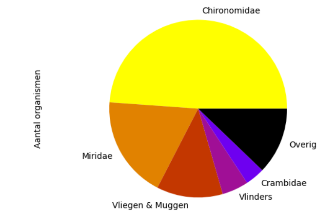
Voorkomen van ordes op 2023-09-10 (totaal = 706)
