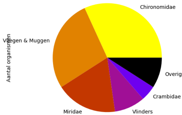
Voorkomen van ordes op 2023-09-22 (totaal = 22)
