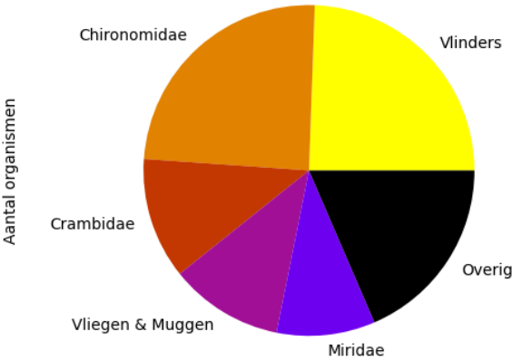
Voorkomen van ordes op 2023-09-14 (totaal = 135)
