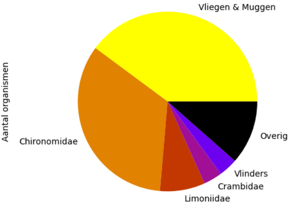
Voorkomen van ordes op 2023-08-27 (totaal = 148)
