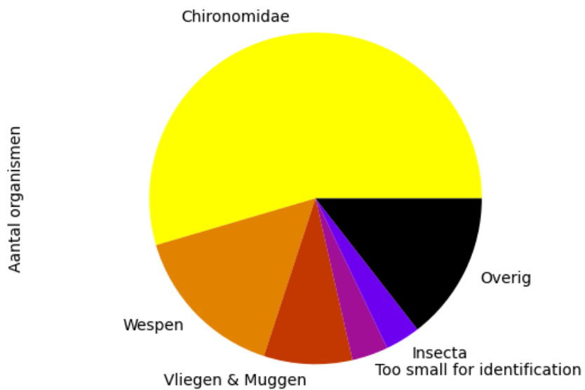
Voorkomen van ordes (totaal = 966)
