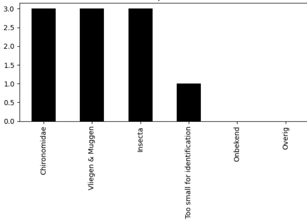
Voorkomen van ordes op 2023-09-19 (totaal = 10)
