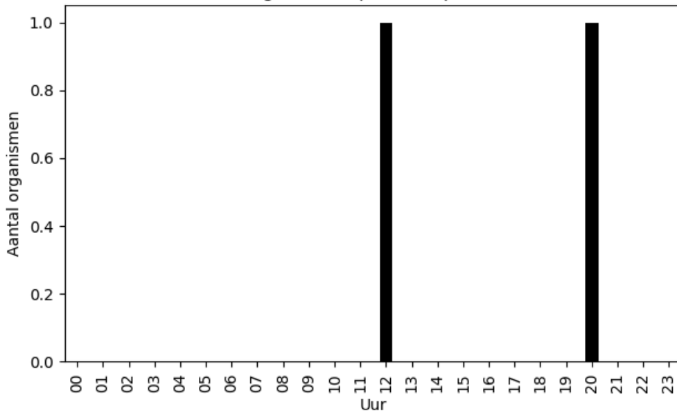
Aantal organismen per uur op 2023-08-15
