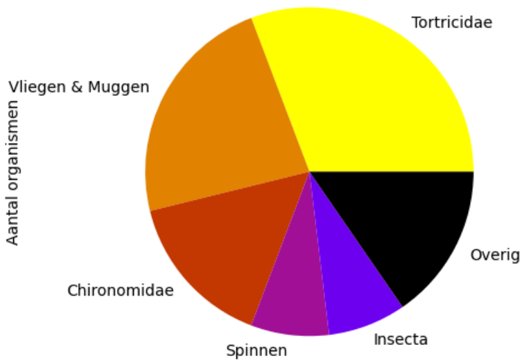
Voorkomen van ordes op 2023-09-03 (totaal = 13)
