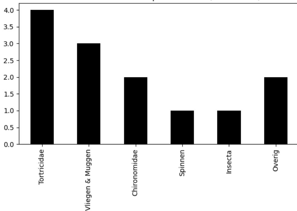
Voorkomen van ordes op 2023-09-03 (totaal = 13)
