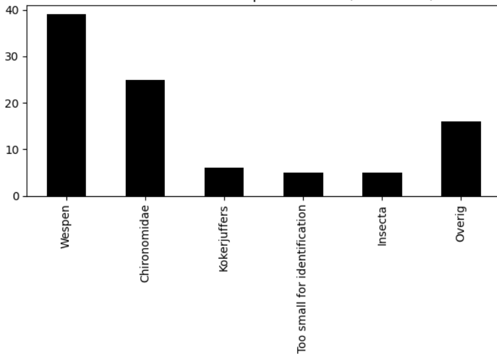
Voorkomen van ordes op 2023-09-11 (totaal = 96)
