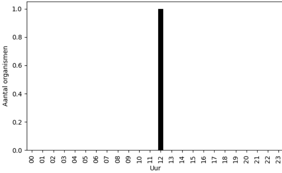
Aantal organismen per uur op 2023-08-23
