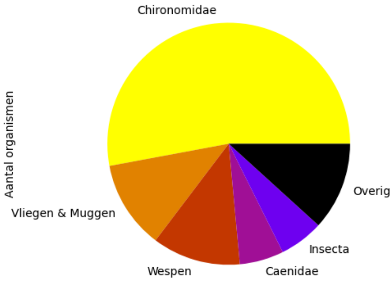
Voorkomen van ordes op 2023-08-07 (totaal = 17)
