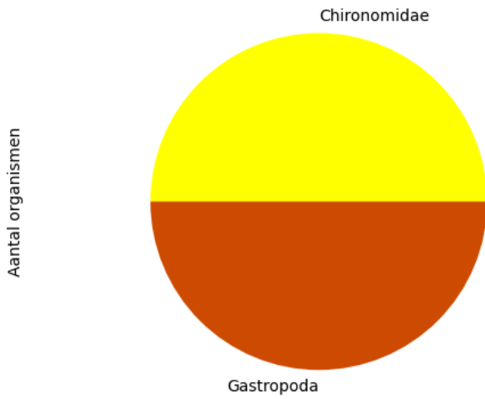
Voorkomen van ordes op 2023-08-15 (totaal = 2)
