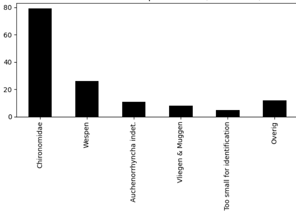
Voorkomen van ordes op 2023-09-09 (totaal = 141)
