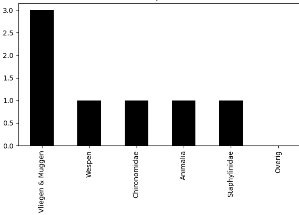
Voorkomen van ordes op 2023-08-31 (totaal = 7)
