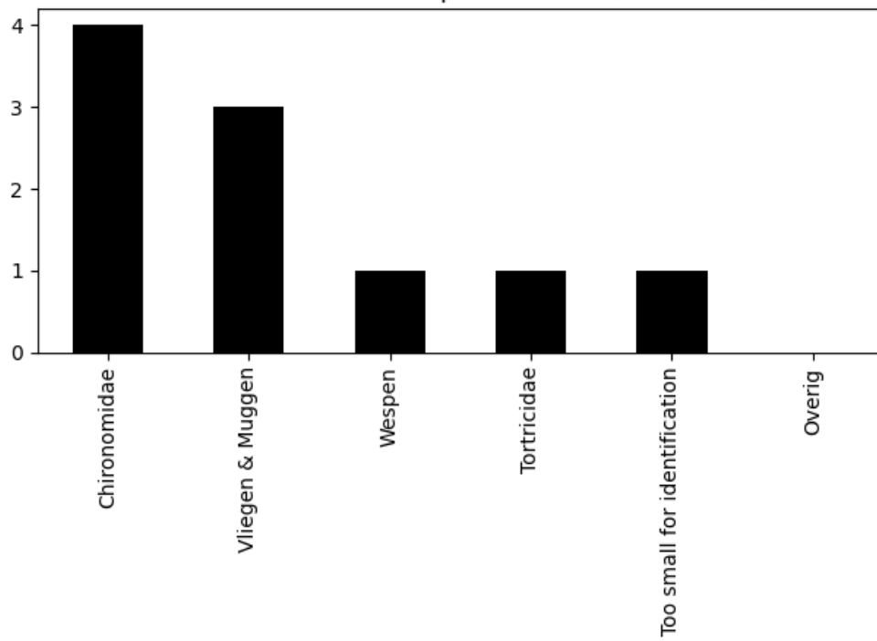
Voorkomen van ordes op 2023-09-13 (totaal = 10)
