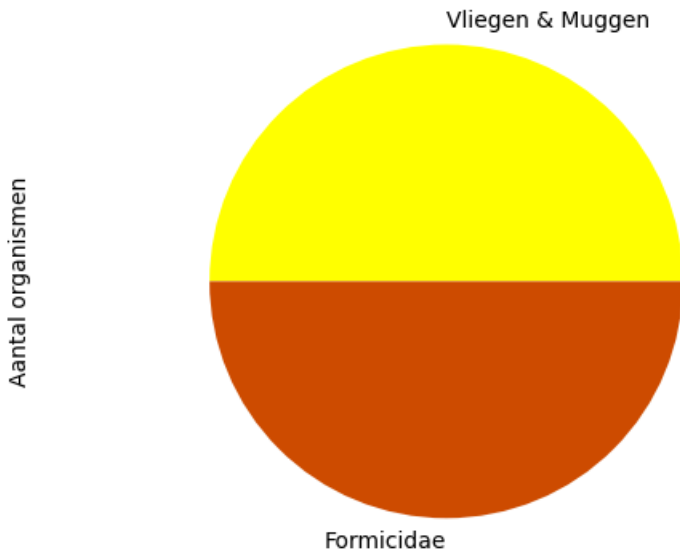
Voorkomen van ordes op 2023-08-29 (totaal = 2)
