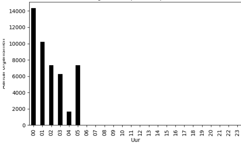
Aantal organismen per uur op 2023-05-09
