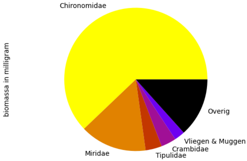
Verdeling biomassa per orde (totaal = 9 gram)
